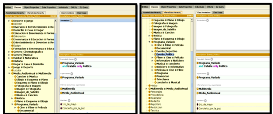
Razonador FaCT++
