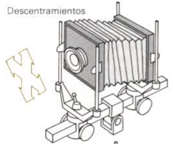
Basculamiento vertical
