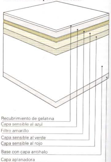
Estructura de la película en color
