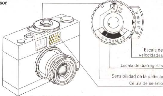
Exposímetro de selenio no acoplado
