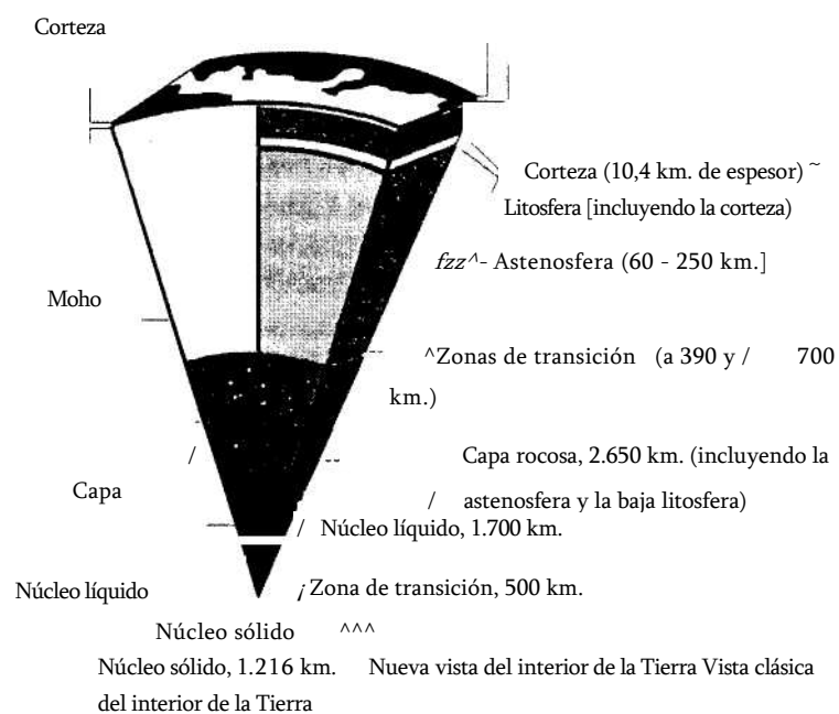
Figura 6. Nueva vista del interior de la Tierra
