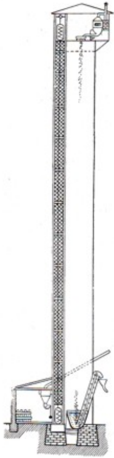
Figura 59. Torre perdigonera de una fábrica de municiones
