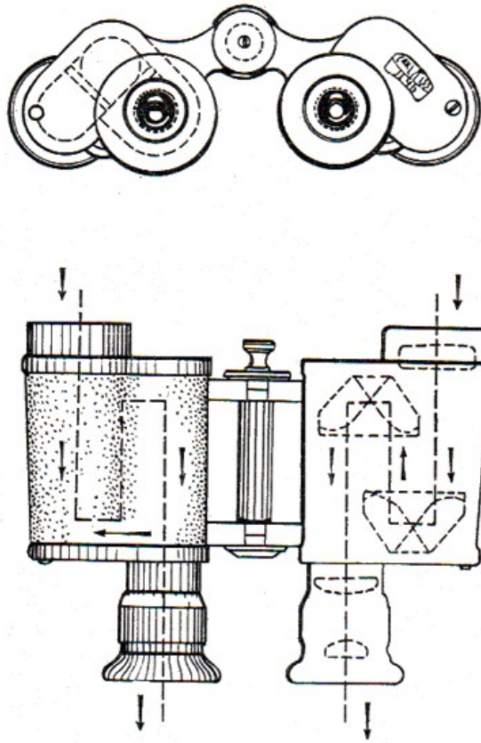
Figura 132. Prismáticos
