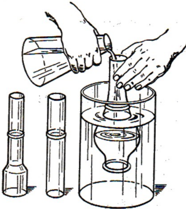
Figura 54. La presión del líquido sobre el fondo de la vasija depende exclusivamente del área de su base y de la altura a que se encuentra el nivel del líquido. En la figura se muestra un procedimiento para comprobar esta regla.
