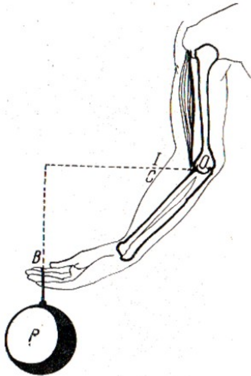
Fig. 27. El antebrazo C del hombre es una palanca de segundo género. La fuerza que actúa se aplica en el punto I; el apoyo de la palanca se encuentra en el punto O de la articulación; la resistencia que se vence (la pesa P) está aplicada en el punto B. La distancia BO es, aproximadamente, 8 veces mayor que la IO.
