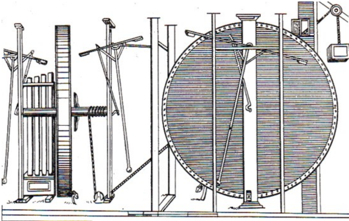
Figura 49. Rueda automotora de Orfirius, que estuvo a punto de ser adquirida por Pedro I (reproducción de un antiguo dibujo).
