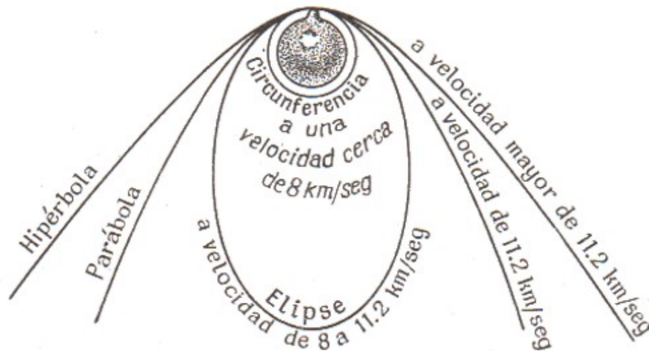
Figura 26. Trayectoria del proyectil disparado con una velocidad inicial de 8 km/seg y con velocidades mayores.
