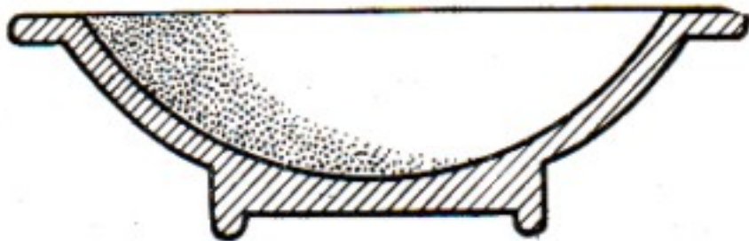
Figura 114. Vasija para hacer lentes de hielo.
