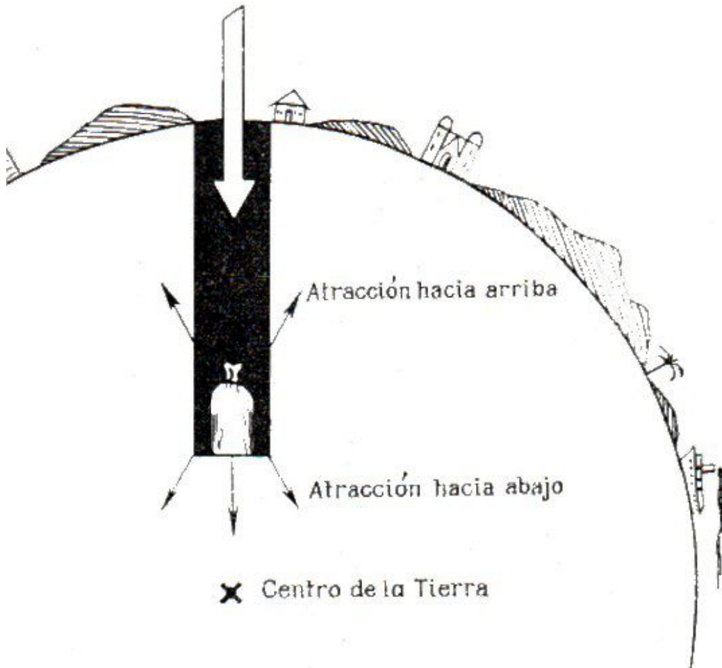
Figura 23. Explicación de por qué al ir penetrando en la Tierra disminuye la gravedad.
