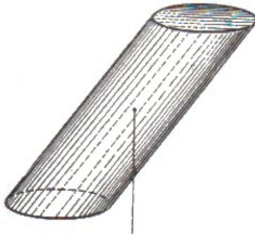
Figura 14. Este cilindro debe volcarse, puesto que la vertical de su centro de gravedad no pasa por la base.
