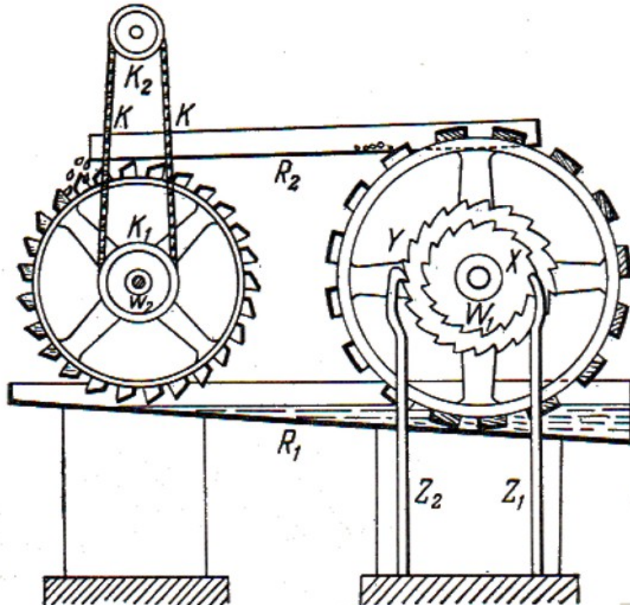
Figura 77. Mecanismo de un reloj que se da cuerda a sí mismo
