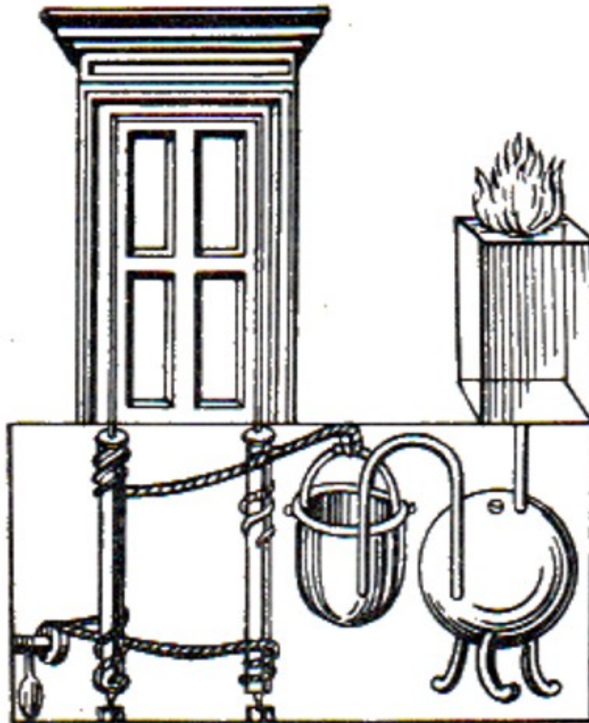
Figura 75. Esquema del mecanismo de las puertas del templo, que se abrían solas cuando ardía el fuego en el altar
