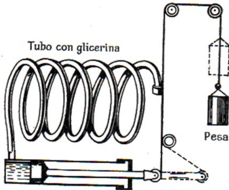
Figura 78. Esquema del mecanismo de un reloj automático de otro tipo.
