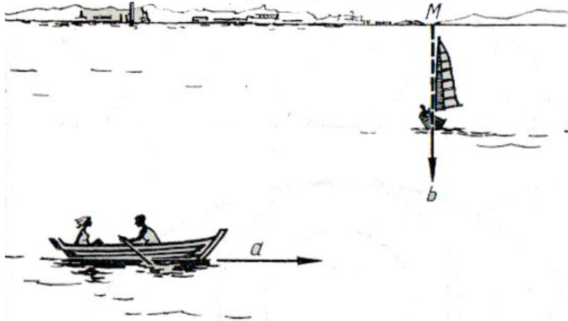
Figura 11. La barca de vela navega perpendicularmente a la dirección de la de remos. Las flechas a y b indican las velocidades respectivas. ¿Qué ven los pasajeros de la barca de remos?
