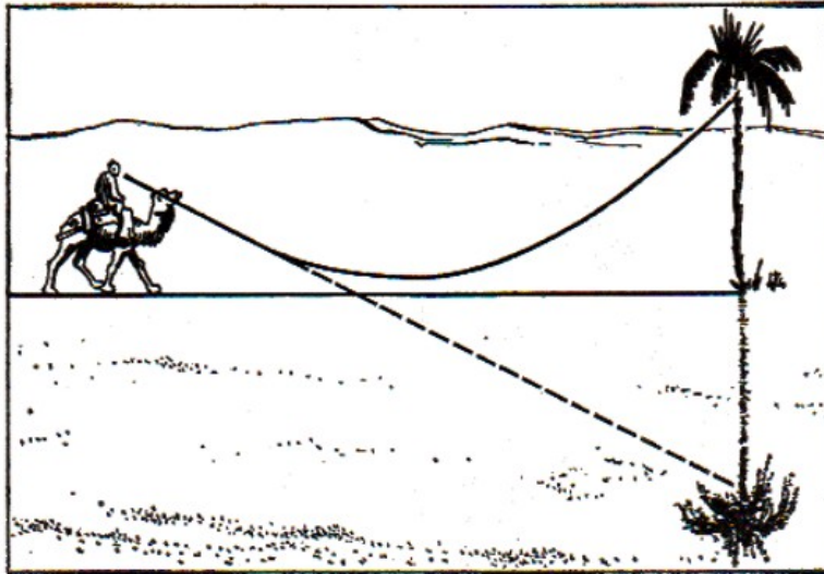
Figura 115. ¿Cómo se produce el espejismo en el desierto? Este dibujo, que generalmente reproducen los libros de texto, representa el camino que sigue un rayo de luz, cuyo ángulo de inclinación con respecto a la tierra está muy aumentado.
