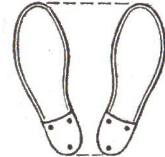
Figura 16. Cuando una persona está en pie, la vertical de su centro de gravedad pasa por la superficie limitada por las plantas de sus pies.
