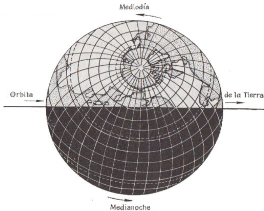
Figura 6. En el hemisferio de la Tierra en que es de noche, la gente se mueve más deprisa alrededor del Sol que en el que es de día.
