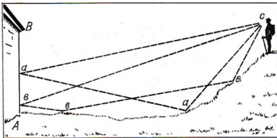
Fig. 150. Aquí el eco es muy claro.
