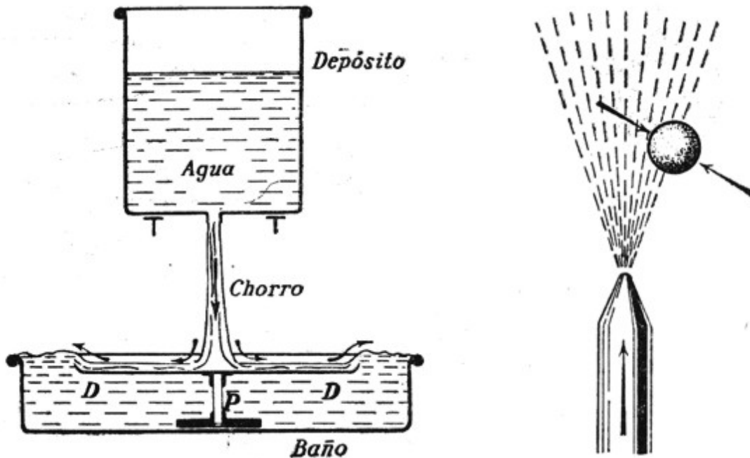
Figura 74 (izquierda). El disco DD sube por la barra P cuando sobre él se proyecta el chorro de agua del depósito. Figura 75 (derecha). El chorro de aire no deja que se caiga la pelotita.
