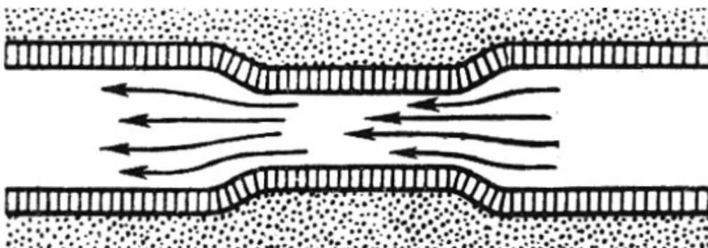
Figura 69. En las partes estrechas del canal el agua fluye más de prisa y presiona menos sobre las paredes que en las partes anchas.
