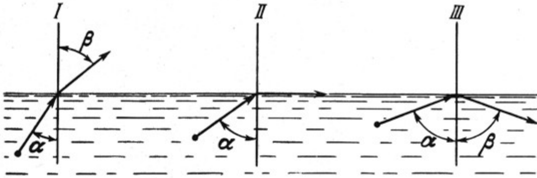
Figura 118. Varios casos de refracción de un rayo al pasar desde el agua al aire. En el II caso el rayo incide formando el ángulo límite con la perpendicular de incidencia y sale del agua rasando su superficie. El III caso representa la reflexión total.
