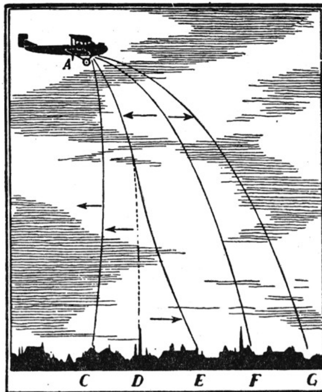
Figura 4. Trayectorias que siguen las bombas lanzadas desde un avión: AF, cuando no hace viento; AG, con viento favorable (de cola); AD, AC, con viento contrario (de proa); EA, con viento contrario arriba y favorable abajo
