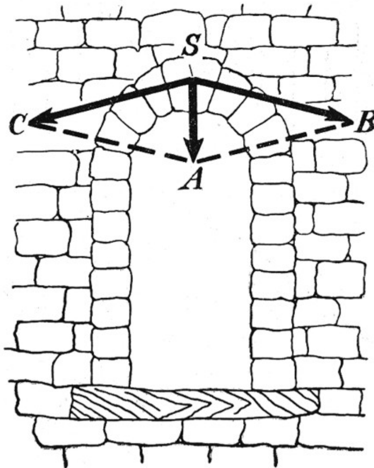
Figura 18. Explicación de por qué son tan resistentes los arcos.
