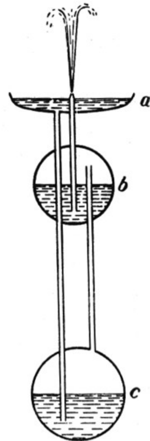
Figura 63. La fuente de Herón clásica.
