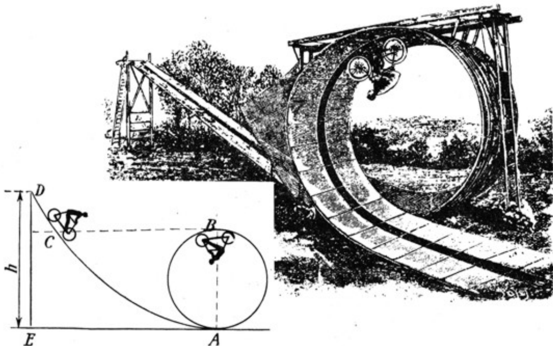
Figura 44. El "rizo de la muerte". Abajo a la izquierda el esquema para el cálculo.
