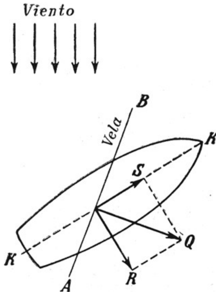
Figura 20. Así se puede navegar a vela en contra del viento.
