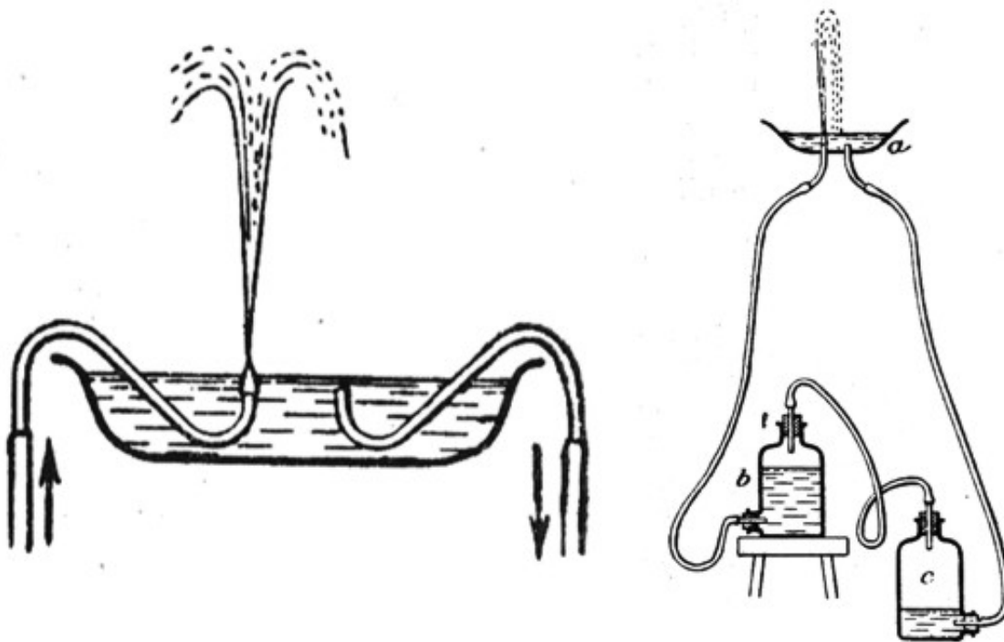
Figura 64. Modificación actual de la fuente de Herón. Izquierda una variante que evita horadar el fondo del plato superior.
