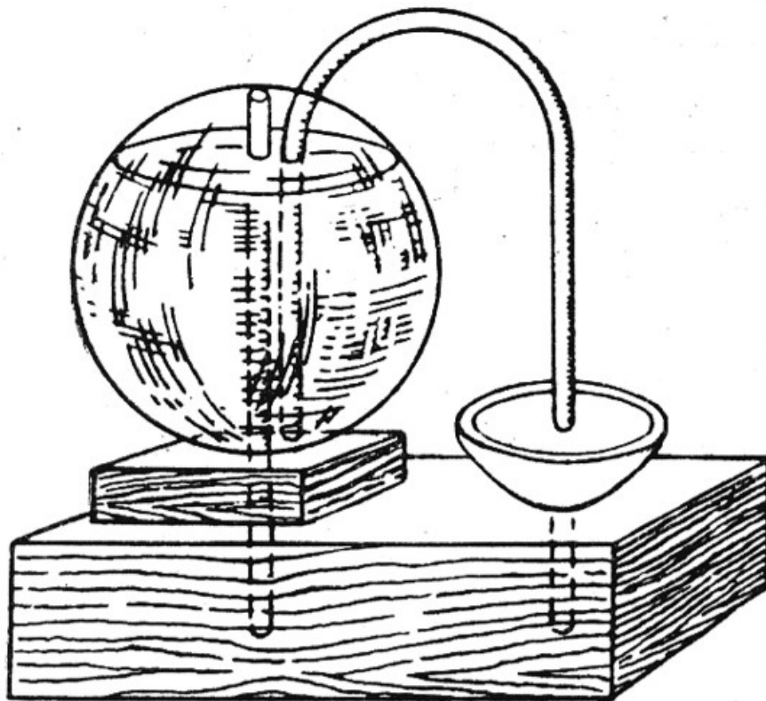
Figura 85. Termoscopio de Herón.
