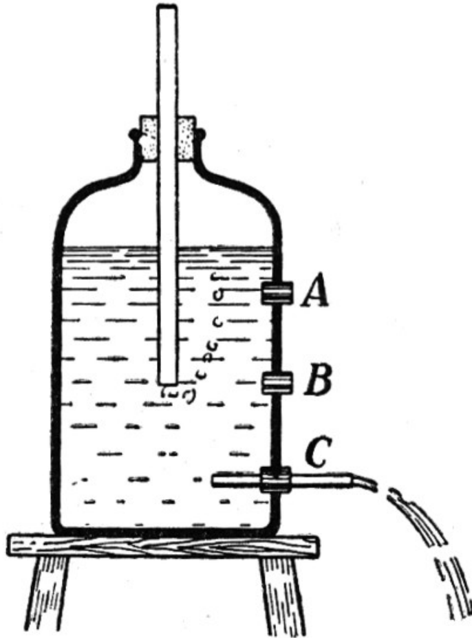
Figura 60. Esquema del frasco de Mariotte. El agua sale del orificio uniformemente.
