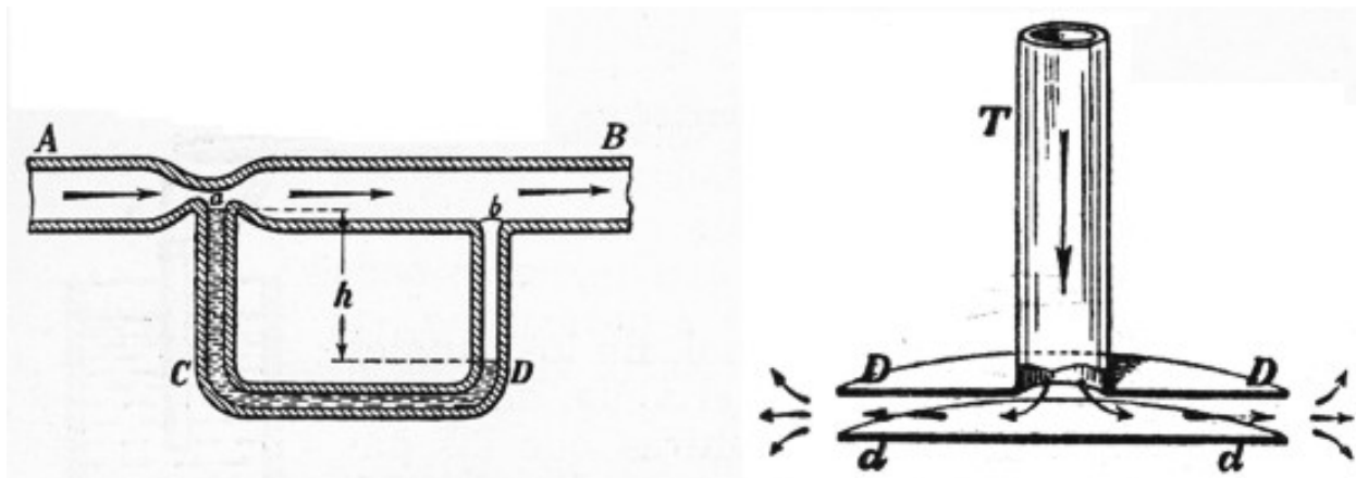
Figura 72 (izquierda). Ilustración del teorema de Bernoulli. En la parte más estrecha (a) del tubo AB la presión es menor que en la más ancha (b). Figura 73 (derecha). Experimento con discos
