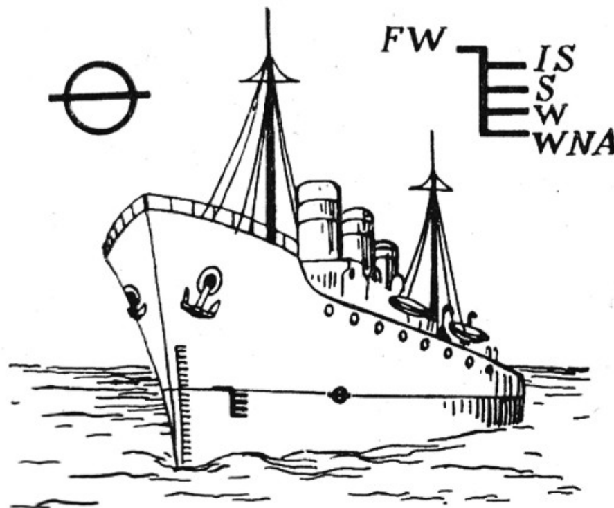
Figura 52. Disco de carga máxima en el costado de un buque. Las marcas se hacen al nivel de la línea de flotación. Para que se vean mejor se muestran aparte aumentadas. El significado de las letras se explica en el texto.
