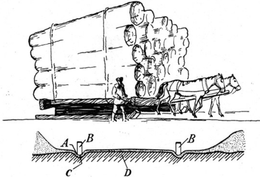
Figura 23. Arriba, un trineo cargado sobre un camino de hielo; dos caballos arrastran una carga de 70 toneladas. Abajo, el camino de hielo; A, carril; B, deslizaderas del trineo; C, nieve apisonada; D, fundamento de tierra de la carretera.
