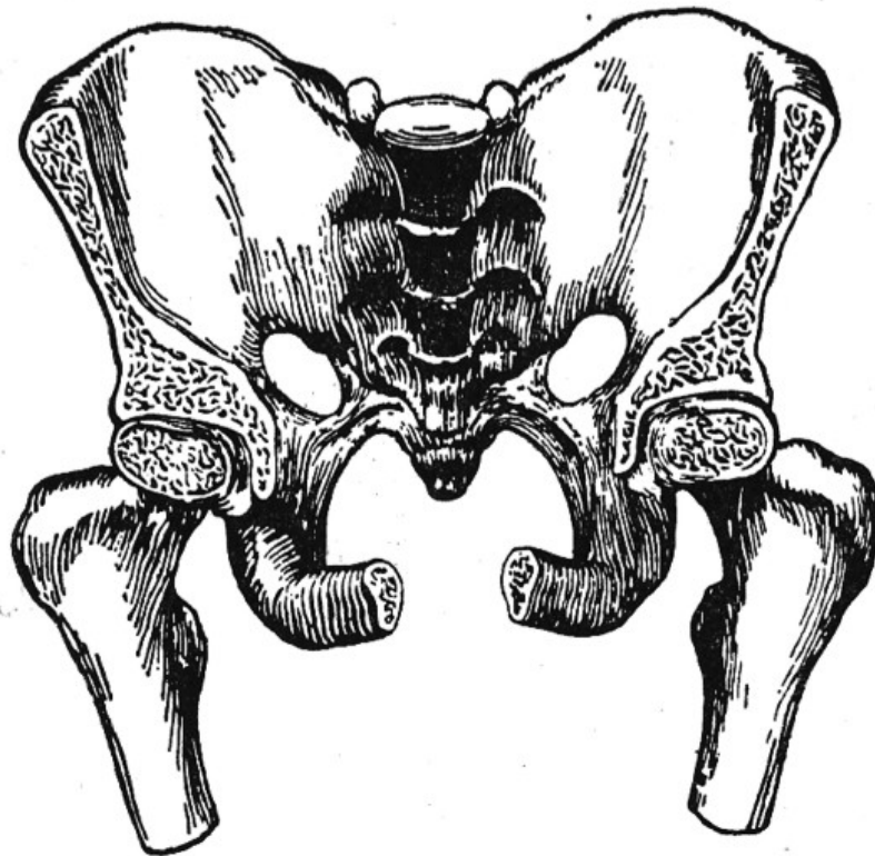
Figura 62. Los huesos de nuestras articulaciones coxofemorales no se separan debido a la presión atmosférica, que los sujeta lo mismo que a los hemisferios de Magdeburgo.
