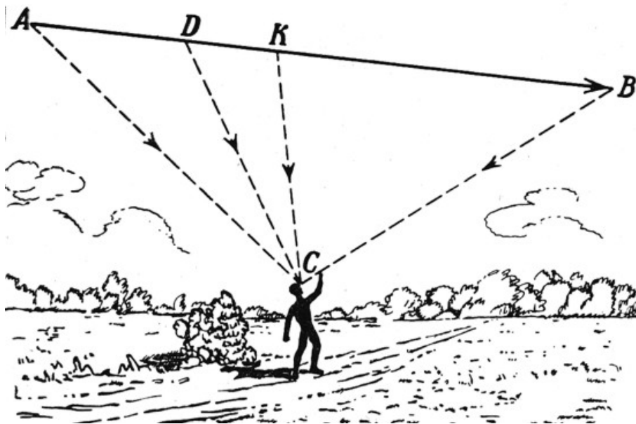
Figura 154. Explosión ilusoria de un bolido.
