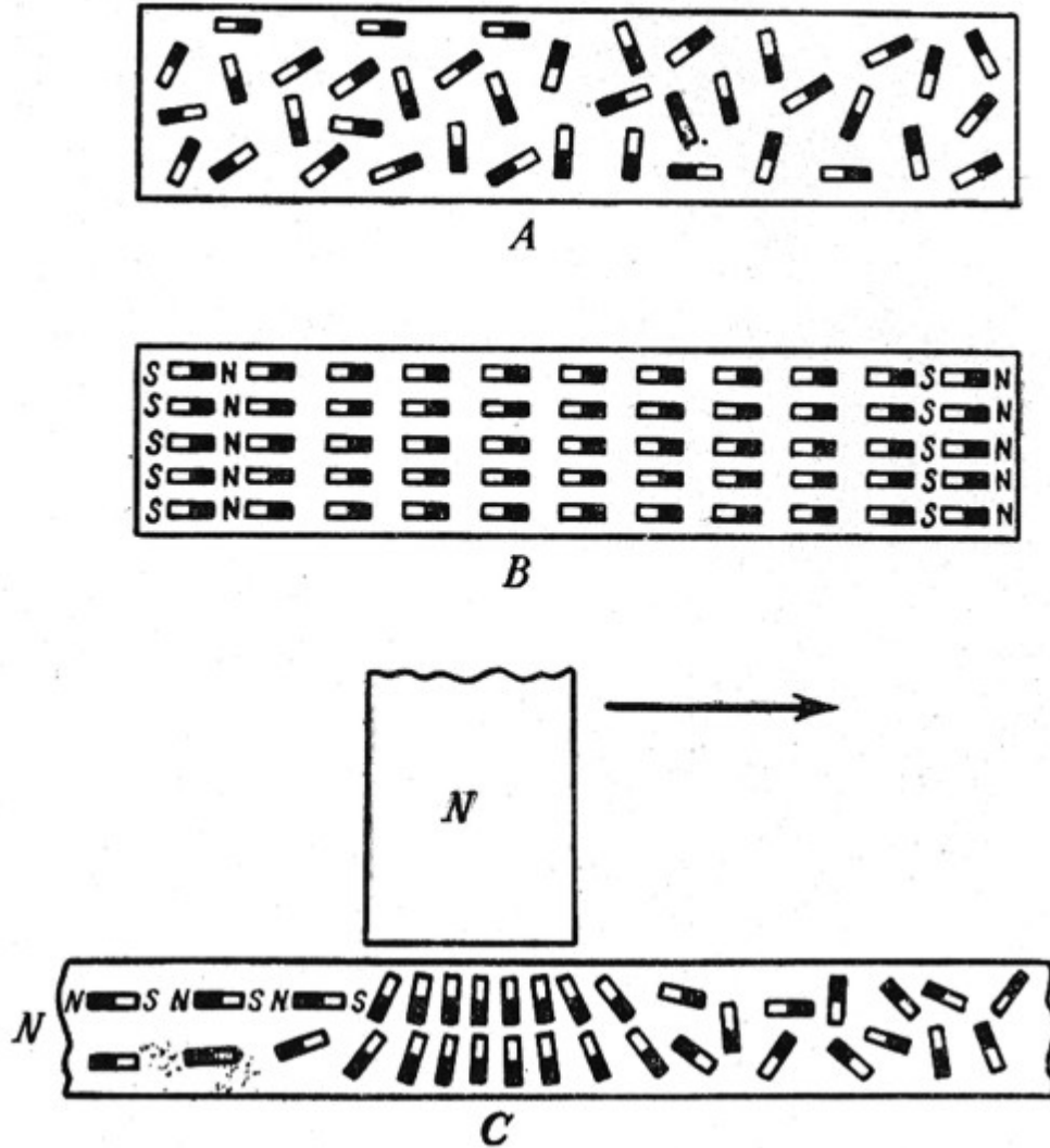
Figura 93. A, disposición de los imanes elementales en una barra no imanada; B, ídem en el acero imanado; C, acción del polo del imán sobre los imanes elementales del acero que se imanta.
