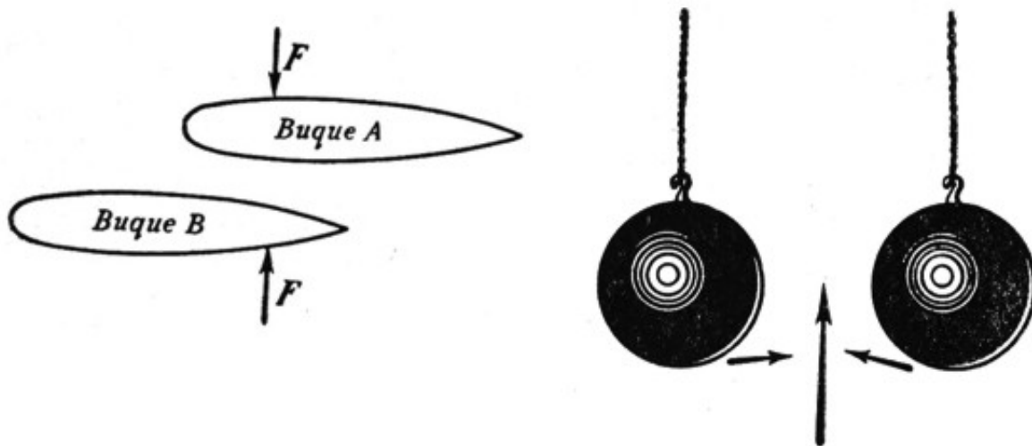
Figura 77 (izquierda). Cuando los barcos navegan hacia adelante, el B gira y pone proa hacia el A. Figura 78 (derecha). Si se sopla entre dos esferas ligeras se ve como se aproximan y hasta llegan a juntarse.
