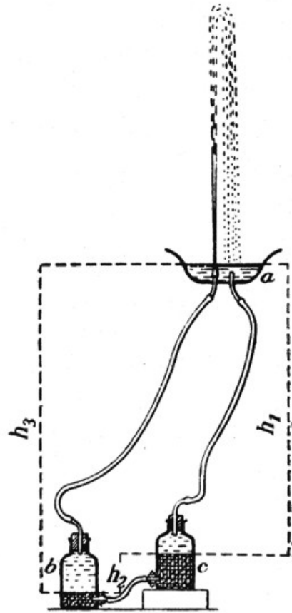
Figura 65. Fuente que funciona por la presión del mercurio. La altura a que sube el Chorro es diez veces mayor que la diferencia entre los niveles del mercurio.
