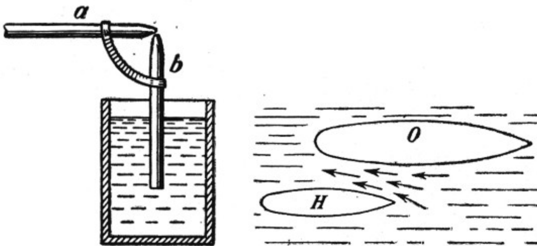
Figura 70 (izquierda). Esquema del pulverizador. Figura 71 (derecha). Corriente de agua entre dos buques que navegan juntos.
