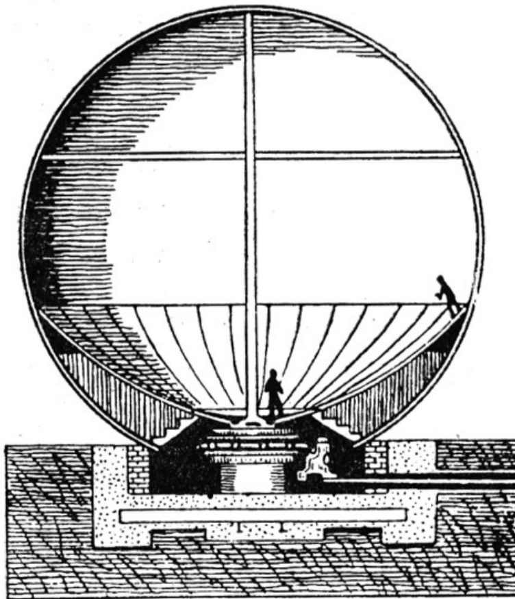
Figura 40. La esfera "encantada" (corte)
