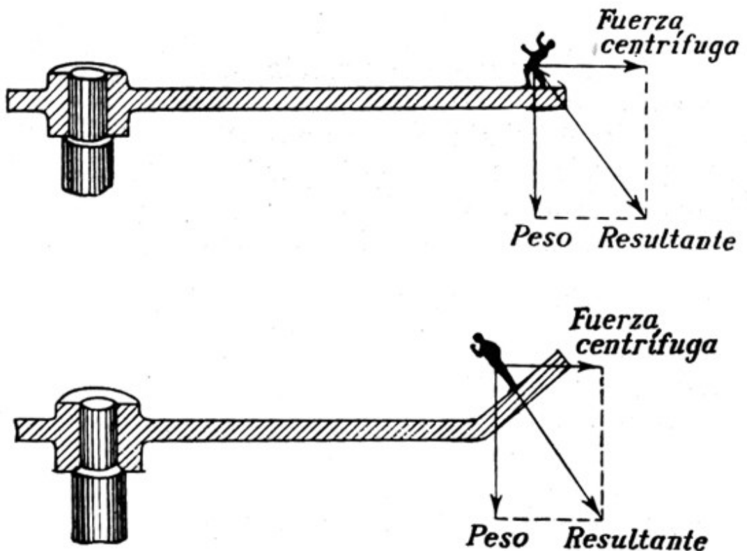
Figura 37 arriba. Fuerzas que actúan sobre una persona que se encuentra en el borde de una plataforma giratoria. Figura 38 abajo. Cuando la plataforma tiene el borde inclinado, la persona que se encuentra en él guarda el equilibrio perfectamente.
