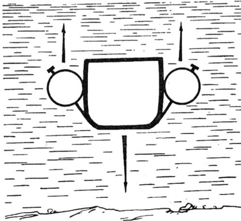
Figura 54. Esquema del salvamento del rompehielos "Sadko"; se muestra el corte del rompehielos, los flotadores y las bragas
