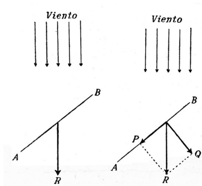
Figura 19. El viento siempre le empuja a la vela formando un ángulo recto con su plano.
