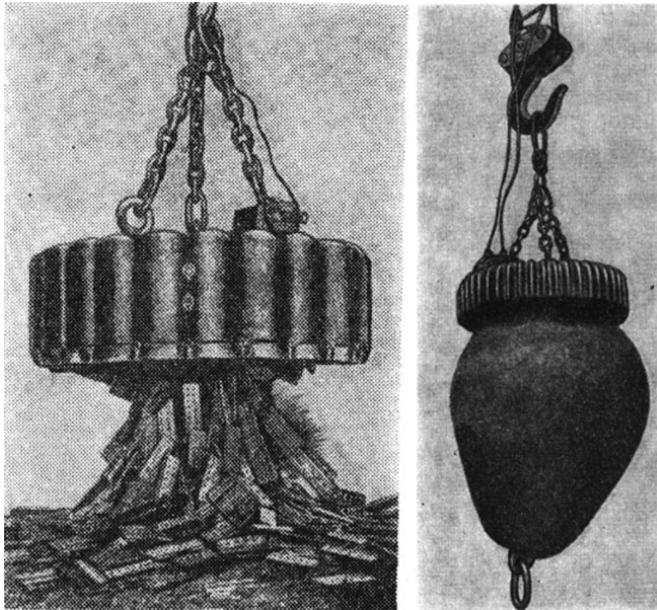
Figura 94 (izquierda). Una grúa de electroimán transportando planchas de hierro. Figura 95 (derecha). El electroimán de una grúa transportando un bloque de hierro de 6,5 t.
