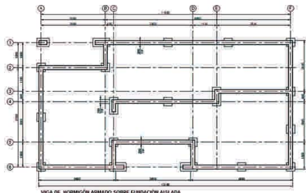
Figura 8 - 37: Plano de fundación aislada con viga de hormigón armado, donde se especifican los ejes que es necesario replantear para los cimientos aislados.
