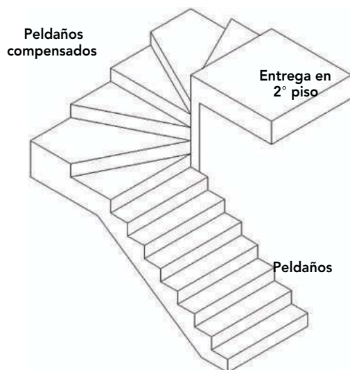
Figura 12 – 11: Isométrica de escalera de un tramo con peldaños compensados de media vuelta.
