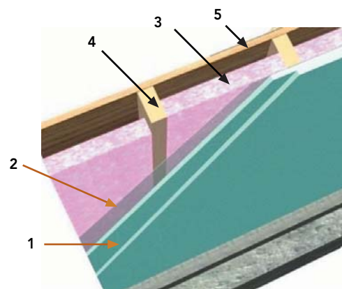
Figura 14-96: Vista de los componentes del paramento interior del tabique.
