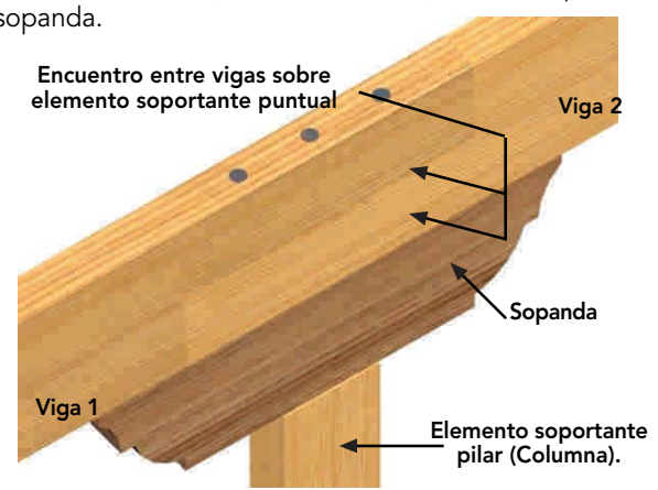
Figura 9 - 41: Utilización de sopanda como elemento de apoyo en encuentro entre vigas sobre elemento soportante puntual.
