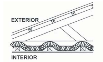
Figura 14 - 17b: Material aislante flexible en cielo horizontal.
