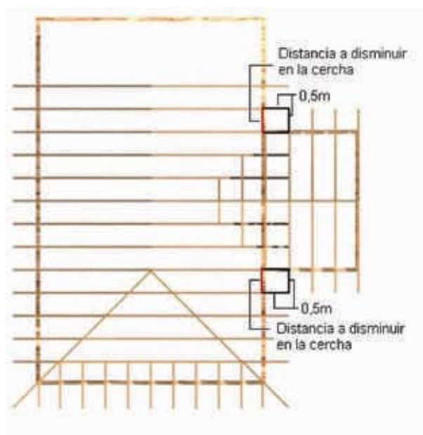
Figura II - 14: Determinación de la magnitud a disminuir en forma secuencial en cada cercha.
