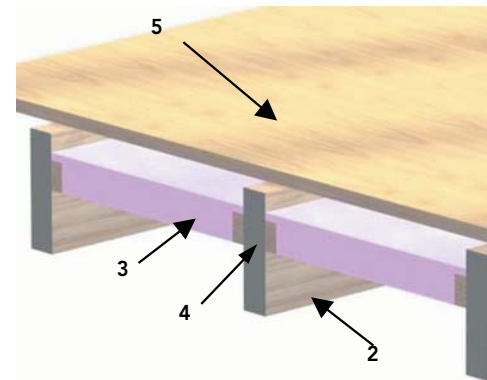
Figura 14 - 70: Colocación de aislación termo-acústica entre el listoneado de cielo sobre la plancha de yeso cartón, para luego colocar el tablero estructural, arriostando la estructura de plataforma del entepiso.
