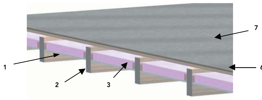
Figura 14 - 71: Vista general del entramado de entepiso, utilizando como terminación sobre el tablero de piso estructural, un pañete de lana de un espesor mínimo de 8 a 10 mm y alfombra de lana o draylón acrílico, de un espesor mínimo de 10mm.
