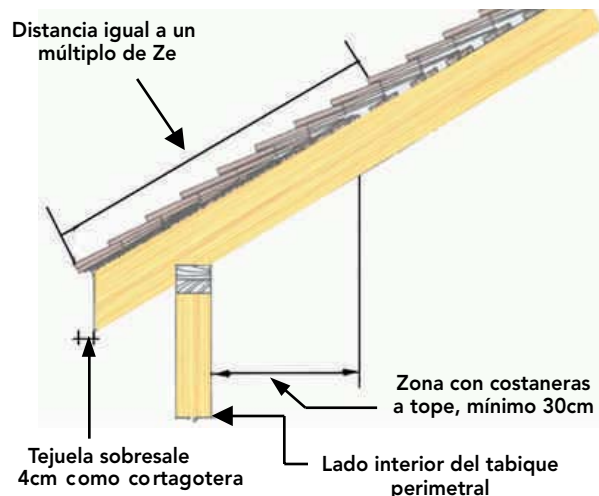
Figura 17-18: Corte que muestra las zonas y distancias mínimas de la techumbre a proteger de la humedad.
