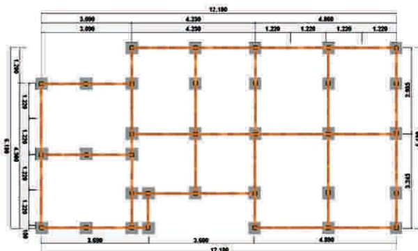
Figura 8 - 48 : Plano de vigas principales que amarran las cabezas de los pilotes, conformando el plano horizontal de la plataforma de madera.
