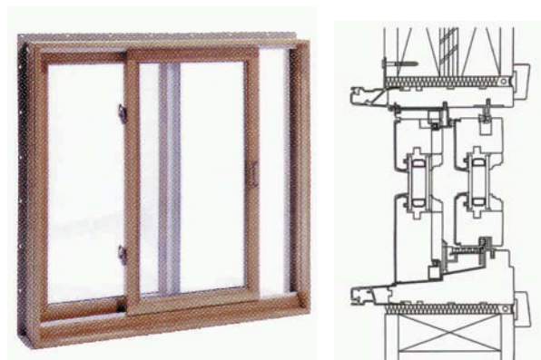
Figura 22 –25: Ventana de movimiento deslizante.
