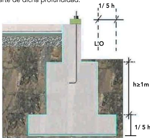
Figura 8 - 22: Situación de fundación con zapata que sobresale de la línea oficial (L.O = línea oficial).
