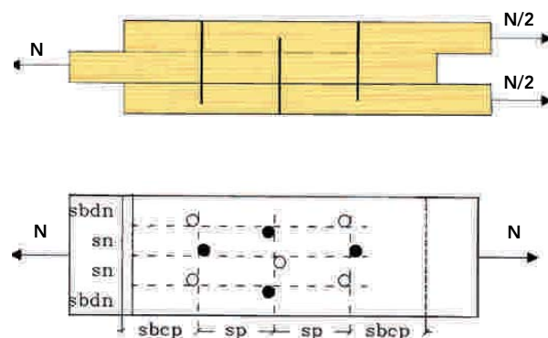
Figura 7- 21 : Disposición de clavado.
