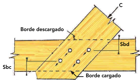
Figura 7 - 9 : Espaciamiento mínimo entre un elemento de unión y el borde vecino.
