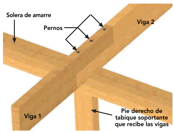
Figura 9 - 42: Empalme típico de dos vigas sobre un tabique estructural llamado ensamble en Entabladura , el cual consiste en ejecutar un corte tipo media madera y fijarlo con pernos, clavos, adhesivos o tarugos.
