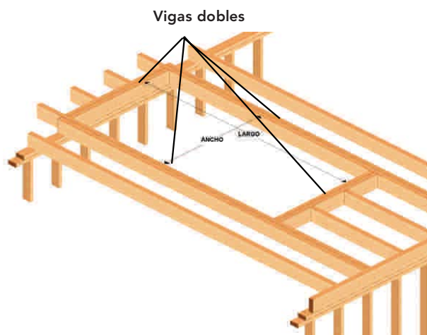
Figura 9 – 52 : Escotilla necesaria para pasada de escalera, se coloca doble viga como cabezal y refuerzos donde se apoyarán las otras vigas.
