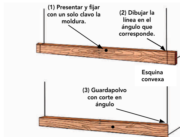
Figura 21-8: Secuencia para llegar a realizar el corte en 45° en la moldura.
