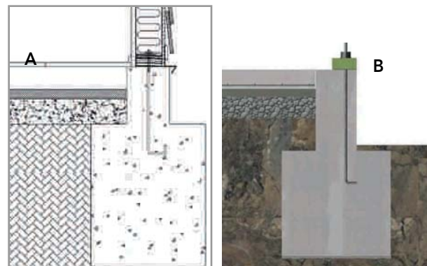
Figura 8 - 28: Figura A, representación técnica del corte de la fundación tipo, figura B, un corte de la fundación en terreno.
