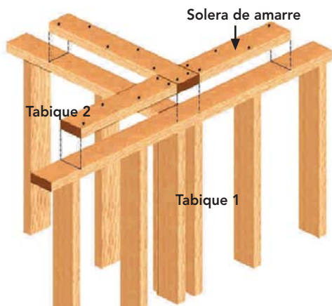
Figura 10 - 16: Solera de amarre o sobresolera que une un muro perimetral con un tabique interior.
