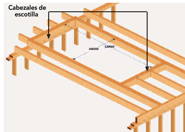
Figura 9 - 29: Cabezales que forman la escotilla con dos piezas de 2" x 8" (2 (2" x 8")) de la escalera que comunica el primer y el segundo piso.
