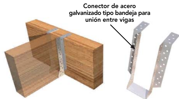
Figura 9 – 47: Conector de acero galvanizado, el cual incorpora perforaciones tanto triangulares como circulares, que permite resistir altas cargas cuando es fijado con clavos comunes.
