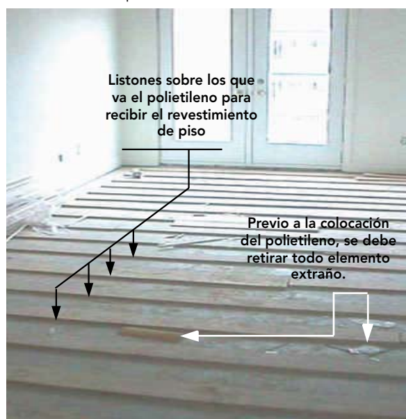
Figura 20 - 8: Disposición de los listones sobre plataforma de hormigón, donde irá el polietileno de espesor de 0,2 a 0,5 mm.
