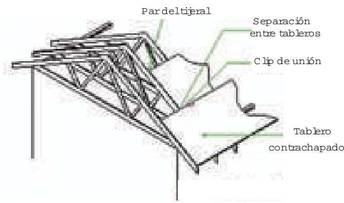
Figura 11-63: Los bordes extremos menores de los tableros deben apoyarse sobre los pares.
