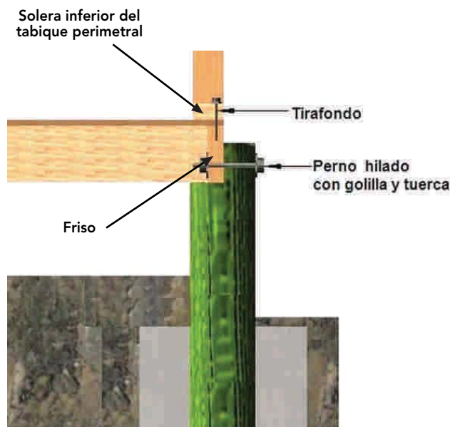
Figura 9 - 23: Corte intermedio de viga perimetral del entramado horizontal, se fija a cada pilote mediante perno hilado con golillas y tuerca, cuyas dimensiones las determina el cálculo. Normalmente son de un diámetro mínimo de 12 mm y largo de 7" a 8" (170 a 200 mm). Solera inferior del tabique perimetral se fija al friso mediante tirafondos cada 0,40 m, definidos según cálculo.
