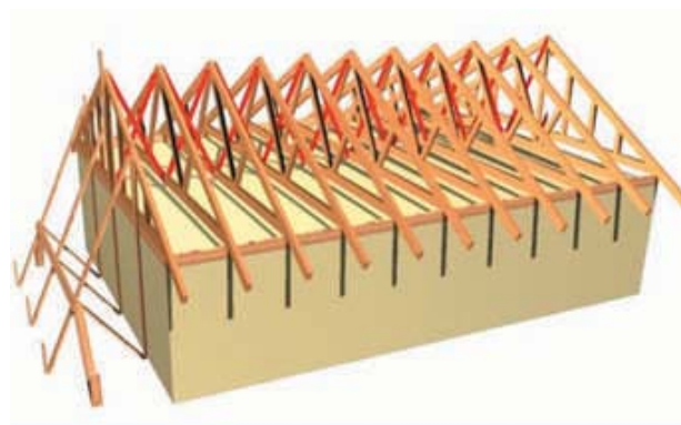
Figura 11-33: En rojo se destacan las riostras que van perpendiculares al plano de las diagonales. En caso de considerar que queden permanentes, su solución debe ser dada por el calculista.
