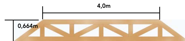
Figura II - 8: Determinación de la dimensión de cerchas trapezoidales.
