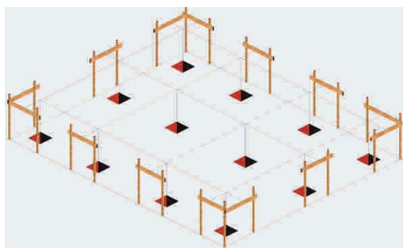
Figura 8 - 35: Cerco perimetral que permite replantear cada eje de los cimientos aislados según plano de fundaciones.
