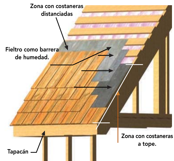
Figura 11-62: Arriostramiento de la techumbre con costaneras, las que además recibirán la solución de cubierta con tejas de madera.
