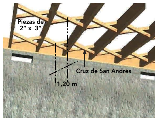
Figura 9 - 7: Vista desde abajo de la plataforma de madera anclada sobre una fundación continua. Crucetas con distancia máxima a 1,2 m según proyecto.
