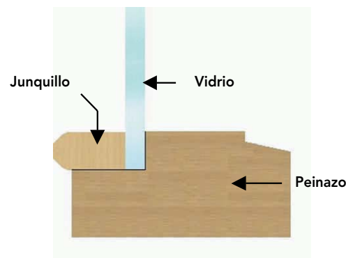
Figura 22 - 45: Vidrio colocado con junquillo de madera.
