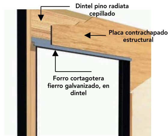
Figura 22 - 43: Forro cortagoteras o vierteaguas en dintel de ventana.
