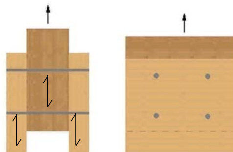
Figura 7- 18 : Carga paralela a la fibra.
