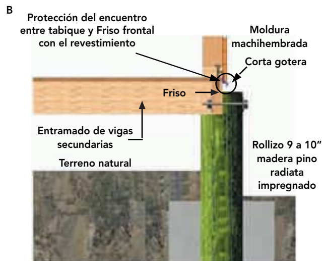
Figura 18 - 11b: Detalle del encuentro del revestimiento con fundación aislada, que debe cubrir al friso a lo menos en 50 mm, además del corta gotera correspondiente.
