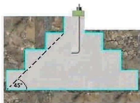
Figura 8 - 18: Caso de fundación en terrenos aluviales.
