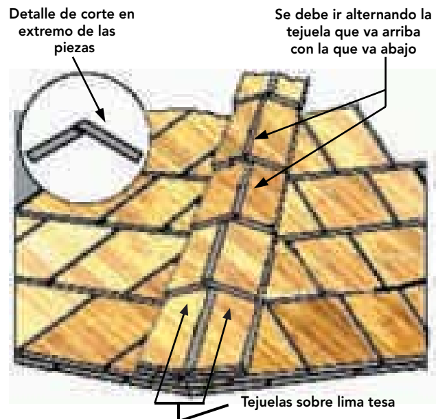
Figura 17-34 : Protección del encuentro de lima tesa con tejuelas de madera.
