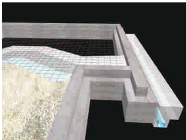
Figura 3 - 5: Tubo de P.V.C perforado adyacente al cemento y que colecta las aguas, evacuándolas al punto más bajo.
