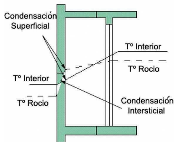
Figura 13 - 17: Condensación superficial e intersticial en clóset.
