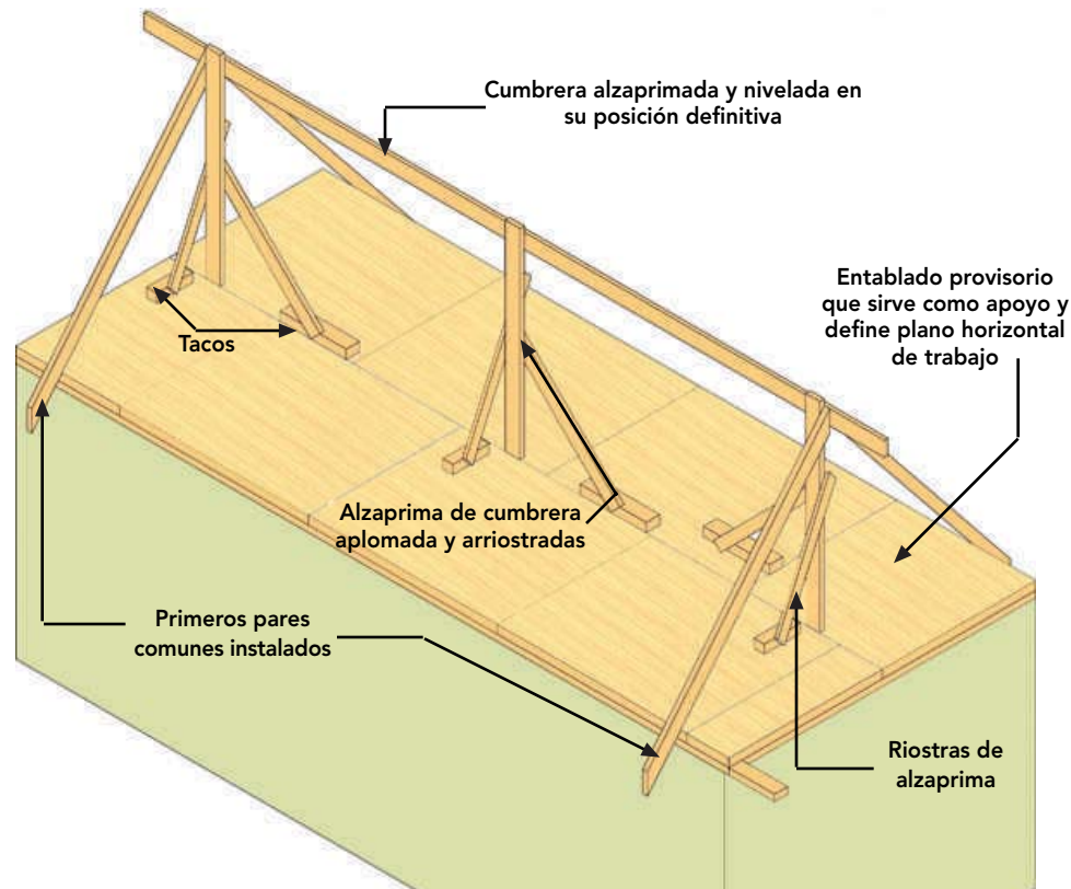
Figura 11-58 : Ejemplo de cómo iniciar el armado del tijeral en su posición definitiva. Se ven las alzaprimas temporales auxiliares para poder colocar en su ubicación definitiva la cumbra que luego recibirá los pares, conformando la techumbre definitiva.
