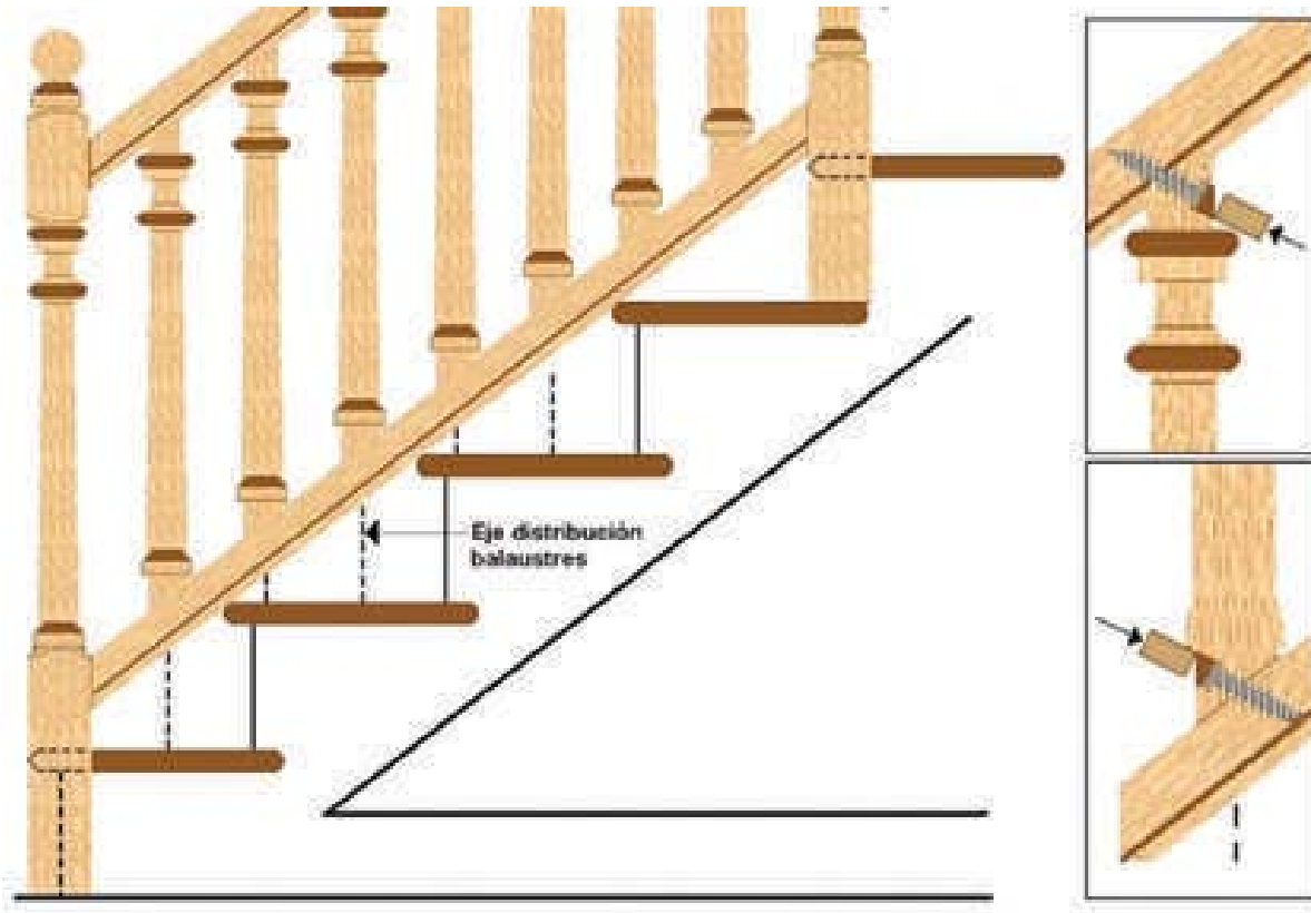
Figura 12 – 38: Fijación de balaustres y baranda mediante tornillos.
