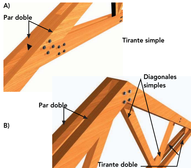
Figura 11-21: Unión de los elementos de una cercha mediante pernos. Figura A, encuentro entre tirante simple y pares doble. Figura B, encuentro entre diagonales simples y pares dobles.
