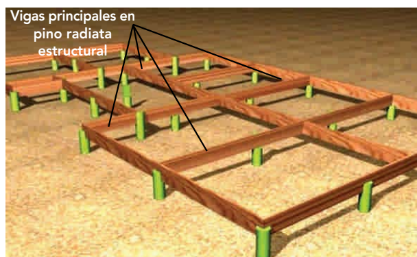
Figura 9 - 20: Ejemplo de vigas maestras o principales en entramados de piso sobre fundación aislada en Pino radiata estructural.
