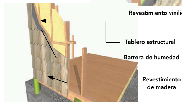
Revestimiento con tejas de madera
