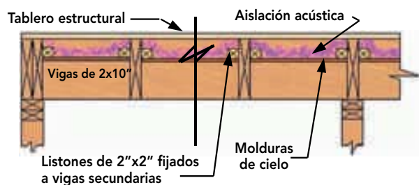
Figura 19-14: Corte de entrapado que muestra las molduras fijadas a listones, quedando las vigas a la vista.
