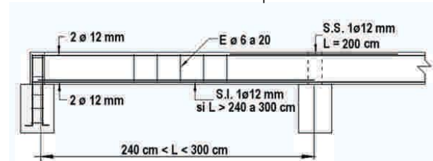
Figura 8 - 41: Plano detalle de la armadura de la viga de fundación.
