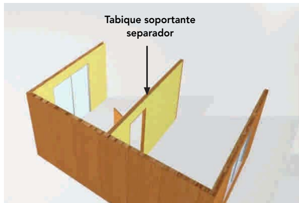
Figura 9- 33: En este caso se debe cubrir la luz entre los tabiques extremos y se cuenta con un tabique soportante separador entre estos.
