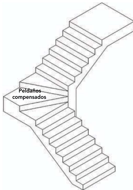
Figura 12 – 9: Isométrica de escalera de dos tramos en ángulo recto con peldaños compensados.
