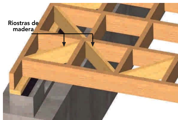
Figura 9 - 8 : Riostras de 2 x 8 en plataforma de piso, de igual escuadría que vigas secundarias.
