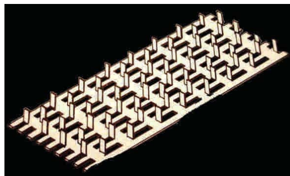
Figura 7-36: Placa metálica dentada de espesor mínimo de 1 mm.
