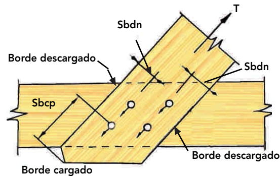
(A) Unión traccionada en pieza solicitante.
