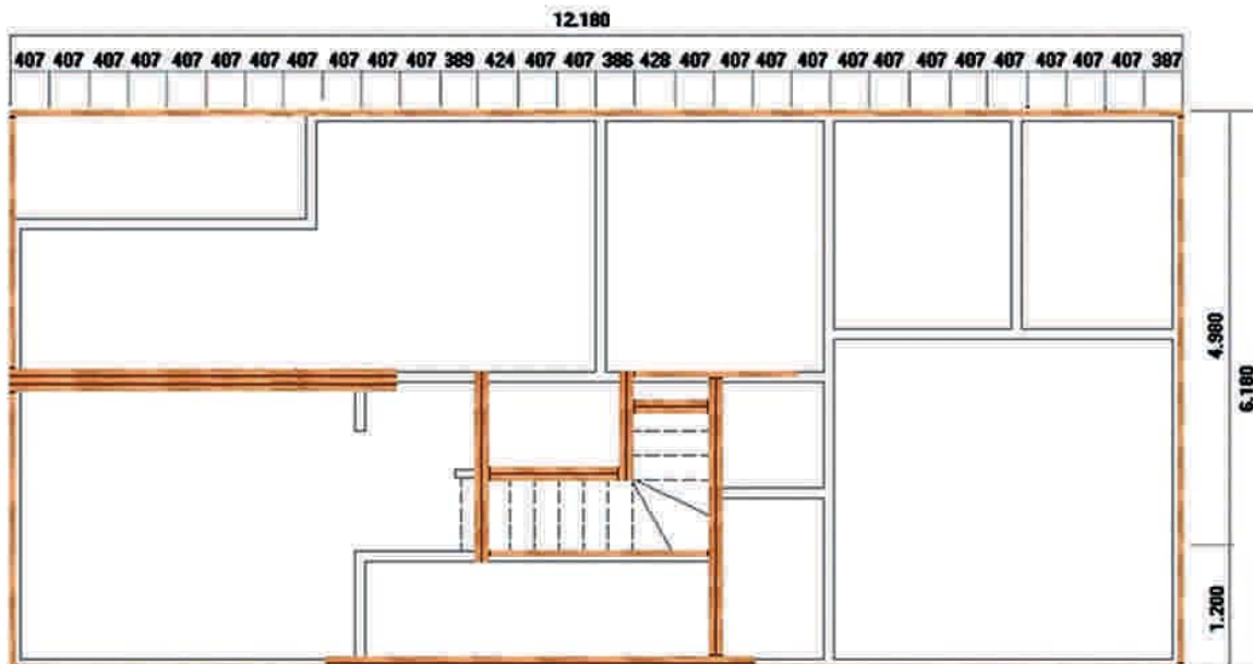
PLANO DE ELEMENTOS ESTRUCTURALES PRINCIPALES
