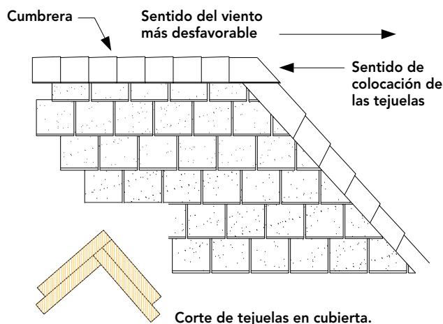
Figura 17 - 13: Los elementos que conformarán la cubierta deben ser instalados siguiendo el sentido contrario al que tiene el viento predominante de la zona.
