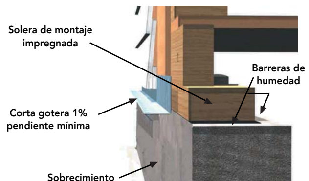
Figura 8 - 2: Solera de montaje impregnada con 8 \text{ kg/m}^3 de retención, anclada al sobrecimiento, protegida del contacto directo del hormigón con una barrera de humedad (doble fieltro asfáltico).
