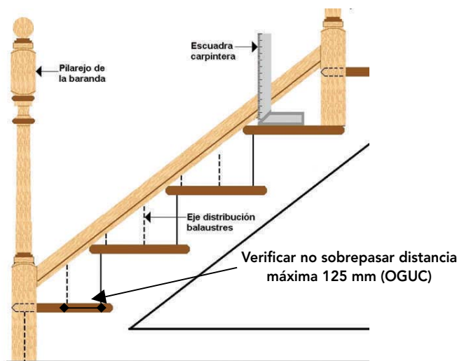
Figura 12 - 36: Armado de la baranda de la escalera. Se puede observar la colocación de los pilarejos y la presentación y forma de atraque del zócalo.
