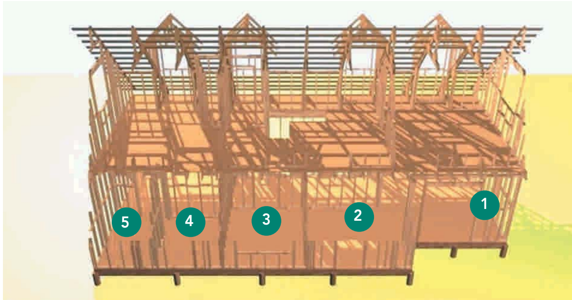
CORTE VIVIENDA TIPO EN VISITA A OBRA PISO 1°
