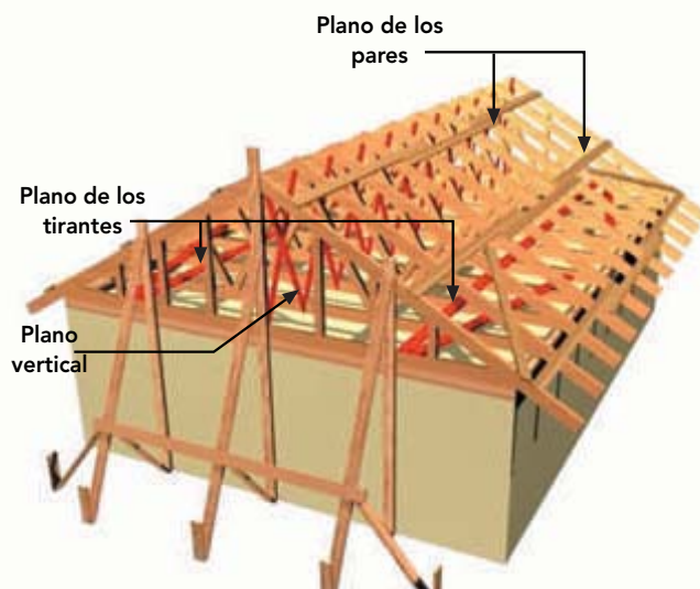
Figura 11-30: Planos en los que se deben realizar los arriostamientos de las cerchas.
