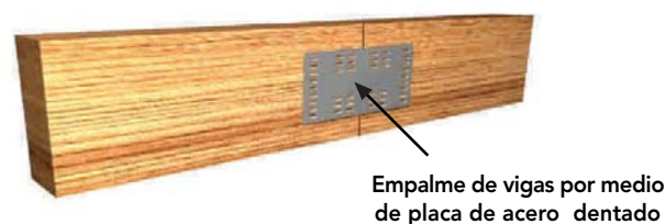
Figura 9 - 37: Las uniones con placas metálicas dentadas se pueden usar sólo en componentes constructivos, solicitados predominantemente por cargas estáticas.
