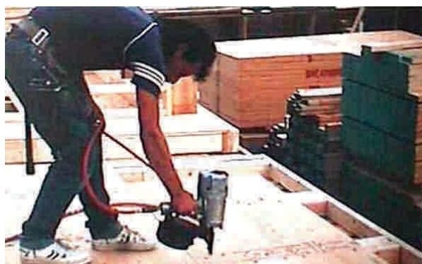
Figura 10 - 33: Fijación de contrachapado estructural al entramado por medio de clavadoras de aire comprimido.
