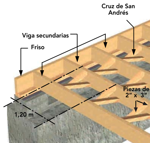
Figura 9 - 6: Crucetas de 2" x 3" en plataforma de primer piso, conformado por vigas principales de 2" x 10".
