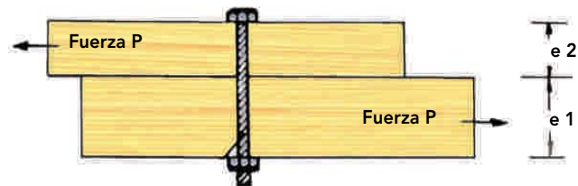
Figura 7- 6 : Unión con perno sometida a cizalle.
