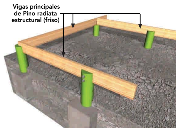
Figura 9 - 30: En el ejemplo, se muestra el friso que remata el contorno del entramado de piso en una solución de fundación aislada.
