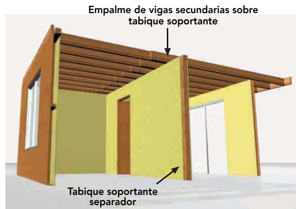
Figura 9 - 35: Vista en perspectiva de la solución del empalme traslapado de las vigas de la plataforma del entrepiso.
