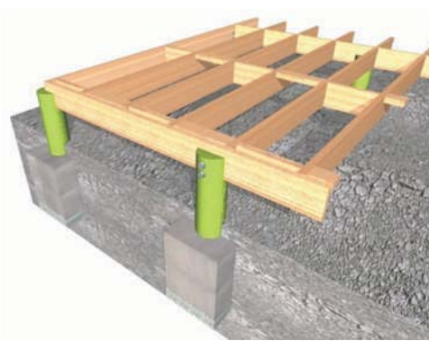
Disposición de cadenas estructurales y de apoyo a tableros.
