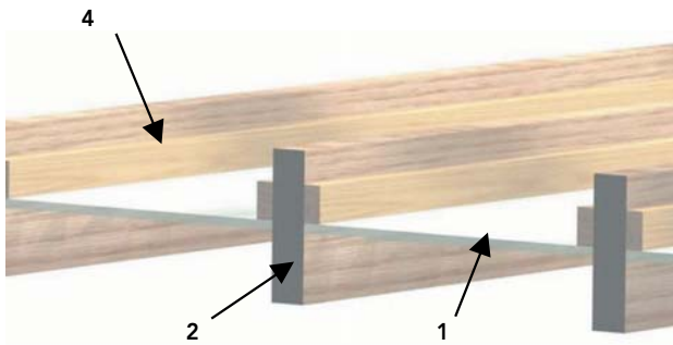
Figura 14 - 69: Colocación de plancha de yeso cartón como revestimiento de cielo soportado por listones de 1"x 2", fijadas a las vigas del entramado de entepiso.
