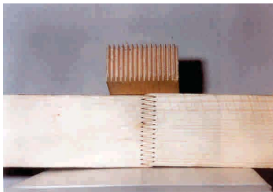
Figura 7-38: Uniones mediante finger-joint.
