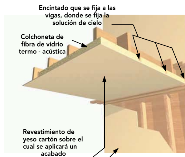
Figura 19-2 : Revestimiento de cielo y paramentos verticales en placa de yeso cartón sobre los cuales se aplicará un acabado.
