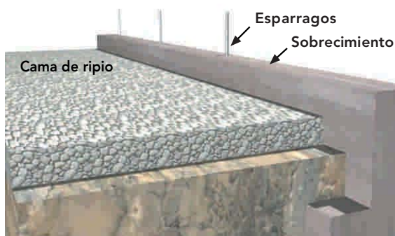
Figura 8 - 53: Colocación de la cama de ripio de espesor de 8 a 10 cm.
