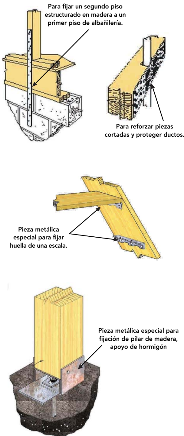
Figura 7-35: Existen variados conectores para unir o fijar los más diversos elementos.
