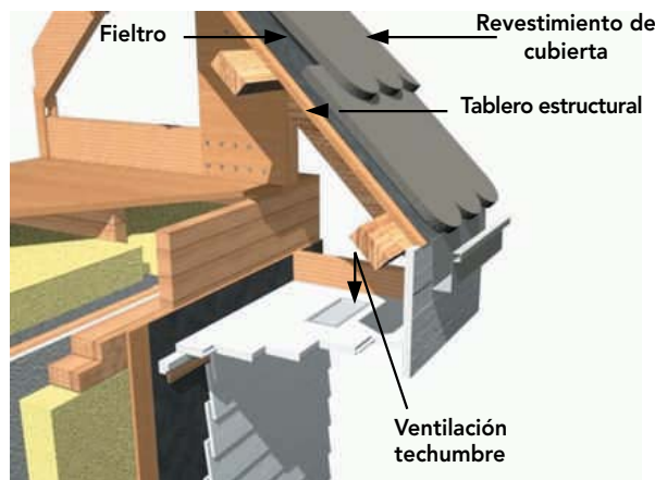
Figura 17-17 B: Sobre el tablero estructural se instala la barrera de humedad (fielto) y sobre éste la solución de revestimiento.
