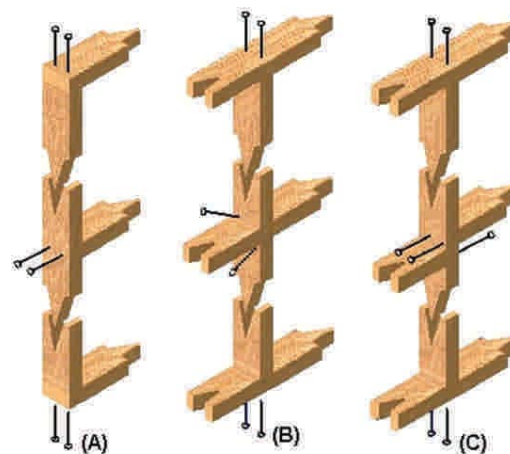
Figura 10 - 29: Distribución y colocación de clavos en piezas componentes de un muro soportante o tabique.
