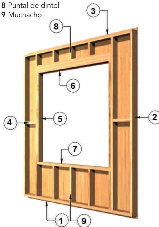
Figura 10 - 6: Piezas principales que componen un entramado vertical.
