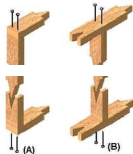
Figura 7-3 : Unión de piezas mediante clavos, en tabiques, (A) pie derecho inicial (B) pie derecho intermedio.
