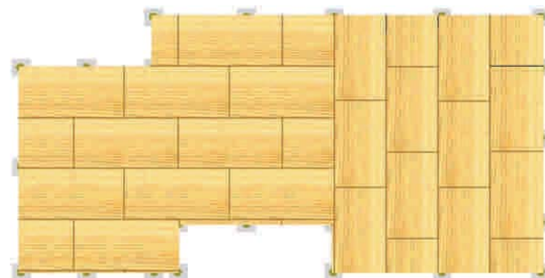
Figura 9 - 13: El plano de planta de construcción debe especificar la disposición de los tableros estructurales: contrachapado fenólico (terciado estructural) o de hebras orientadas (OSB).
