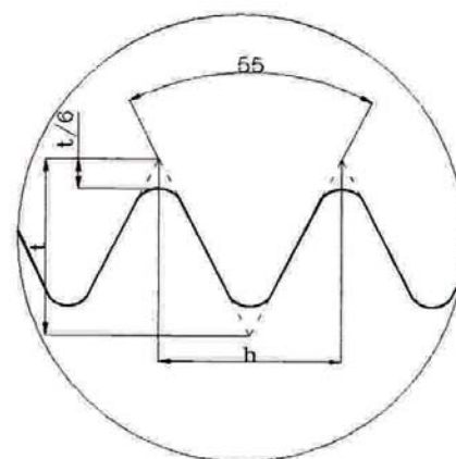
Figura 7-29: Detalle de la rosca Whitworth.
