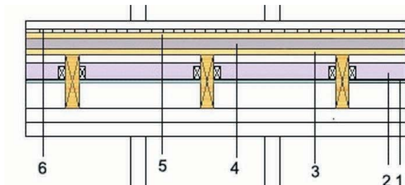
Figura 14-76: Representación técnica de la estructura de entrepiso, envigado a la vista y piso con revestimiento en madera.
