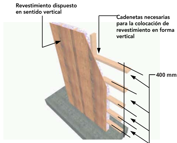
Figura 18 - 44: Clavado del revestimiento cada 400 mm, tanto en sentido vertical como horizontal.
