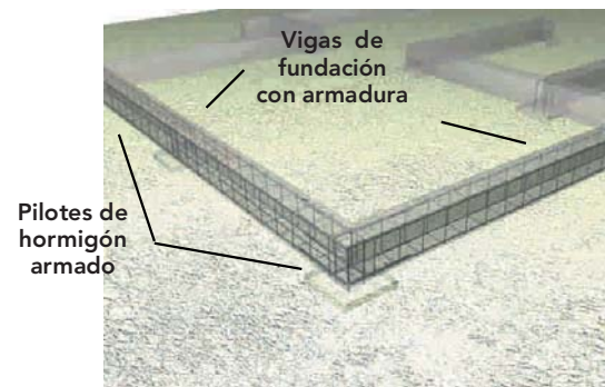
Figura 8 - 42: Viga de fundación hormigonada con suples correspondientes.
