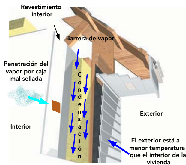
Figura 16-11: Figura que muestra situación de riesgo de condensación.
