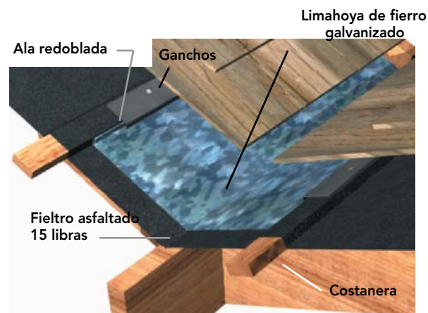
Figura 17- 35A : Solución de limahoya, para cubierta de tejuela sobre costaneras.
