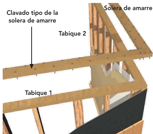
Figura 10 - 17: Solera de amarre en encuentro esquina, entre tabiques perimetrales soportantes. Clavos se ubican en forma alternada cada 15 cm.
