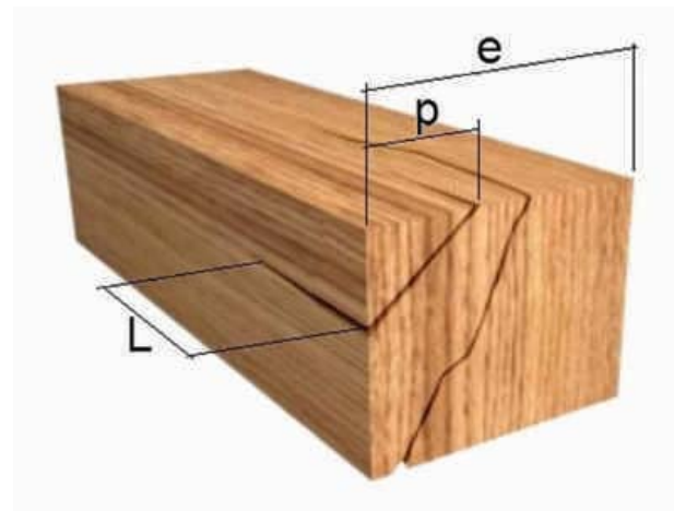
Figura 1- 46: Medición de la longitud de la zona afectada por la rajadura.
