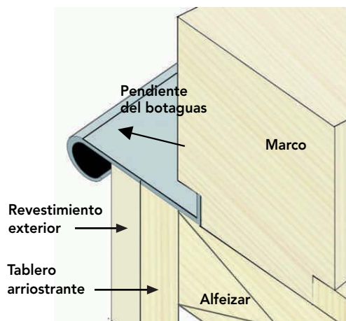
Figura 22 - 41: Botagua en hierro galvanizado 0,5 mm con pendiente de 15°.
