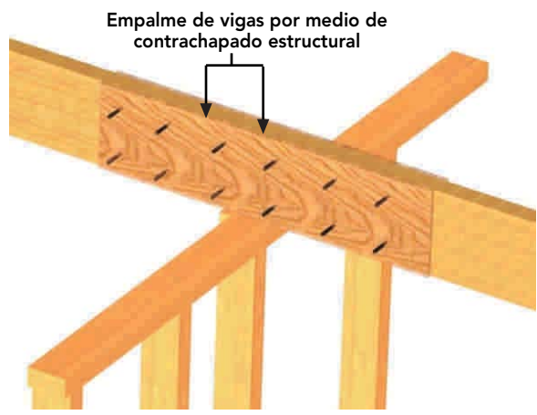
Figura 9 - 39: Empalme a tope sobre tabique soportante, reforzado con conector de contrachapado fenólico (distancia entre fijaciones según cálculo).
