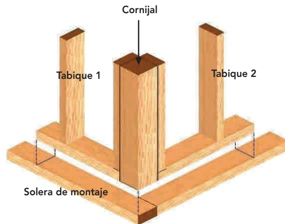
Figura 10 - 19: Cornijal para encuentro en esquina.
