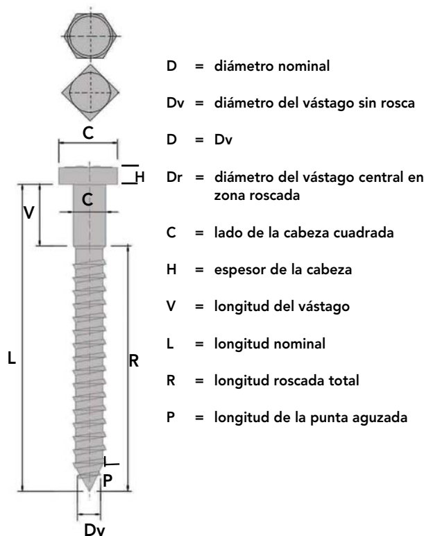
Figura 7-26: Esquema de un tirafondo.
