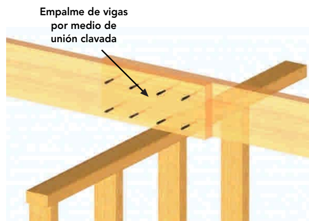
Figura 9 - 36: Ejemplo de empalme de dos vigas de 2 x 8 unidas con clavos de 4" según cálculo. Apoyo sobre el tabique soportante como se explicó en la sucesión de figuras anteriores.
