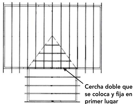
Figuras 11-35: Planta de techumbre en la cual se aprecia la disposición de las cerchas de limahoya y el refuerzo de doble cercha que debe ser colocado.
