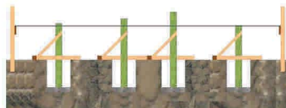
Figura 8 - 46: Control geométrico de los pilotes, planimetría y altimetría según plano. Arriostramiento de pilotes para cuidar la verticalidad durante el hormigonado del cimiento.
