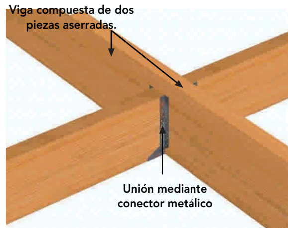
Figura 9 - 58: Unión de viga secundaria de tope a viga principal compuesta mediante conector metálico, según cálculo.
