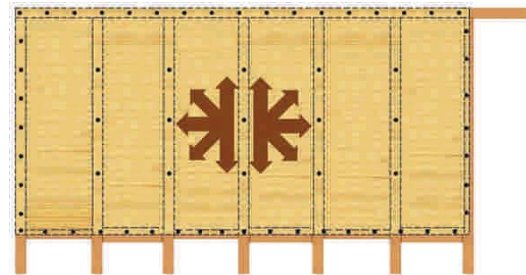
Figura 7-5 : Unión de placa terciada fenólica como elemento arriostrente con clavos o tornillos al entramado horizontal.
