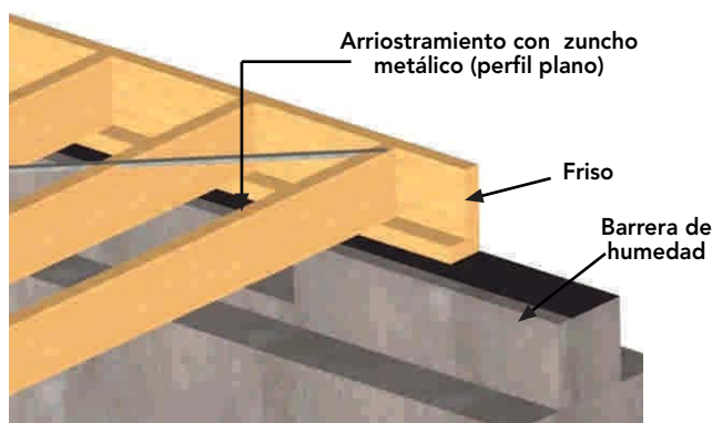
Figura 9 - 10 : Zuncho metálico, pletina de ancho 20 mm y espesor 2,5 mm para plataforma de primer piso, anclada a la fundación continua.
