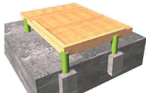
Figura 8 - 16: Plataforma de madera que se construye sobre la estructura de la fundación aislada, conformando el primer piso de la vivienda.
