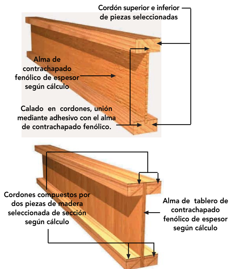
Figura 9 – 62: Viga doble T, formada por un alma de contrachapado fenólico con cordones (superior e inferior) de piezas dobles seleccionadas.
