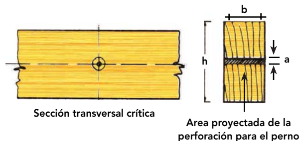
Figura 7-7 : Sección transversal neta de la unión para una pieza con un perno.
