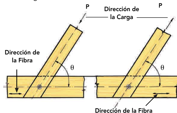
Figura 7-8 : Carga inclinada respecto a la fibra de la madera.
