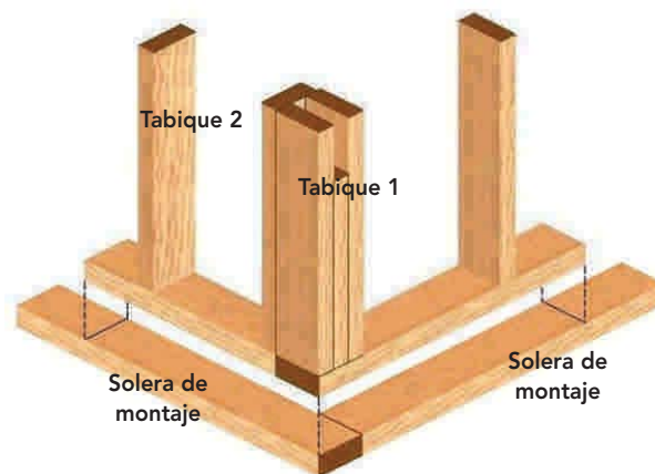
Figura 10 - 15: Solera de montaje que se ancla a la plataforma sobre la cual se alzarán los tabiques.
