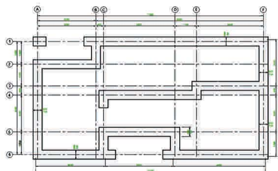
Figura 8 - 24: Plano de excavaciones de la vivienda prototipo.
