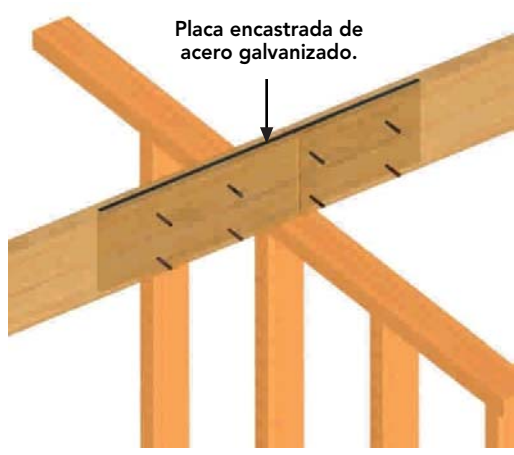
Figura 9 - 40: Empalme a tope sobre tabique soportante, reforzado con placa encastrada de acero galvanizado (distancia entre fijaciones según cálculo).
