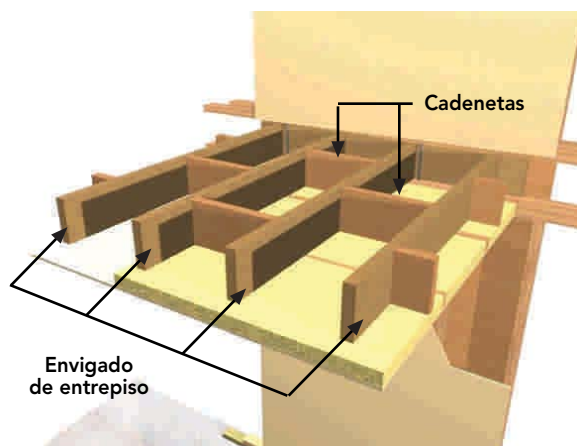
Figura 9 - 5: Piezas de madera dispuestas en forma normal, de sección similar a las vigas secundarias del entrepiso.
