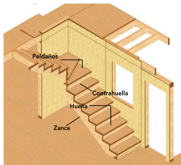
Figura 12 – 12: Vista isométrica de los componentes de una escalera de madera.
