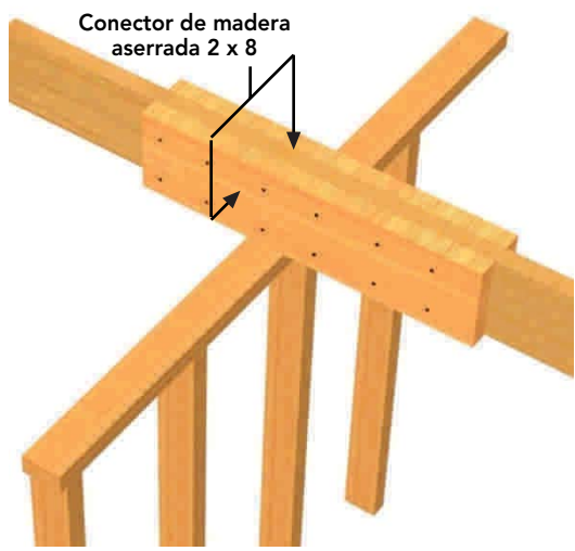
Figura 9 - 38: Empalme a tope sobre tabique soportante, reforzado con conector de madera de 2 x 8 (distancia entre fijaciones según cálculo).
