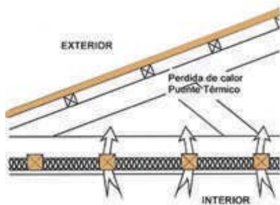
Figura 13 - 18: Puente térmico. Por la trascara de la plancha de yeso (interior) el sector donde la plancha no se encuentra aislada presenta franjas oscuras, debido a que la diferencia de temperatura en dicho sector es menor de la plancha de yeso del cielo.
