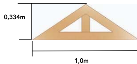
Figura II - 15: Dimensiones de las distintas cerchas involucradas.
