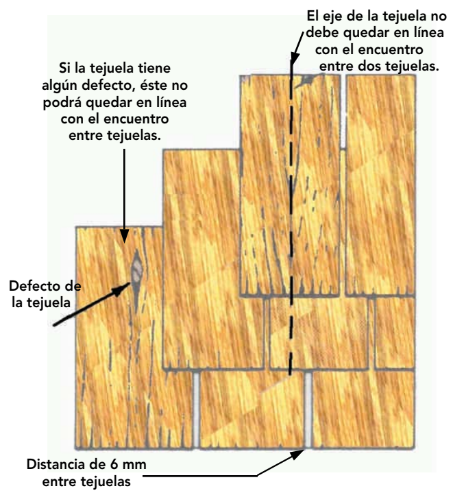
Figura 17-29: Restricciones de las tejas en su colocación.
