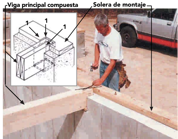
Figura 9 -57: Fijación de la viga maestra compuesta de Pino radiata estructural. Previamente se ha dejado el espacio necesario para su ubicación en el sobrecimiento continuo, cuidando que coincida con la altura de la solera de montaje de los tabiques estructurales perimetrales. Se debe considerar una huelga de 5 a 8 mm como se observa en el detalle (1), para colocar espuma de poliuretano impregnada con bitumen asfáltico, que asegure aislar la humedad por capilaridad a la viga al contacto con el hormigón.
