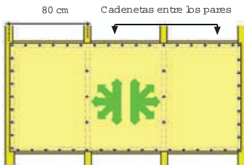
Figura 11-64 : Clavado de placa a los pares, de cerchas o diafragma inclinado, ubicados cada 80 cm y a cadenetas ubicadas en el perímetro de la placa.
