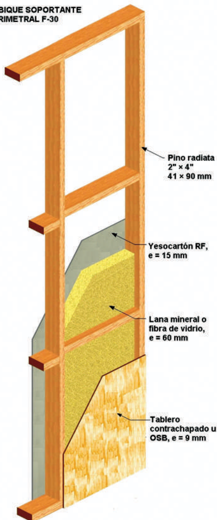
Figura 15 - 26: Solución mínima F-30 para tabiques soportantes perimetrales. Una o dos filas de transversales cortafuego son opcionales.
