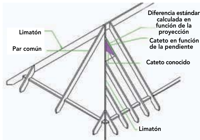
Figura 11-54: Dedución del cálculo de la diferencia estándar, en base a la distancia entre pares y la pendiente de la techumbre.
