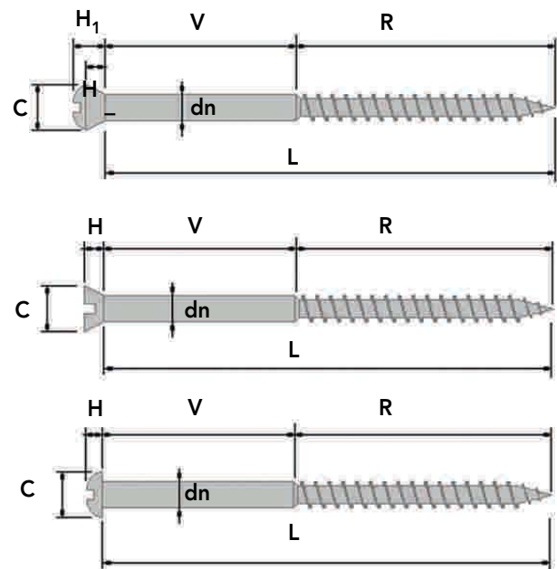
Figura 7- 25 : Detalles de tornillos con cabeza plana, oval y redonda.
