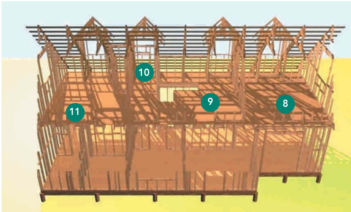
CORTE VIVIENDA TIPO EN VISITA A OBRA 2° PISO
