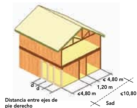
Figura V - 5: Situación para un pasillo interior de ancho máximo de 1.20 m, en viviendas de 2 pisos.
