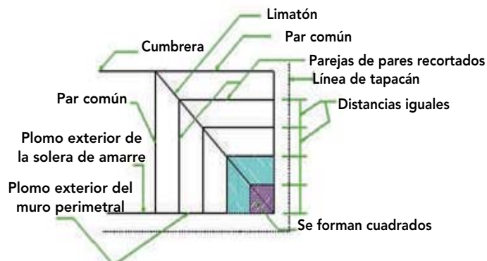
Figura 11-51: Vista en planta de los cuadrados proporcionales generados por las proyecciones de los pares comunes y pares recortados formados en la esquina, siendo los lados del cuadrado mayor, los dos pares comunes que se aprecian en la vista.
