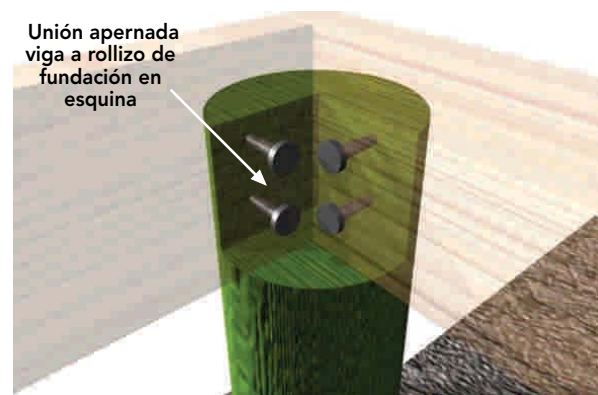
Figura 9 - 26: Solución unión esquina de dos vigas perimetrales, dimensiones 2" x 10", que se apoyan sobre un pilote de diámetro 10". Unión realizada en este caso mediante dos tirafondos de dimensiones definidas, según cálculo y bajo supervisión.
