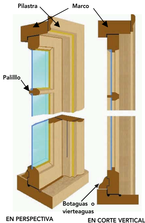
Figura 22 - 31: Ventana que abre hacia el interior. Perspectiva de una sección vertical, en que se aprecian sus partes.
