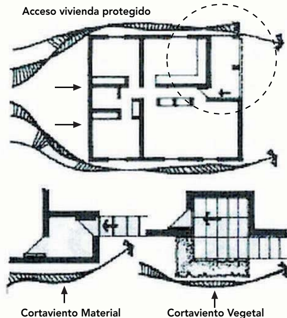
Figura 14 – 50: Ubicación y protección del acceso a la vivienda.
