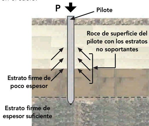
Figura 8 - 6 : Fundación de pilotes.
