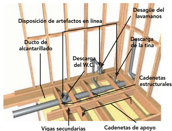
Figura 16-2: En la figura se observan las descargas de artefacto de W.C., lavamanos y tina dispuestos en línea. La descarga perfora las cadenas de la estructura de plataforma. Las vigas y cadenas del ejemplo son de escuadría 2" x 10".
