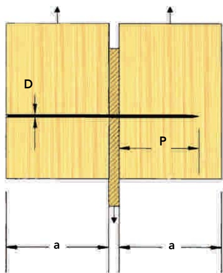
A Cizalle doble
