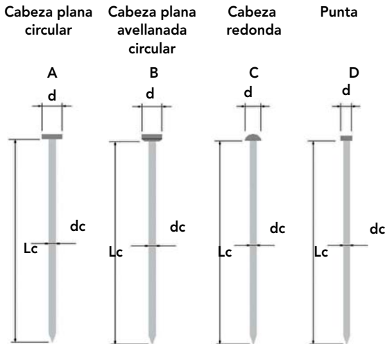
Figura 7- 13 : Clasificación de clavos según los distintos tipos de cabezas, norma NCh 1269.
