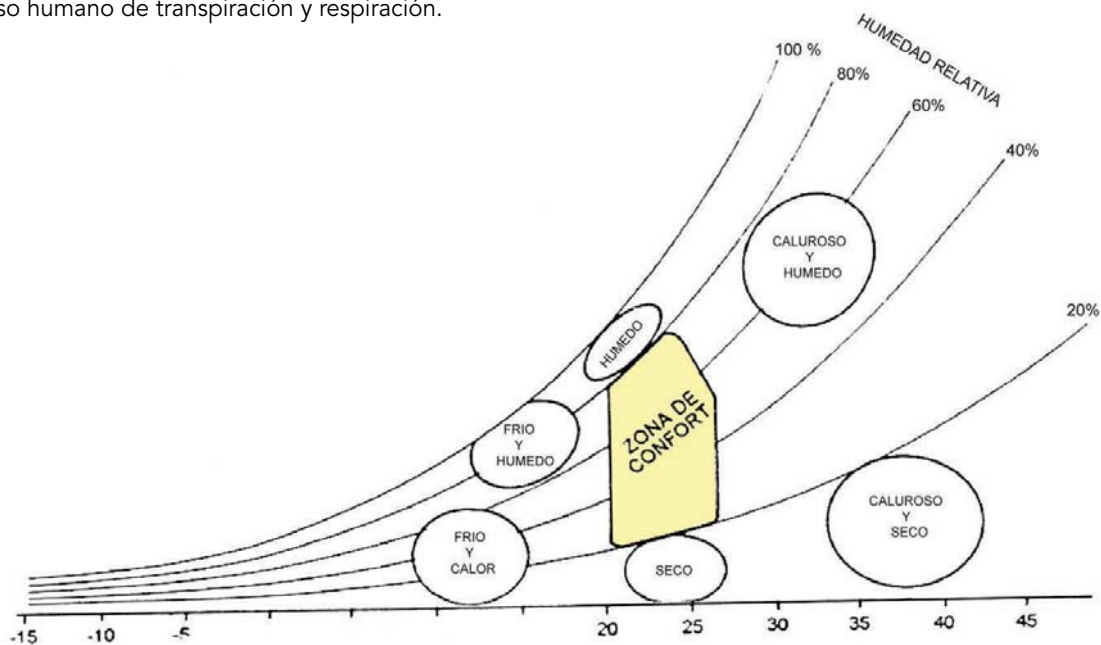
Gráfico 13 - 3: Gráfico psicométrico. Zona de confort interior. 20 ° - 26 °C y humedad relativa 20 % - 80 %.
