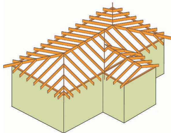
Figura 11-14: Techumbre materializada con diafragma inclinado.
