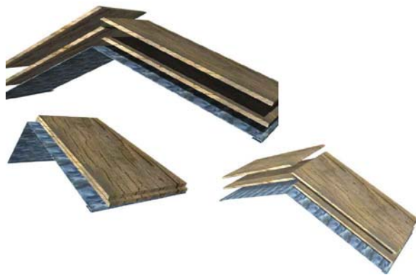
Figura 17-33 : Secuencia en la colocación de los elementos que conforman la cumbrera.
