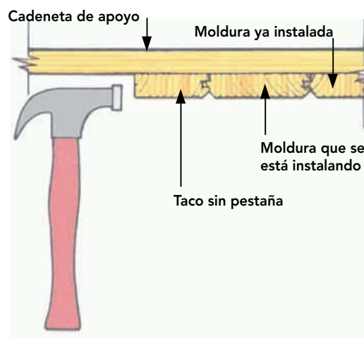
Figura 19 - 32: Corte de tabique donde se muestra taco que ayuda a asegurar el calce entre las molduras machihembradas.
