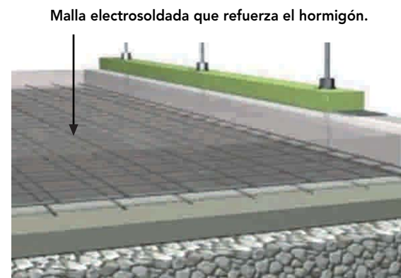
Figura 8 - 56: Colocación de la malla electrosoldada sobre separadores plásticos de 2 cm sobre la barrera de humedad.
