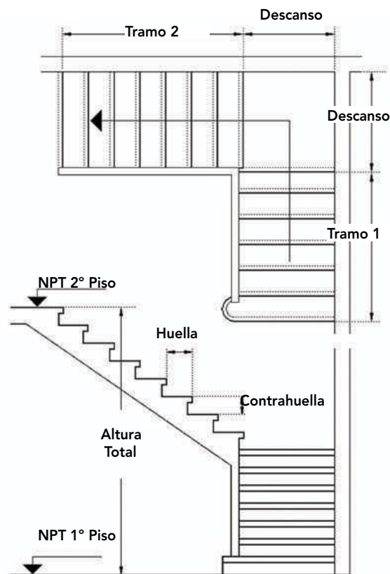
Figura 12 – 4: Planta y elevación tipo de una escalera de dos tramos en ángulo recto con descanso.
