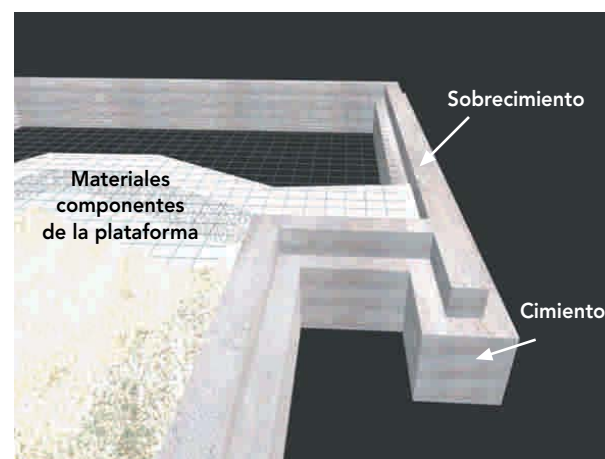
Figura 8 - 7 : Típica solución de fundación continua en plataforma de hormigón, con buena calidad de suelo. Solución ideal de fundación superficial para vivienda estructurada en madera.
