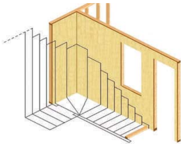
Figura 12 - 26: Trazado de la proyección horizontal y vertical de la escalera y ubicación de la pieza de anclaje (madera o conector metálico), para la fijación de apoyo de los largueros.
