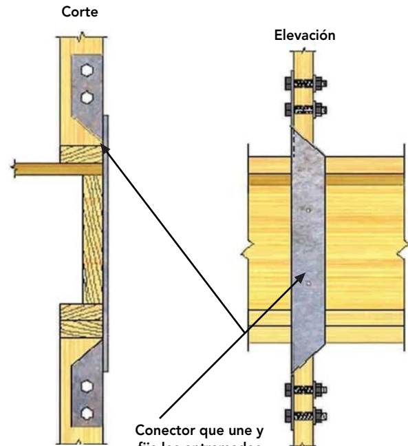
Conector para fijar entramado vertical a fundación corrida
