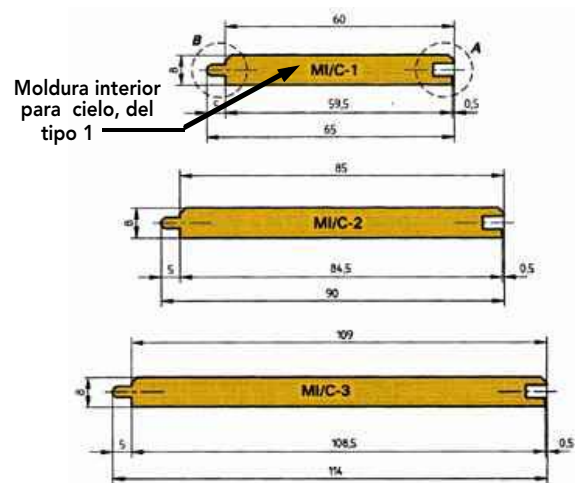
Figura 19-18: Ejemplo de las molduras machihembradas para cielo que define la norma NCh2100.
