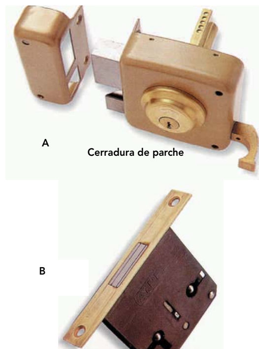
Figura 22 -16: A) Cerradura de parche con caja y pestillo. B) Cerradura embutida para puertas interiores.
