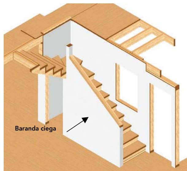
Figura 12 – 17: Baranda de escala de tipo ciega, la cual se prolonga a partir del tabique de apoyo lateral.
