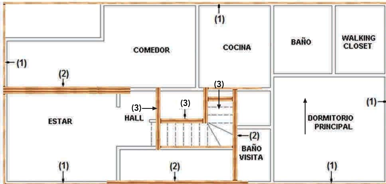
Figura 9 – 31: Plano planta de vigas perimetrales (friso) (1), viga compuesta (2), necesarias según cálculo para reforzar al envigado por distanciamiento de los apoyos y viga cabezal (3) como refuerzo en el perímetro de la escotilla de la escalera.
