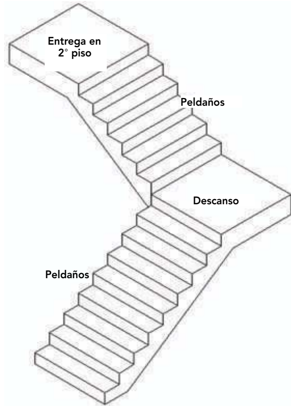
Figura 12 – 8: Isométrica de escalera de dos tramos en ángulo recto con descanso.
