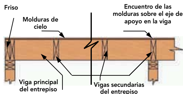
Figura 19-13: Corte de entrapado que muestra las molduras apoyadas y fijadas sobre el envigado, quedando las vigas a la vista. Sobre éstas se debe considerar la base para la solución de pavimento y aislación acústica.
