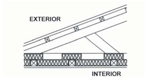
Figura 14 -17a: Material aislante rígido en cielo horizontal.
