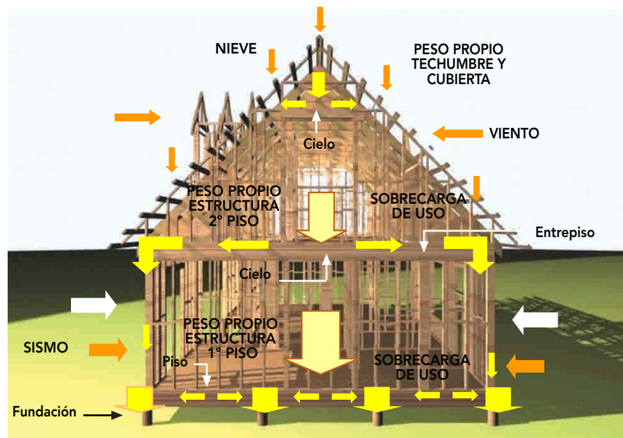
Figura 9 - 2: Los entramados horizontales absorben las cargas permanentes, variables y las fuerzas laterales transmitiéndolas a las estructuras soportantes tales como: tabiques, vigas principales, pilares y finalmente al terreno; en este caso, a través de la solución de fundaciones aisladas.
