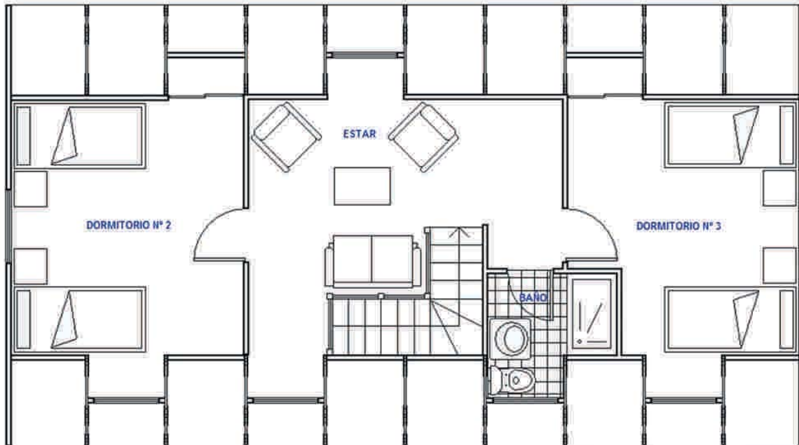
PLANO PLANTA DE ARQUITECTURA 2° PISO
