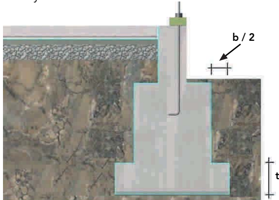
Figura 8 - 21 : Ancho máximo de la zarpa sin armar.
