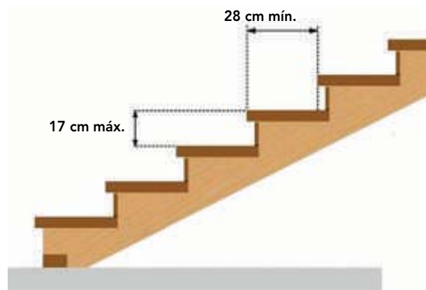
Figura 12 – 13: Dimensiones reglamentarias para escaleras de viviendas unifamiliares según OGUC.
