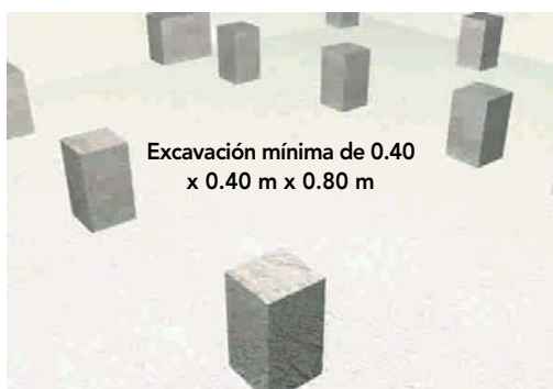
Figura 8 - 36: Corte realizado a nivel del emplantillado que muestra las excavaciones que se deben realizar para los cimientos.
