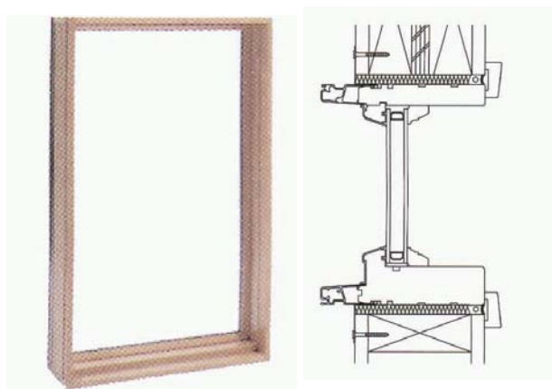
Figura 22 - 22: Ventana fija.
