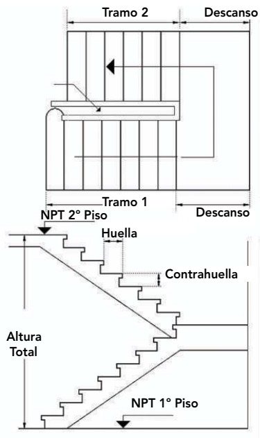
Figura 12 – 6: Planta y elevación tipo de una escalera de dos tramos rectos con descanso de media vuelta.
