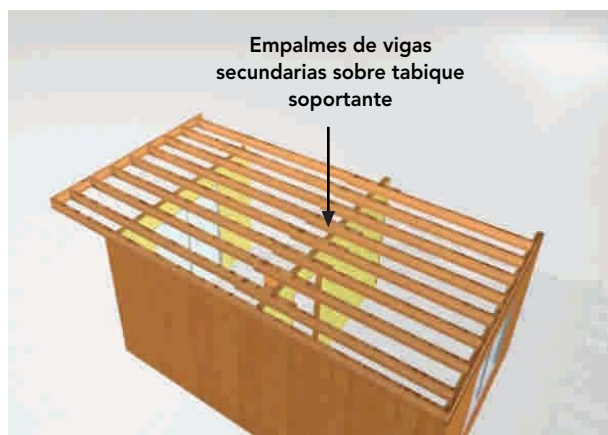
Figura 9 - 34 : Se ubican las vigas que conformarán la plataforma del entrepiso. Dichas vigas se traslapan sobre el tabique soportante separador.
