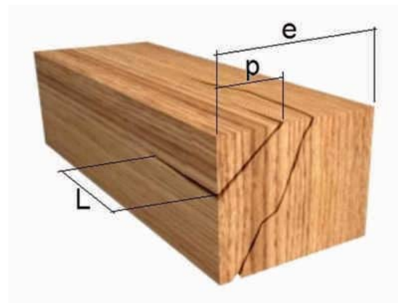
Figura 1 - 56: Medición de la longitud de la zona afectada por rajadura.
