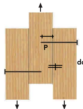
Figura 7- 16 : Resistencia lateral, cizalle simple.
