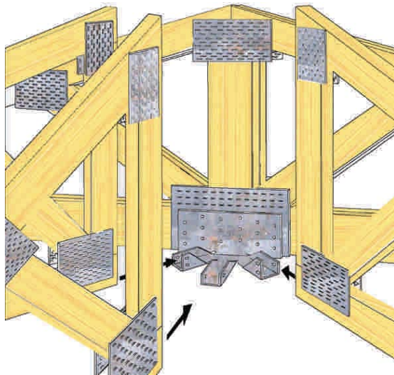
Figura 7- 33 : Alternativas de conectores metálicos para fijar elementos verticales como tabiques o pie derecho.
