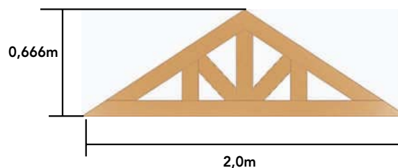
Figura II - 13: Como determinar la magnitud a disminuir a cada cercha.
