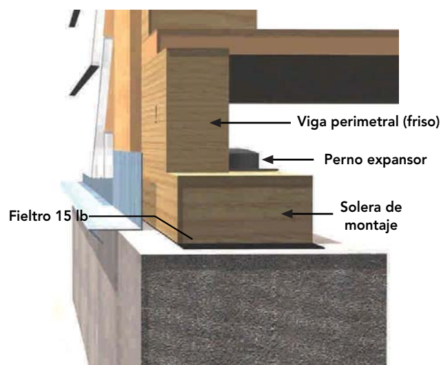
Figura 9 - 21: Solución de conexión de la viga perimetral al sobrecimiento, a través de una solera de montaje tratada con preservante CCA. Considera además, aislamiento entre ambos materiales con fieltro alquitranado. La solera está anclada al sobrecimiento mediante espárragos o pernos expansores cada 80 cm.
