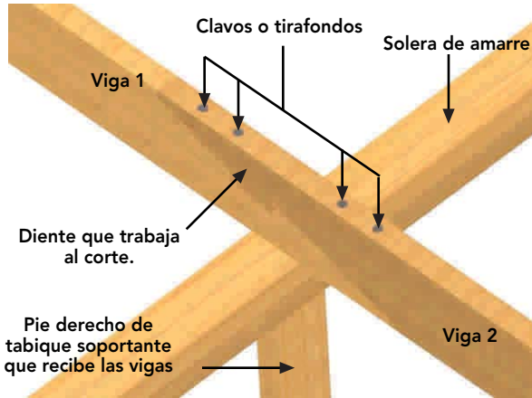
Figura 9 – 43: Empalme de dos vigas llamado Rayo de Júpiter sobre tabique estructural, en el cual las vigas se cruzan como en la solución Entablatura , pero incorporando un diente que trabajará al corte. Se puede utilizar en su fijación pernos o clavos.
