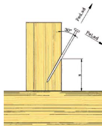
Figura 7- 22 : Detalle para la correcta colocación de clavos lanceros.
