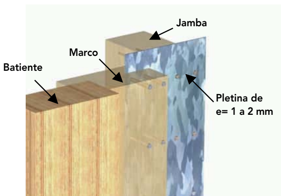
Figura 22 - 39: Sistema flexible.
