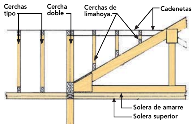
Figura 11-36: Elevación que muestra cadenetas entre cerchas.
