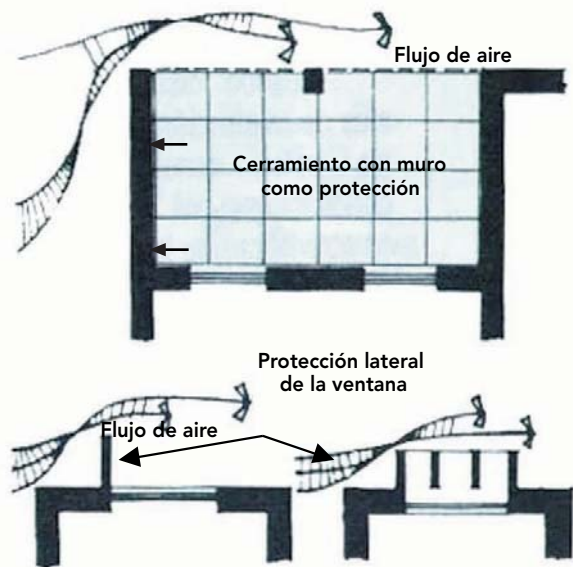
Figura 14 – 48: Protección de las aberturas.
