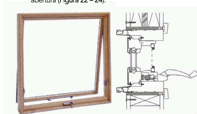
Figura 22 -24 : Ventana de quicio fijo horizontal.
