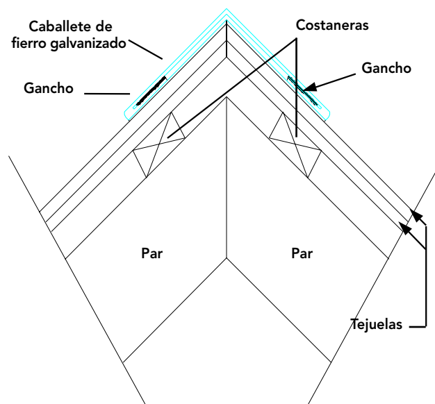
Figura 17-32: Corte de la cumbrera donde se ve la fijación del protector de fierro galvanizado.
