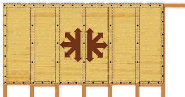
Figura 9 - 15: Instalación de tablero con clavos o tornillos, sin adhesivo sintético. Considera la fijación desde el centro hacia los bordes.
