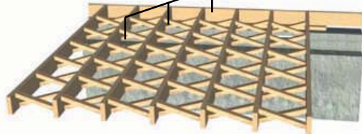
Figura 16-7: La utilización de cruz de San Andrés permite colocar ductos paralelos a vigas secundarias, sin tener que perforar cadenas.
