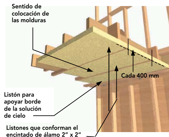
Figura 19-15: Ubicación de los listones que conformarán el encintado.
