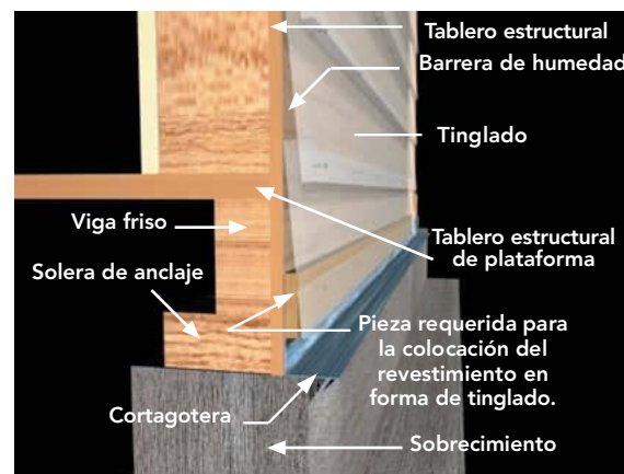
Figura 18 - 25: Inicio de la colocación del revestimiento, sobre la solera de anclaje con viga friso sobre fundación continua, con plataforma de madera en el primer piso.
