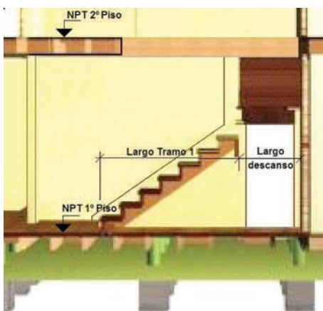
Figura 12 - 20a: Largo total de la escalera tramo 1.
