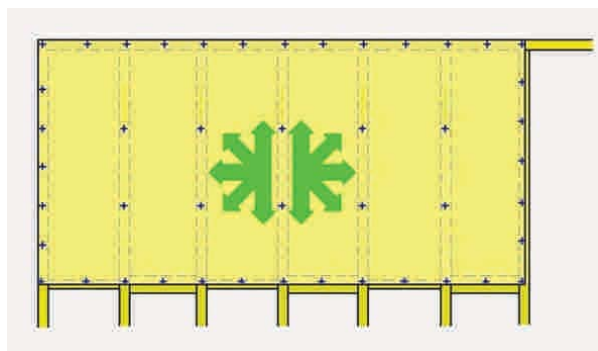
Figura 9 - 16: Instalación de tablero con clavos o tornillos con adhesivo sintético. Considera que la fijación se debe iniciar desde el centro hacia los bordes.
