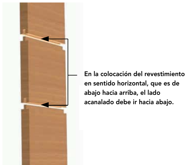
Figura 19 - 28: Secuencia de la colocación de molduras como revestimiento de paramento.
