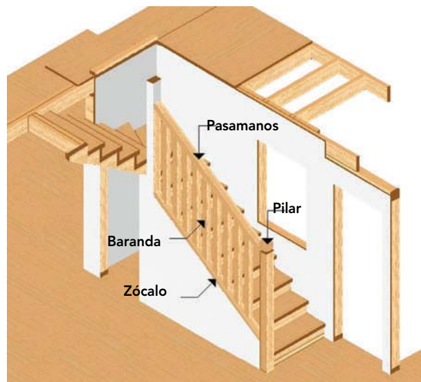
Figura 12 – 16: Baranda de escala de tipo semitransparente, conformada por pasamanos, zócalo y balaustres de madera.
