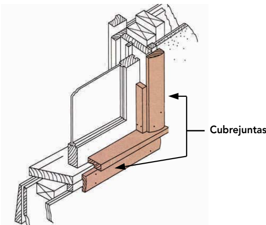
Figura 21 - 17: Cubrejuntas en ventanas.
