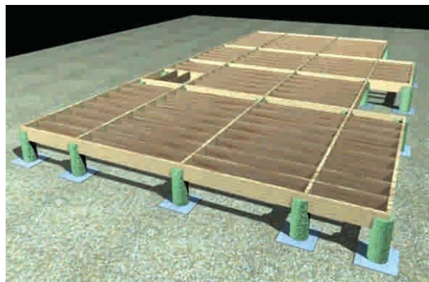
Figura 9 – 4: Vigas de Pino radiata estructural, de escuadrías según cálculo, normalmente de 2" x 8" o 2" x 10" que conforman el entramado de piso en fundación aislada sobre pilotes de madera.
