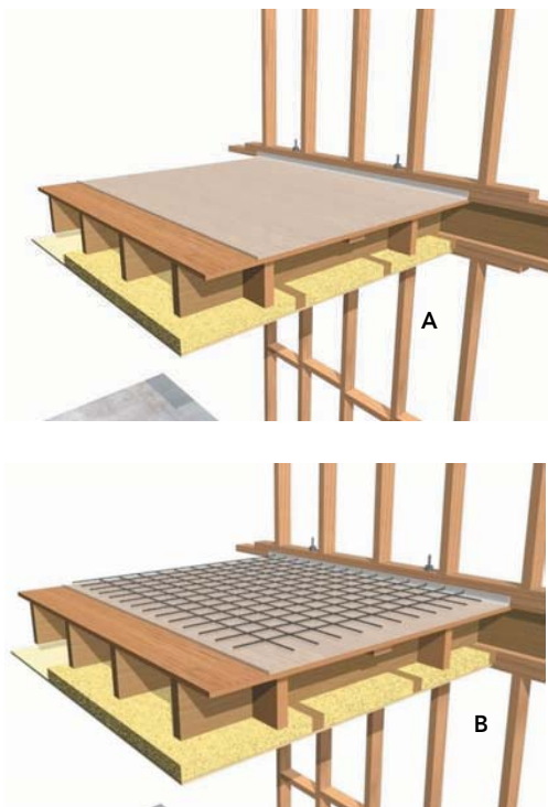
Figura 14-37: A Instalación de barrera de humedad de polietileno especial, espesor 10 mm, sobre el entepiso que cumple el objetivo de impedir el paso de humedad y de barrera acústica. B Instalación de malla electro soldada, fierro de diámetro de 4.3 mm como refuerzo de la loseta acústica. C Loseta de hormigón gravilla de H18, solución de piso, moldura Pino radiata de 1x4 machihembrada.
