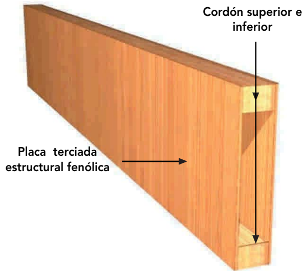
Figura 9 – 63: El material más utilizado en las vigas cajón como recubrimientos laterales es el contrachapado, por su alta resistencia.
