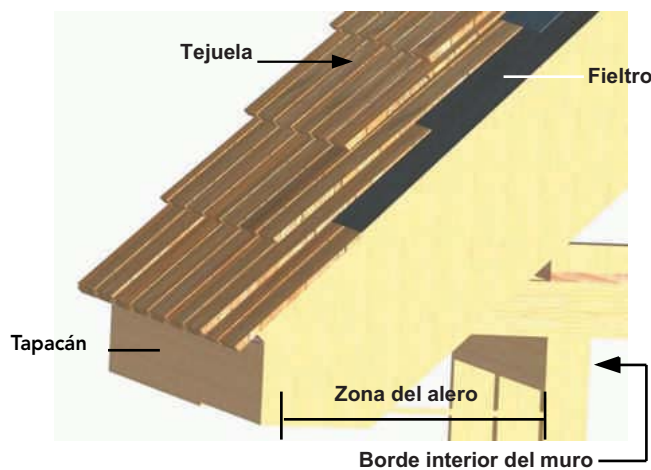
Figura 17-15: Fieltro debe cubrir al inicio de la techumbre el alero y al menos 300 mm pasados el borde interior del muro perimetral.
