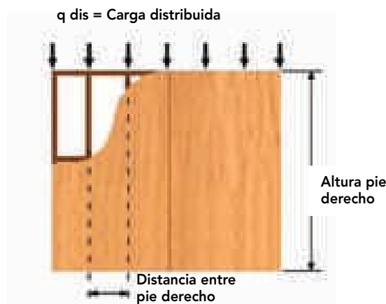
Figura V- 3: Tabique estructural no expuesto al viento.
