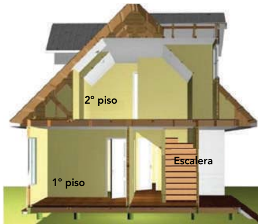
Figura 12 - 1a: Corte transversal de la vivienda tipo en que se observa la escalera que comunica ambos pisos de la misma.
