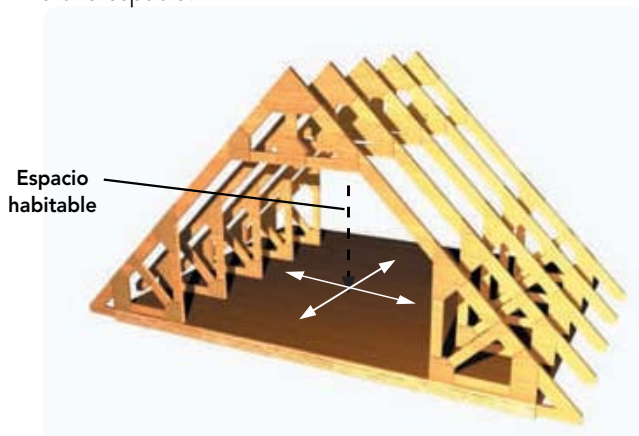
Figura 11-15: Cerchas habitables que forman la mansarda.
