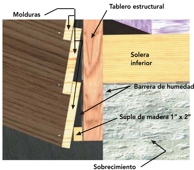
Figura 18 - 6: Revestimiento tinglado.
