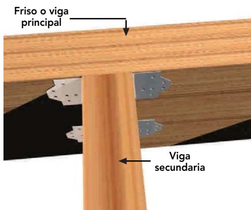
Figura 9 – 48: Conector de acero galvanizado de 1,7 mm de espesor utilizado para unir friso con vigas maestras de piso o entrepiso. Soporta bien las fuerzas paralelas y perpendiculares que puedan recibir las vigas maestras.
