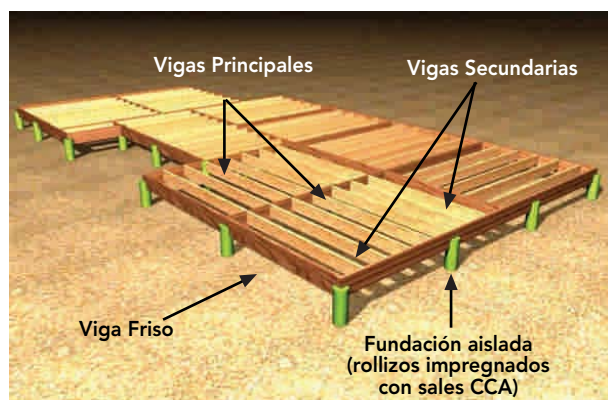
Figura 9 - 1: Ejemplo de un entramado horizontal sobre una fundación aislada, conformado por un conjunto de vigas (principales y secundarias) dispuestas en forma ortogonal.
