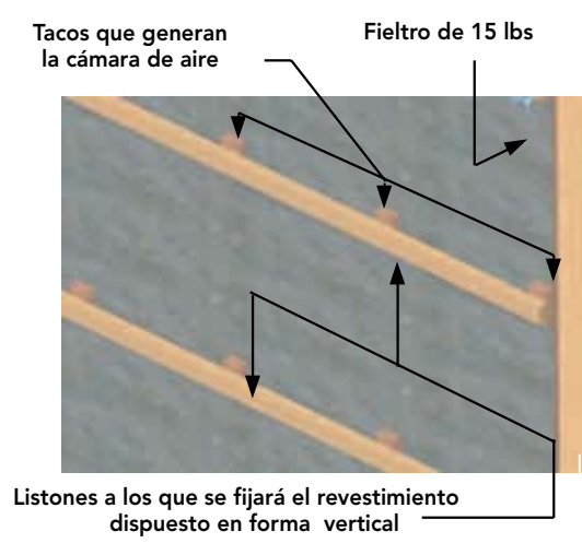
Figura 18 - 40: Preparación del tabique para recibir revestimiento vertical, dejando cámara de aire.
