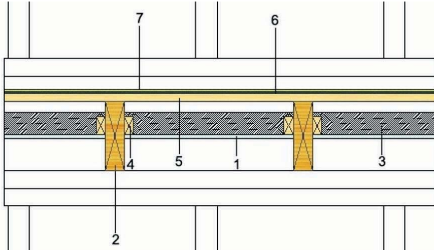
Figura 14 - 68: Representación técnica de la estructura de entepiso, envigado a la vista y piso con revestimiento.
