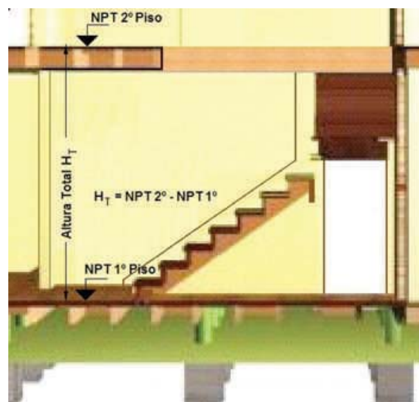
Figura 12 - 19: Altura total de la escalera considerada entre niveles de piso terminado entre ambos pisos de la vivienda.
