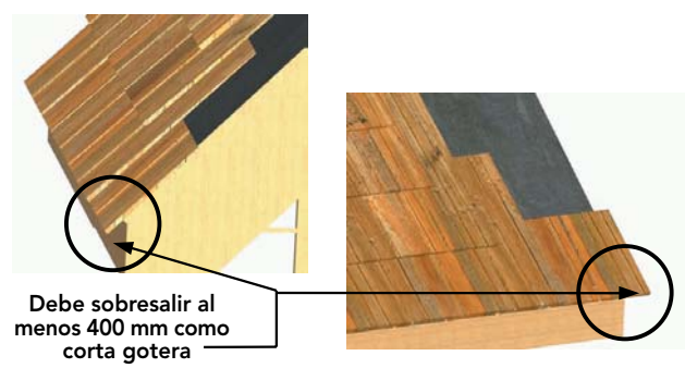
Figura 17-26: Corta gotera dejada por las tejas.
