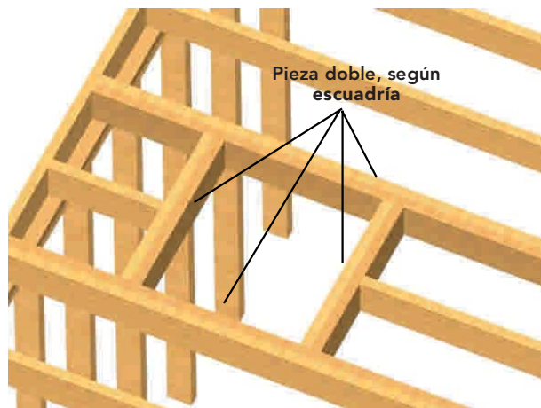
Figura 9 – 53: En el caso de escotillas para la pasada de ductos de chimenea o de ventilación, se soluciona de la misma forma.
