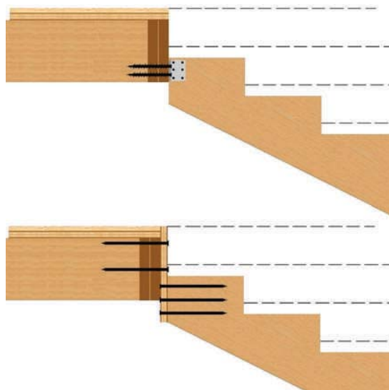
Figura 12 – 28: Anclaje superior de la zanca a la estructura de entrepiso por medio de conectores metálicos o unión clavada con contrachapado.
