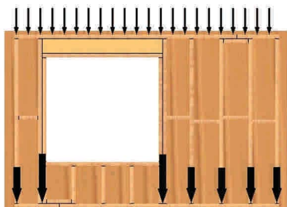
Figura 10 - 7: Esquema de distribución de cargas verticales desde niveles superiores a pie derecho, y de estos a solera inferior.
