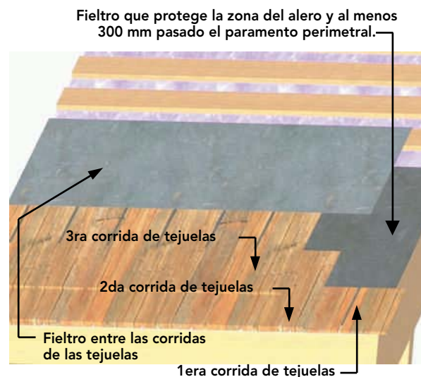
Figura 17-16: Disposición del fieltro en la zona inicial y entre corridas de tejuelas.
