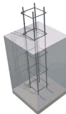
Figura 8 - 11: Pilote de hormigón de sección rectangular, la profundidad del sello de fundación, armaduras y especificaciones, deben ser corroboradas por cálculo estructural.
