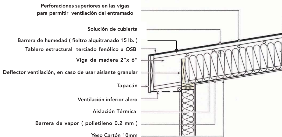
Figura 14 – 22 : Solución de aislación térmica cuando se especifica en el cielo raso y además se debe contar con ventilación entre vigas.
