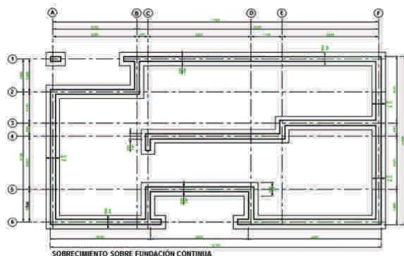
Figura 8 - 27 : Plano de fundación de vivienda prototipo y corte de la solución tipo.
