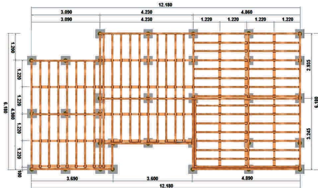
PLANO DE DISPOSICION DE LAS CADENETAS ESTRUCTURALES
