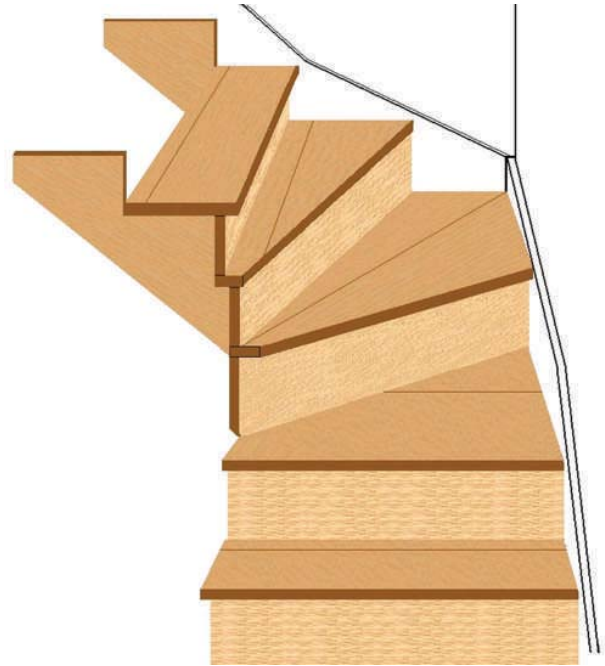
Figura 12 - 33: Ejemplo de huellas encoladas de tipo recto y diagonal en zona de abanico.
