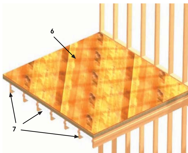
Figura 14-79: Vista general de entrepiso.
