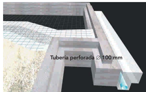
Figura 8 - 1: Instalación de tubo de drenaje en el fondo de zanja que permite evacuar el agua al punto más bajo, inmerso en un relleno de suelo granular.
