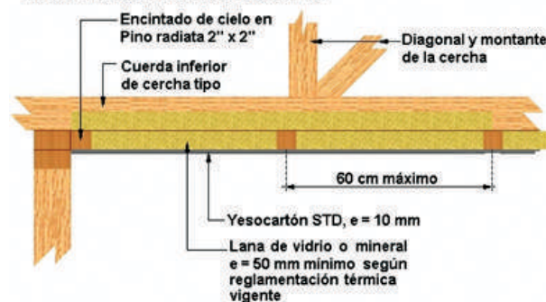
ENTRAMADO DE CIELO RASO F-15
