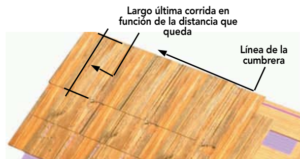
Figura 17-25: Vista de las tejas al llegar a la cumbrera.
