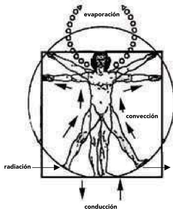
Figura 13 - 10: Intercambio termodinámico del hombre y su hábitat.
