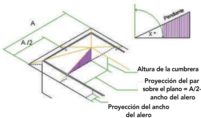
Figura 11-42: Determinar distancias requeridas para formar triángulos.
