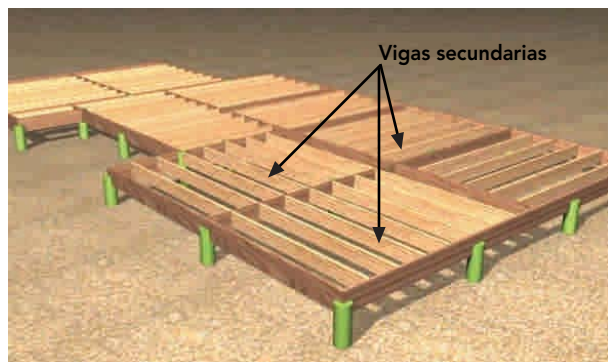
Figura 9 - 27: Entramado de piso dispuesto sobre sistemas de fundaciones aisladas. Conformado por vigas maestras o principales y vigas secundarias que recepcionan los tableros estructurales arriostrantes y base para la solución de piso.
