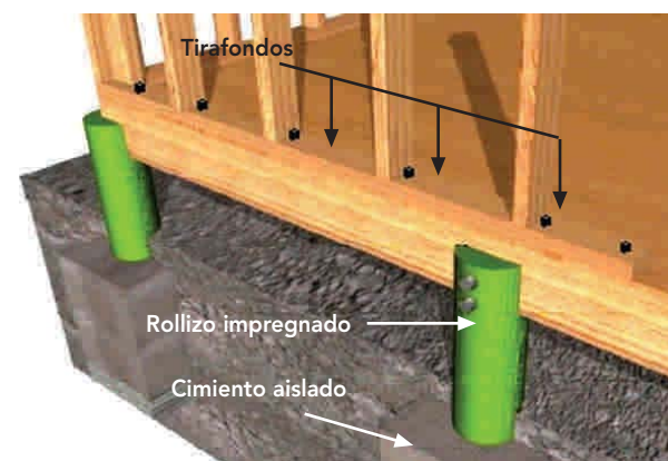
Figura 10 – 41: Ubicación de los tirafondos en la solera inferior del tabique soportante perimetral. En este caso se especifica solera base de montaje.
