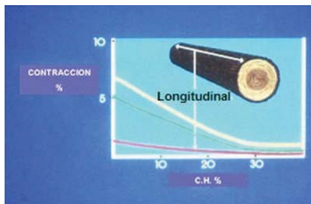
Figura 1 - 27: Gráfico que muestra la proporción de la contracción de la madera en su eje longitudinal.
