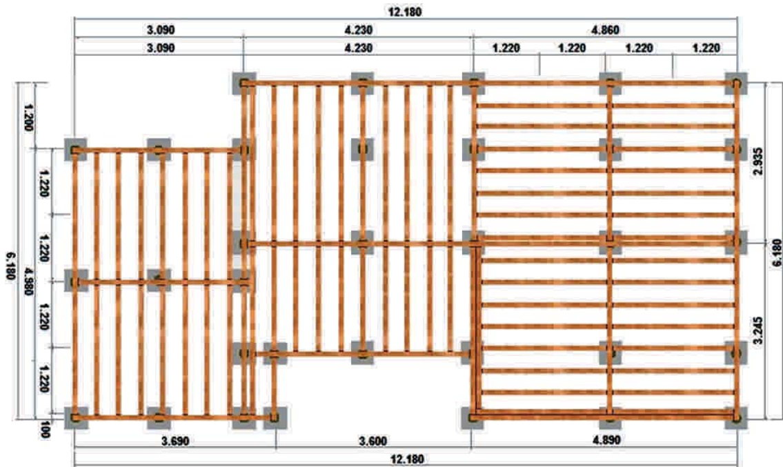
PLANO DE DISPOSICION DE LAS VIGAS SECUNDARIAS
