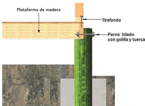
Figura 10 – 42: Anclaje de tabique perimetral soportante con tirafondos a viga principal de la plataforma de madera montada sobre pilotes.
