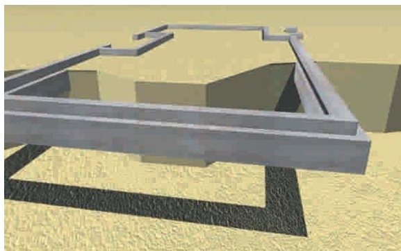
Figura 8 - 17: Vista de un corte del terreno efectuado bajo el cimiento. Altura mínima del cimiento 60 cm.
