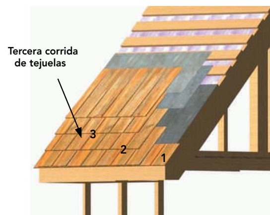
Figura 17-24: Tercera corrida debe dejar zona expuesta de la segunda corrida de tejas.
