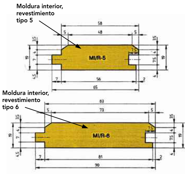
Figura 19-26: Ejemplo de las molduras machihembradas para muros que define la norma NCh2100.
