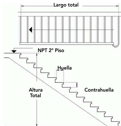
Figura 12 - 2: Planta y elevación de una escalera de tramo recto.
