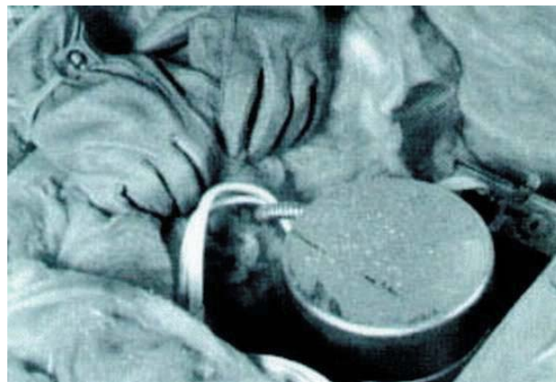
Figura 14 - 21: Se observa el cuidado que se debe tener de no atracar el aislante al foco empotrado en el cielo.
