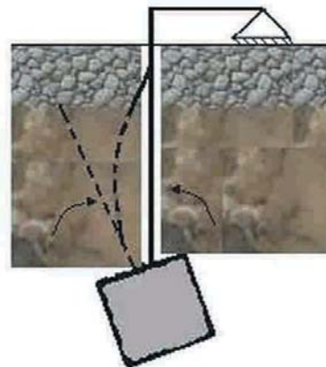
Figura 8 - 4 : Falla de la fundación por volcamiento.
