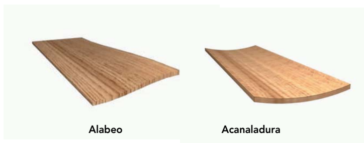
Figura 17 - 6: Deformaciones de la madera producto de variaciones de humedad.
