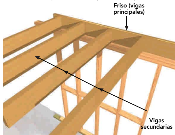
Figura 9 – 3: Piezas de Pino radiata de grado estructural (vigas), de escuadría 2" x 8" o 2" x 10", según cálculo. Vigas que conforman el entramado de entrepiso.
