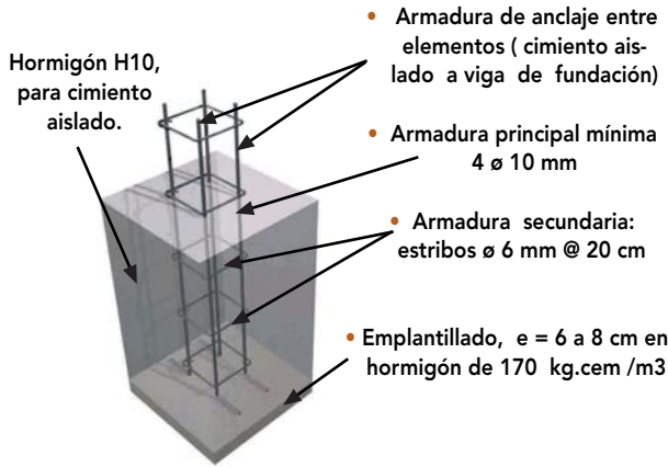
Figura 8 - 39 : Armadura de los cimientos de hormigón.
