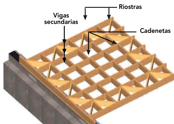
Figura 9 - 9: Riostras materializadas en el perímetro de la plataforma, anclada a fundación continua.
