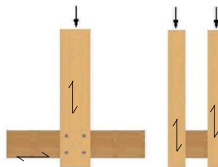
Figura 7- 18 : Carga paralela a la fibra.
