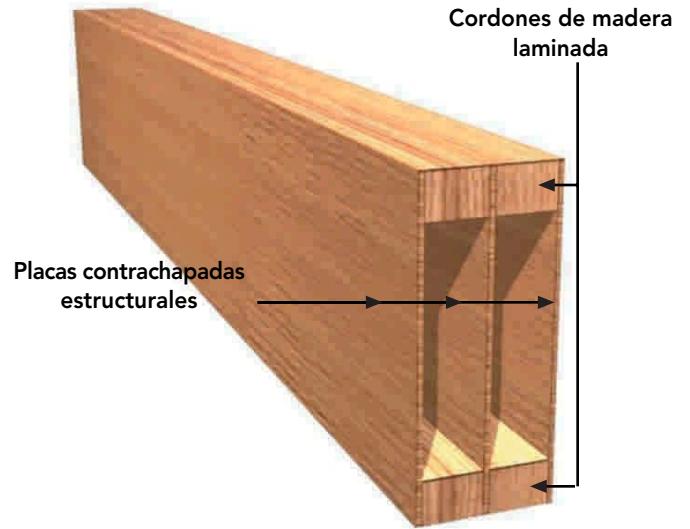
Figura 9 – 65: Para dar mayor resistencia a la viga, se puede intercalar una tercera placa vertical, conformando lo que se llama viga de doble cajón.
