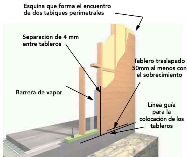
Figura 18 - 39: Colocación de tableros con terminación para revestimiento exterior al inicio de la instalación.
