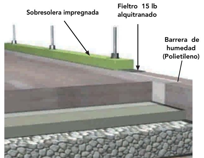
Figura 8 – 59: Instalación de la sobre solera para anclar el tabique perimetral soportante (muro), en la fundación continua con plataforma de hormigón.
