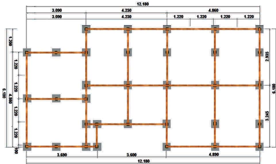
PLANO DE DISPOSICION DE VIGAS PRINCIPALES Y PILOTES
