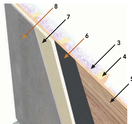
Figura 14-97: Vista de las diferentes pieles que conforman el revestimiento exterior del tabique.
