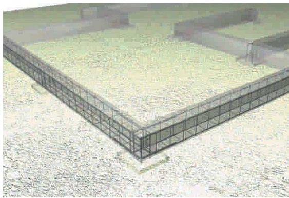
Figura 8 - 13: Viga de fundación que amarra los pilotes de hormigón y receptiona el muro perimetral de la vivienda.
