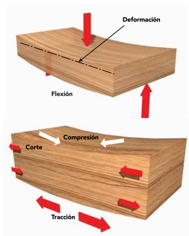
Figura 1 - 31: Esquema de ensayo de la flexión estática.
