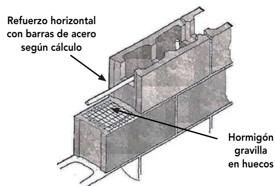
Figura 8 - 33: La instalación de los bloques de hormigón como sobrecimiento debe ceñirse a las especificaciones de cálculo e indicaciones del fabricante.
