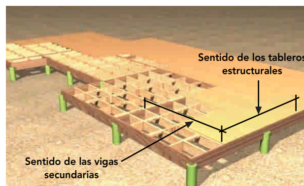
Figura 9 - 14: Instalación de los tableros como riostras y base de plataforma del primer piso en forma alternada y perpendicular a las vigas secundarias.
