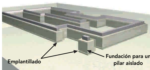
Figura 8 - 9 : Solución de fundación continua con emplantillado de 8 cm de hormigón pobre.
