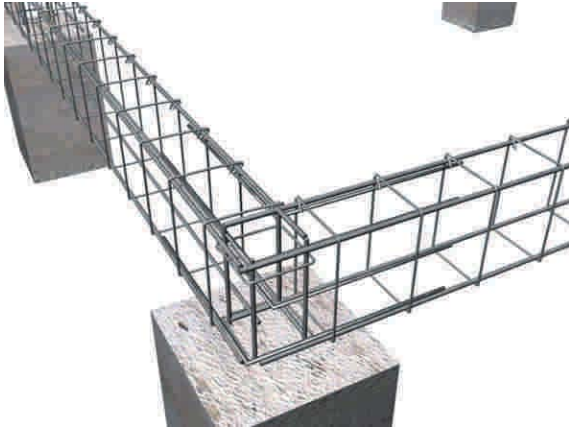
Figura 8 - 12 : Encuentro de esquina de la viga de fundación, donde los fierros del pilote de hormigón pasan a formar parte de la enfierradura de la viga.
