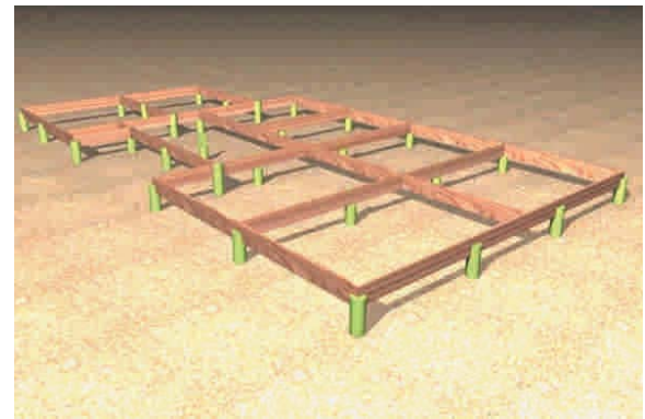
Figura 8 - 15: Vigas friso (viga perimetral) y vigas principales (vigas interiores) que unen las cabezas de los pilotes y transfieren las diferentes cargas de la estructura de la vivienda a la fundación aislada.
