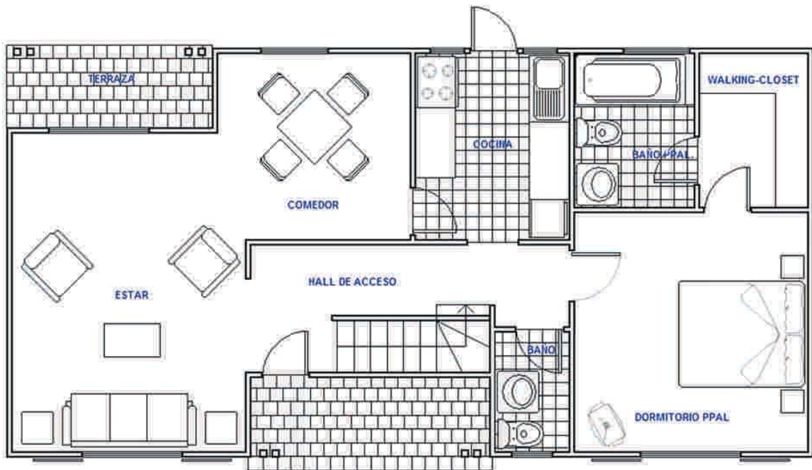
PLANO PLANTA DE ARQUITECTURA PISO 1°
