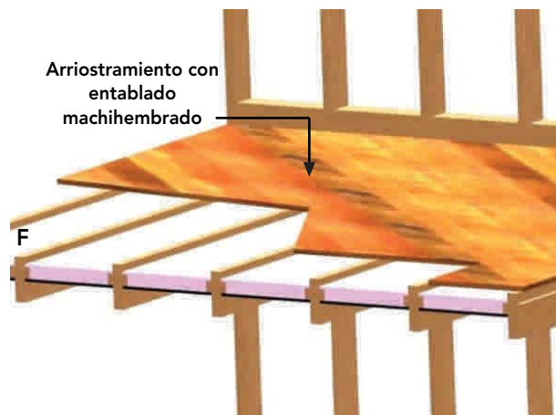
Figura 9 - 11: Ejemplo en el cual se ha especificado como solución de riostra y pavimento terminado a la vista, molduras a 45°, de 114 x 19 mm machihembrada, con aislamiento termo-acústica para la plataforma del entrepiso.
