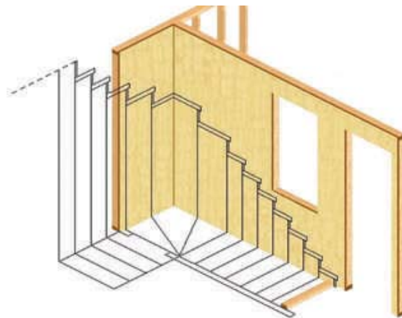
Figura 12 - 27: Trazado de la proyección horizontal y vertical de huellas y contrahuellas de la escalera.
