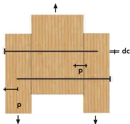
Figura 7- 17 : Resistencia lateral, cizalle múltiple.
