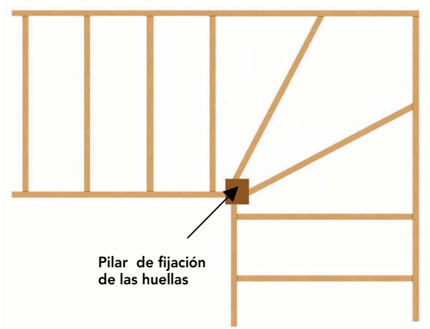
Figura 12 - 34: Piezas de madera fijadas entre zancas para el apoyo y fijación de huellas y contrahuellas.
