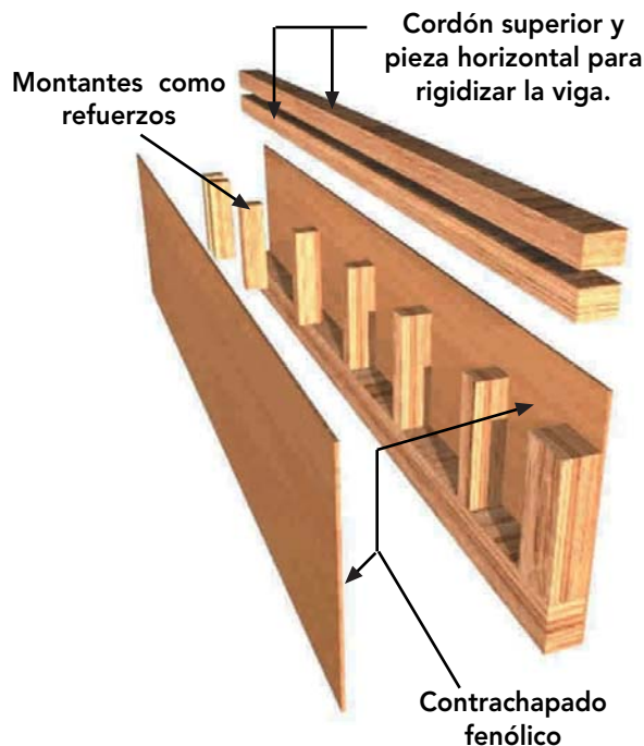
Figura 9 – 67 : En caso que la altura de la viga sea mayor de 1,2 m es necesario armar entre los montantes un entramado horizontal, de forma de rigidizar las tapas laterales.
