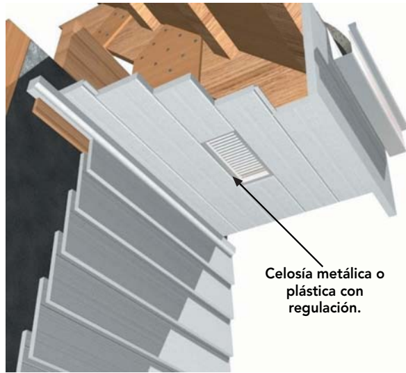
Figura 14 -59: Celosía colocada en el alero cada 50 cm, lo que permite ventilar el entretecho.
