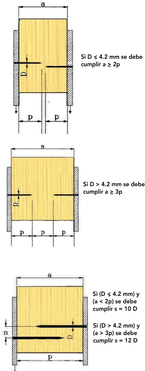
Figura 7- 24 : Uniones de placa de acero y madera con clavado sin disposición alternada.
