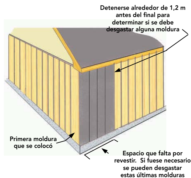
Figura 18 - 36 : Solución para poder obtener una terminación con piezas completas.
