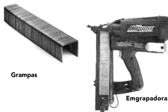
Figura 5 - 29 : Engrapadora neumática.
