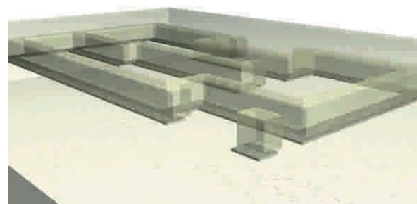
Figura 8 - 19: El sello de excavación debe situarse en un estrato no removido y ripioso, capaz de soportar las tasas previstas.
