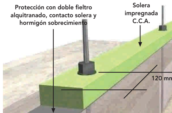
Figura 10 - 36: Detalle constructivo de la distribución de espárragos o barras de anclaje. Espaciamiento de 120 mm entre el último perno y el extremo del término del tabique.
