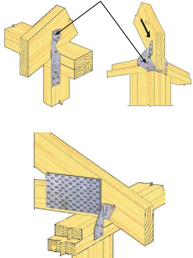
Figura 7- 34: Se muestran algunas alternativas de conectores para los elementos que conforman la techumbre y para su fijación a los entramados verticales.
