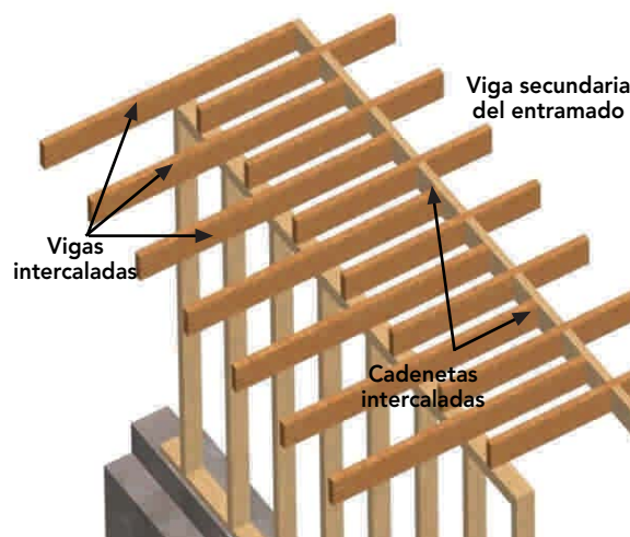
Figura 9 – 50: El voladizo se encuentra en el sentido del entramado de las vigas. En este caso, se intercalaron nuevas vigas entre las existentes, anclándolas a la viga cabezal, dimensiones y largos según cálculo.
