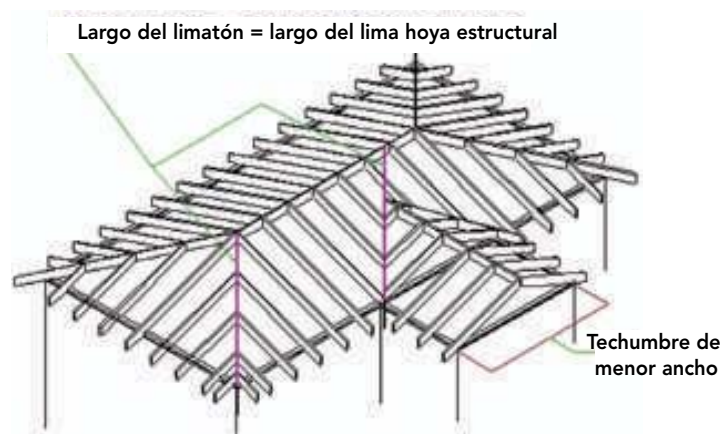
Figura 11-60: Se destacan el limatón y limahoya que tienen el mismo largo, como se observa en la figura.
