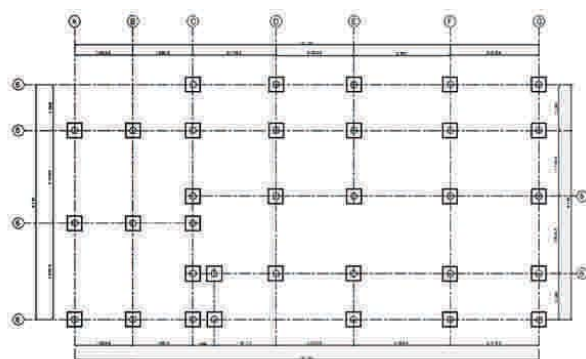
Figura 8 - 44 : Plano de fundación aislada con pilotes de rollizos de madera de diámetro de 8'' a 10'', disposición de los cimientos según los ejes respectivos.
