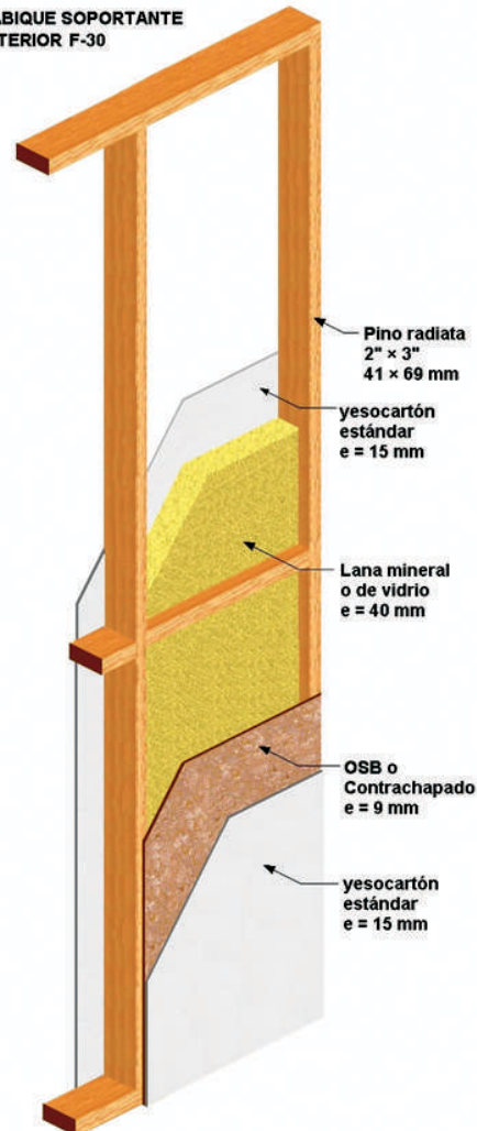
Figura 15 - 27: Solución mínima F-30 para tabiques soportantes interiores. Una o dos filas de transversales cortafuego son opcionales.
