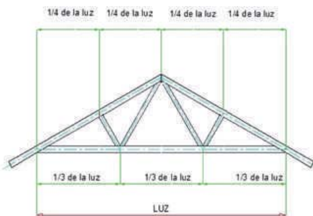
Figura 11-28: Cercha tipo Fink, con los elementos cortados y presentados para su fijación.
