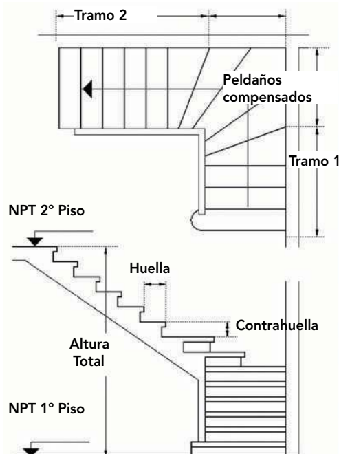
Figura 12 – 5: Planta y elevación tipo de una escalera de dos tramos en ángulo recto con peldaños compensados.
