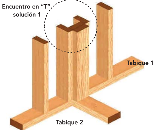
Figura 10 - 59: Solución 1 para encuentro "T" de tope para dos tabiques.
