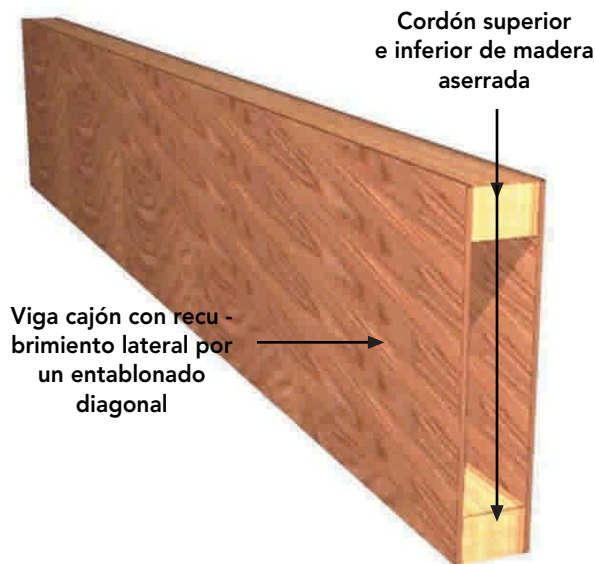
Figura 9 – 64: La altura de una viga cajón varía entre 1/10 a 1/12 de la luz, y la altura de cada uno de los cordones es de aproximadamente 1/7 de la altura total de la viga.
