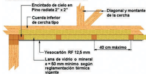
ENTRAMADO DE CIELO RASO F-30
