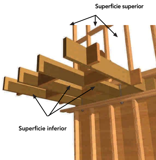
Figura 9 - 28: Vigas secundarias o de entrepiso de escuadrías según cálculo, en este caso, 2" x 8" distanciadas a 400 mm.
