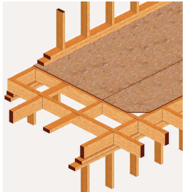
Figura 6 - 12: Elementos horizontales (vigas) apoyados sobre las soleras de amarre de los tabiques del primer piso. Arriostrando el entramado horizontal (plataforma de entresiso) con tableros contrachapado estructural.
