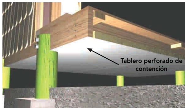
Figura 9-18: Plataforma de primer piso con aislación térmica. La aislación es sujecionada con tablero perforado para mantener ventilada la estructura.
