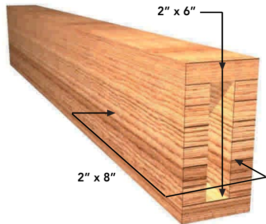
Figura 9 – 66: Viga de cajón laminada que no requiere montantes verticales superiores.
