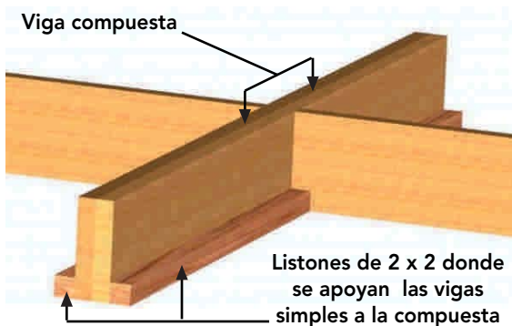
Figura 9 – 59: Solución de unión de viga secundaria a viga compuesta, mediante fijación mecánica y apoyo de pieza aserrada de 2"x 2", según cálculo.
