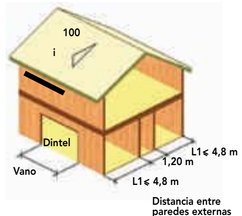
Figura V – 13: Dimensionamiento de dinteles de paredes exteriores de primer nivel en viviendas de dos pisos con entrepiso acústico.
