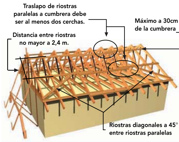
Figura 11-31: Condiciones para las riostras sobre pares.
