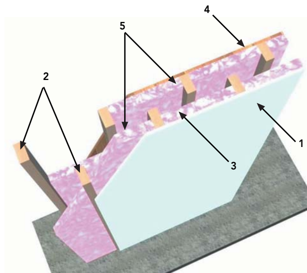
Figura 14 - 89: Disposición de la aislación termo-acústica, entre los doble pie derecho.
