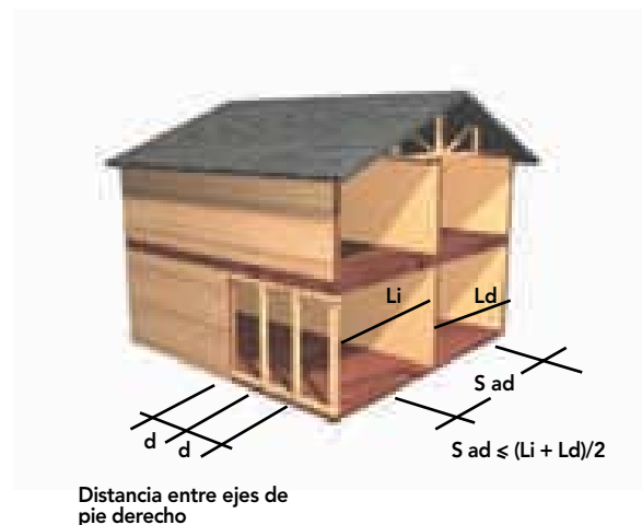
Figura V - 9 : Situación de vivienda de dos pisos, paredes resisten las cargas de piso.
