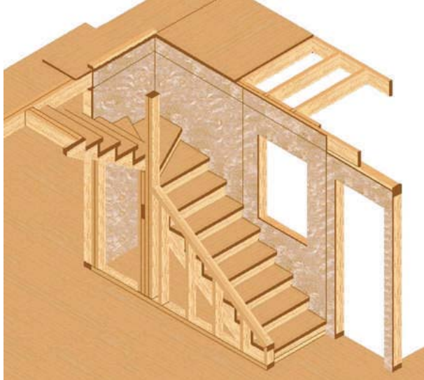
Figura 12 - 35: Se presenta la ubicación del tabique lateral de apoyo y fijación de la estructura de la escalera. Bajo el 2º tramo o tiro, se puede observar un vano de puerta que dará lugar a un clóset bajo la escalera.
