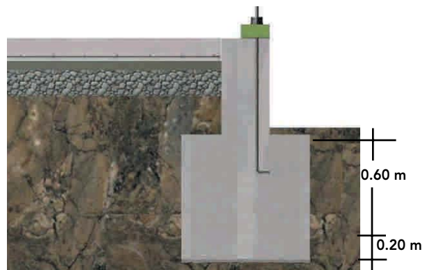
Figura 8 - 20: Profundidad mínima del cimiento con penetración mínima.
