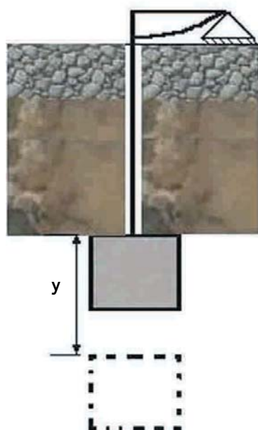
Figura 8 - 3 : Falla de la fundación por descenso.
