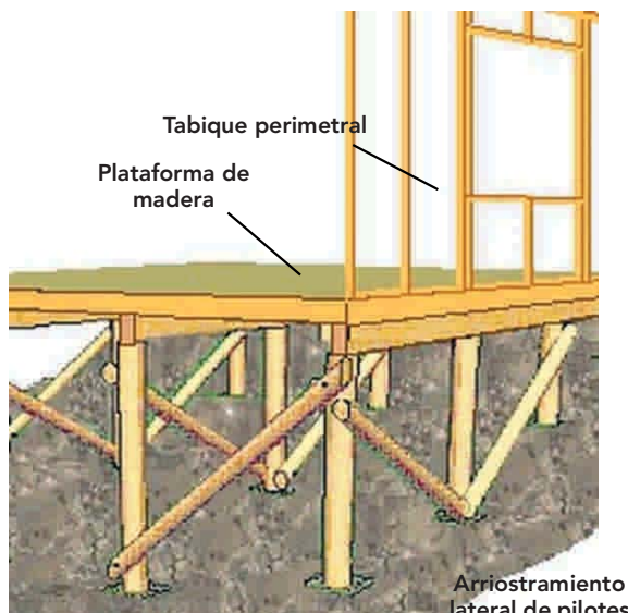
Figura 8 - 49 : Arriostamiento de pilotes según cálculo estructural.
