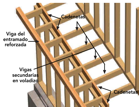
Figura 9 – 51: El entramado se encuentra en sentido perpendicular al voladizo. Envigado secundario de igual escuadría se ancla a la penúltima viga, la que se duplicare forzando dimensiones y largos según cálculo.
