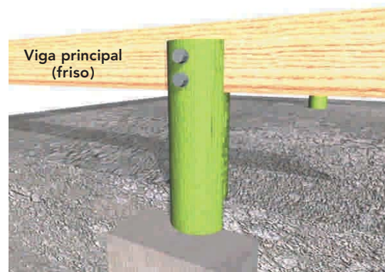
Figura 8 - 50: Fijación de la viga principal a los pilotes mediante pernos, golillas y tuercas
