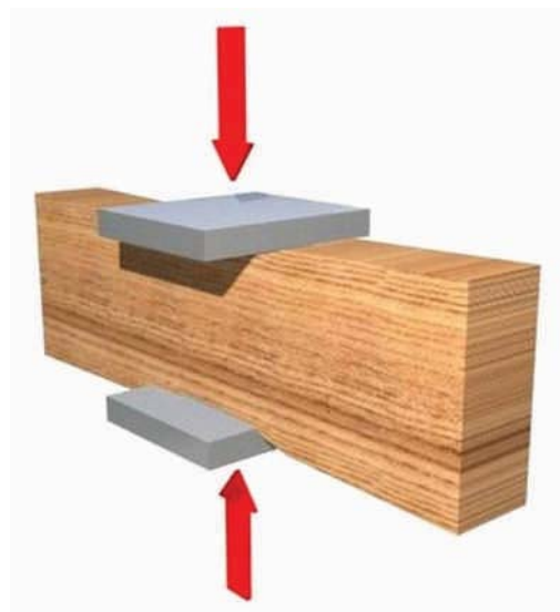
Figura 1 - 30: Esquema de ensayo de compresión normal a las fibras.
