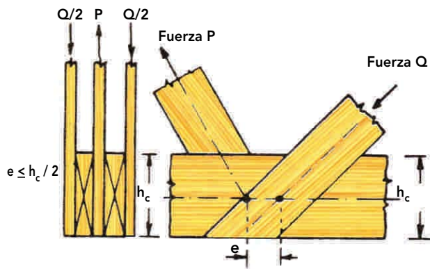
Figura 7- 11 : Uniones de barras excéntricas.
