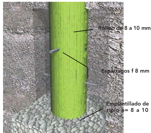
Figura 8 - 45 : Emplantillado de ripio para los pilotes de madera impregnados, espárragos para la adherencia con el hormigón.
