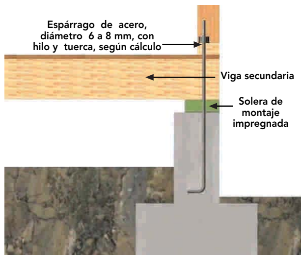
Figura 9 - 22: Viga perimetral del entramado de piso, se fija a solera de montaje en la fundación continua mediante ángulos metálicos. El tabique soportante perimetral es anclado a la fundación mediante la colocación de espárrago con hilo y tuerca (diámetro de 6 a 8 mm), aproximadamente cada 0.80 m, uniendo la solera inferior del tabique con la solera de montaje a través del espárrago anclado al sobrecimiento.
