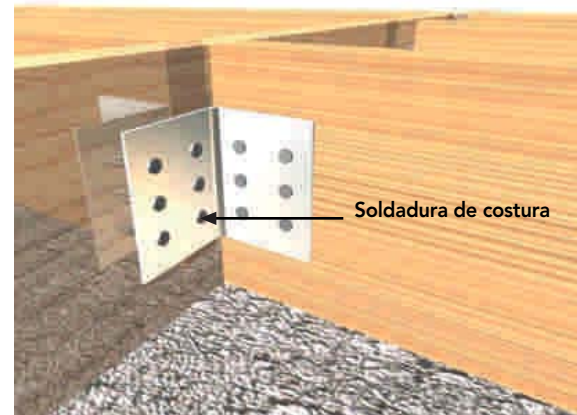
Figura 9 – 46: Conector fabricado con pletina de espesor 3 a 4 mm conformado por dos piezas que se unen mediante soldadura de costura, como se puede apreciar en la figura.
