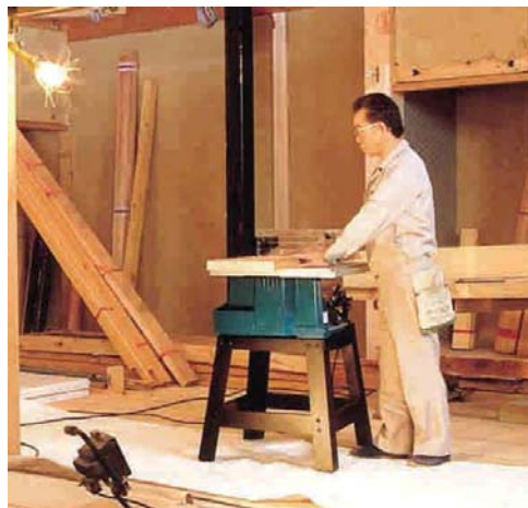
Figura 5 - 46 : Sierra circular para cortes rectos.
