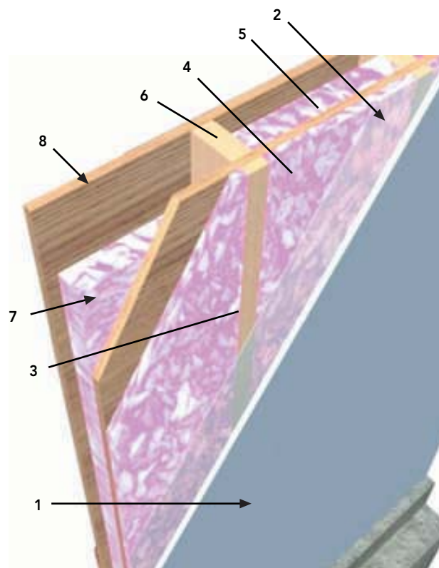
Figura 14-93: Vista interior del tabique perimetral.
