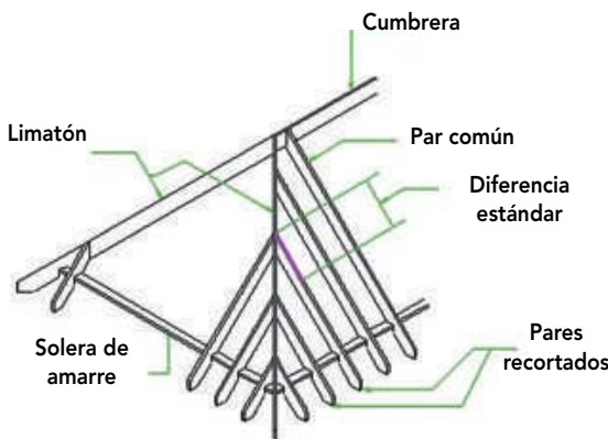
Figura 11-50: Se destaca una longitud llamada "diferencia estándar" para determinar largo de los pares recortados.
