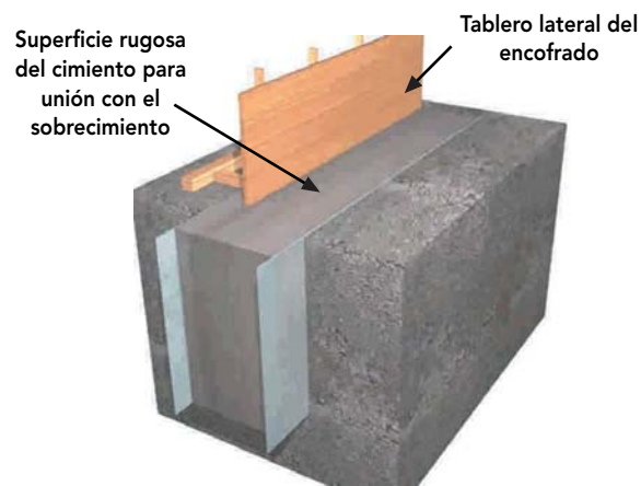
Figura 8-29: Instalación inicial del encofrado para la materialización del sobrecimiento.
