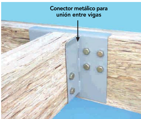
Figura 9 – 44: Conector fabricado con pletina de 3 a 4 mm conformado por dos piezas, las cuales se unen mediante soldadura de costura, como se puede apreciar en la figura. Las vigas se fijan con tirafondos de diámetros y largos según cálculo.
