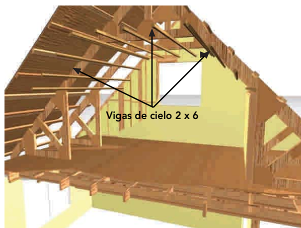
Figura 9 – 32: Vigas que conforman el entramado de cielo bajo cerchas habitables. En este caso, escuadrías de 2 x 6, que recibirán el encintado de 2 x 2 y placas de yeso o entablado como solución de cielo.
