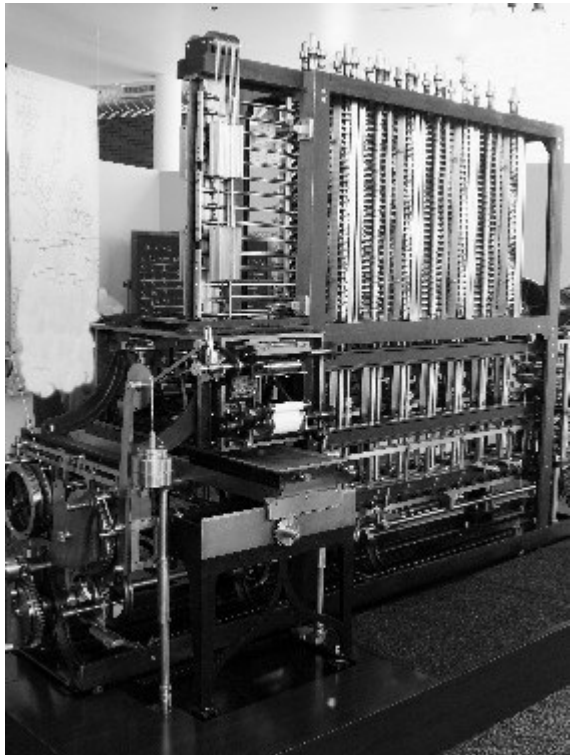
Réplica de la máquina diferencial.
