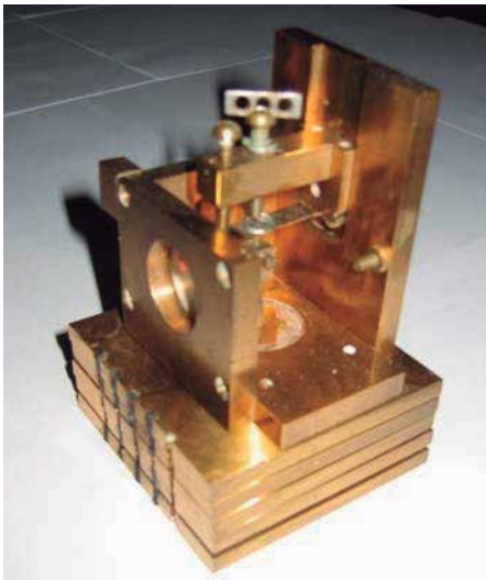
Figura 6.1. Primer Microscopio de Efecto Túnel desarrollado en 1987.
