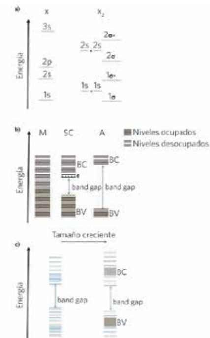
Figura 3.1: a) Niveles de energía cuantizados (orbitales) para átomo X y molécula diatómica X 2 ; b) Niveles de energía y estructura de bandas en sólidos (M: conductor, SC: semiconductor y A: aislante) y c) Niveles de energía discretos y estructura de bandas para nanomateriales.
