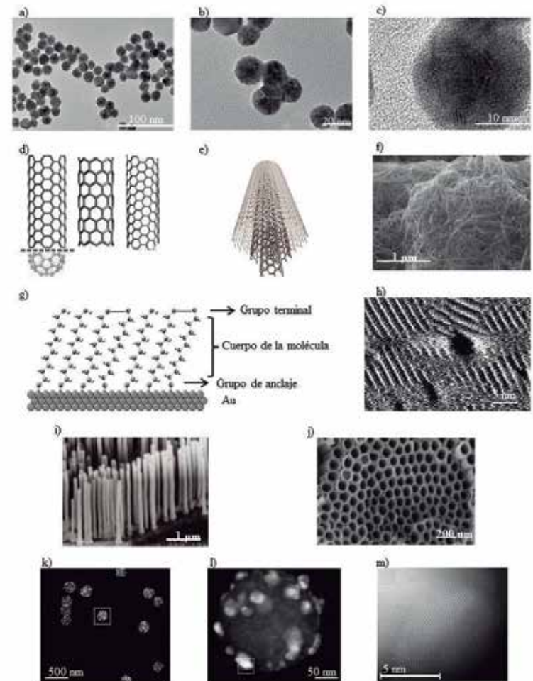
Figura 3.3 Nanomateriales: a-c) Imágenes TEM de Nanopartículas de Au3; d) Estructura de Nanotubos de pared simple, e) Estructura de Nanotubo de pared múltiple, f) Imágenes SEM de Nanotubos de C4; g) Estructura de monocapa de ditiolos sobre Au, h) Imagen STM de monocapa de 1,8 octanoditiol sobre Au; i) Micrografía SEM de Nanoalambres de ZnO; j) Micrografía SEM de TiO nanoporoso8; k-m) Micropartículas de SiO2
