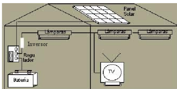
Figura 2. Esquema simple de un sistema fotovoltaico
