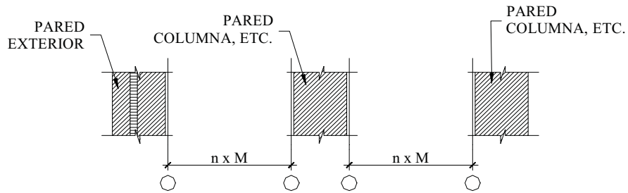
GRÁFICO 6: EJEMPLO DE PLANOS MODULARES EN POSICION LIMITE
