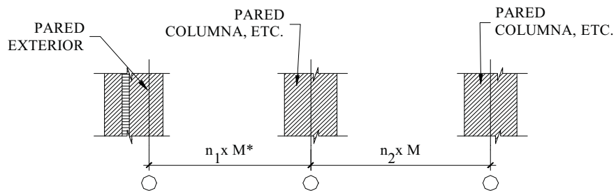
EN EL CASO DE ELEMENTOS ASIMETRICOS (POR EJEMPLO PAREDES EXTERIORES), EL PLANO MODULAR PUEDE NO COINCIDIR CON EL PLANO CENTRAL GRAFICO 7: EJEMPLO DE PLANOS MODULARES EN POSICION AXIAL
