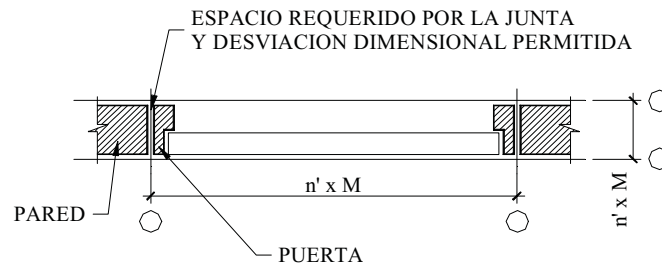
GRAFICO 5: EJEMPLO DE UN COMPONENTE DE EDIFICIO LOCALIZADO EN UN ESPACIO MODULAR ASIGNADO
