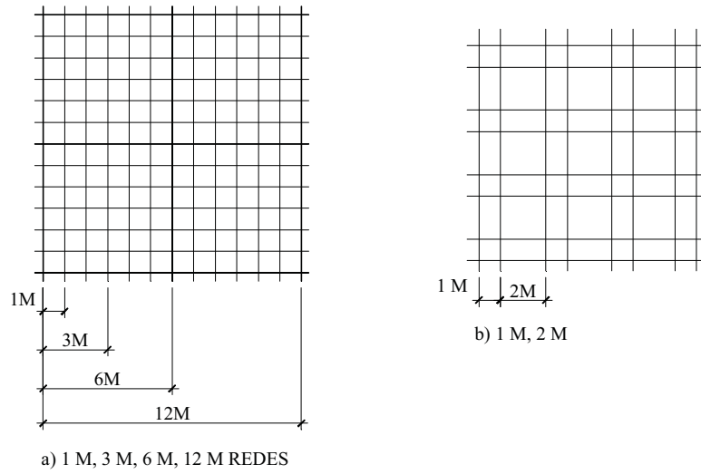
GRAFICO 2: EJEMPLO DE REDES MODULARES SUPERPUESTAS
