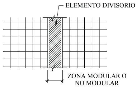
GRAFICO 3: INTERRUPCION DE REDES MODULARES
