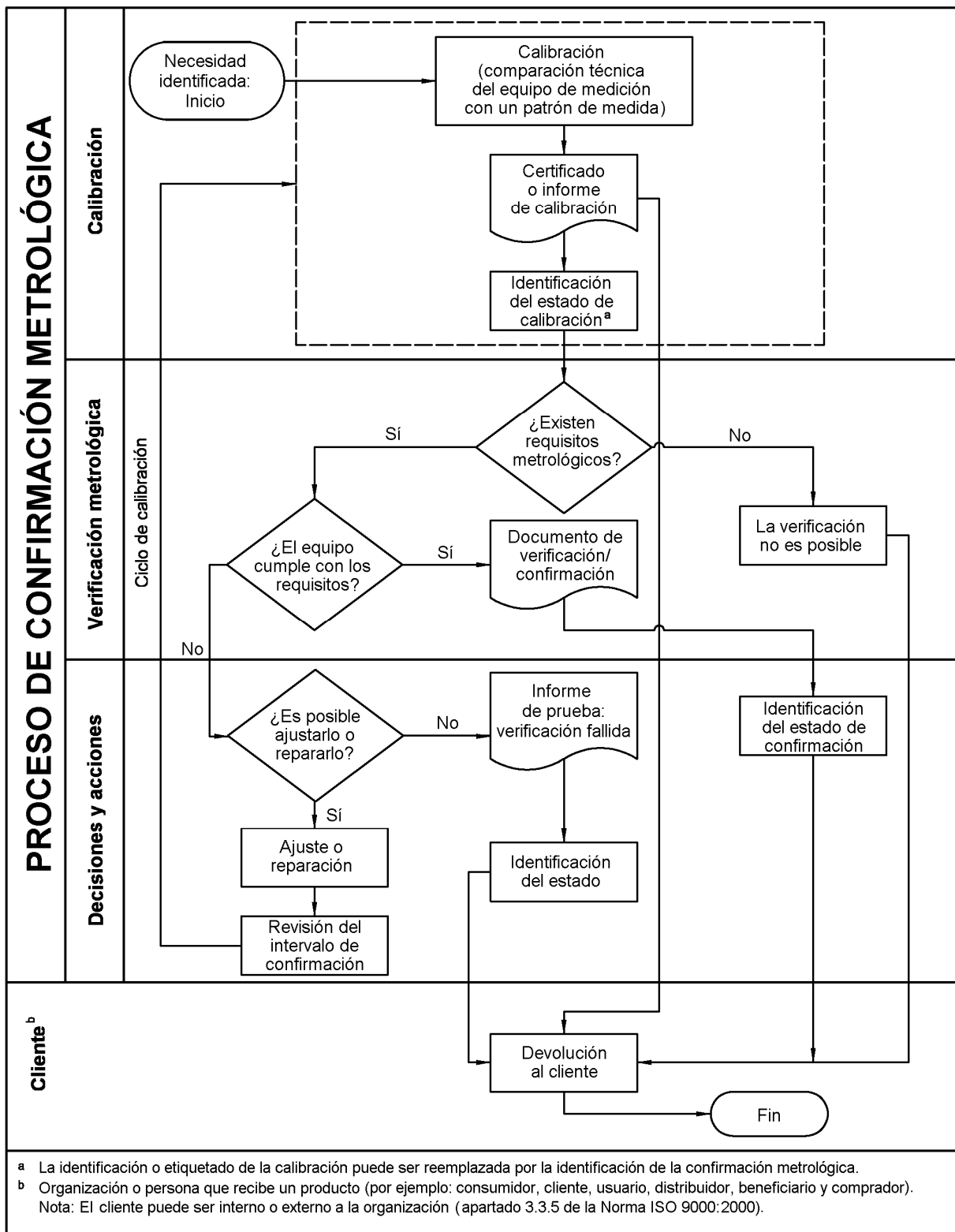
Figura 2 – Proceso de confirmación metrológica del equipo de medición
