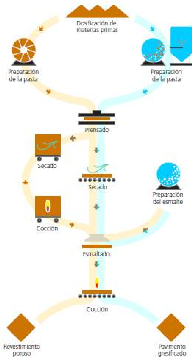
Ilustración 12 Esquema de fabricación de azulejos y gres esmaltado
