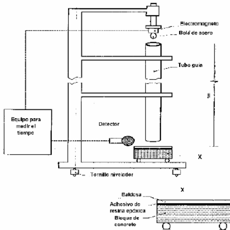
Ilustración 78 Aparato para descargar la bola
