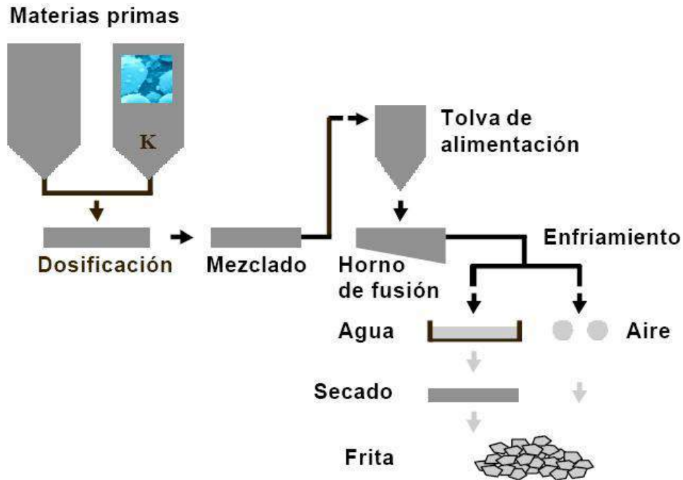
Ilustración 34 Esquema del proceso de fabricación de fritas
