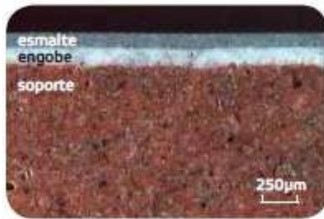
Ilustración 36 Baldosa engobada y esmaltada
