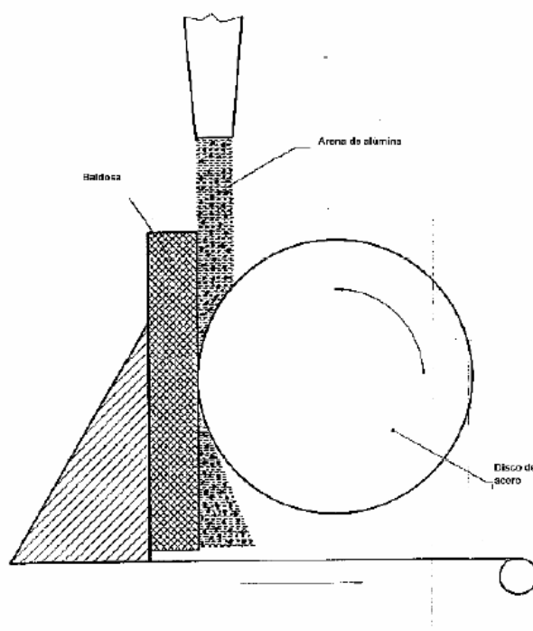
Ilustración 69 Esquema del equipo de abrasión profunda
