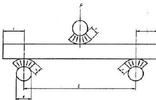
Ilustración 68 Sección de aparato de módulo de rotura
