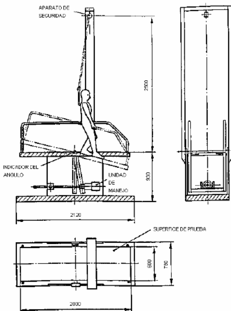
Ilustración 76 Método C plataforma inclinada
