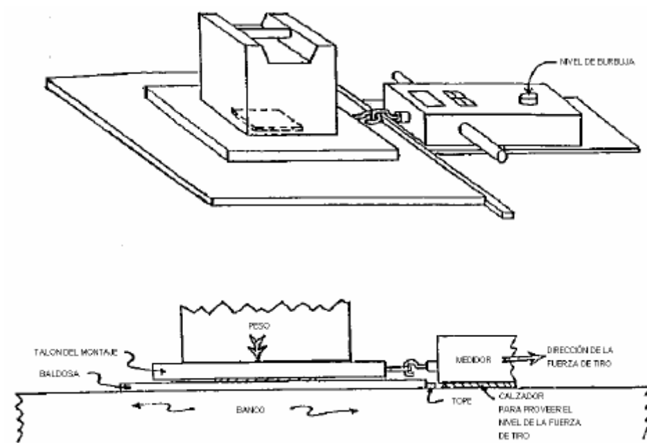
Ilustración 75 Método B deslizador estático
