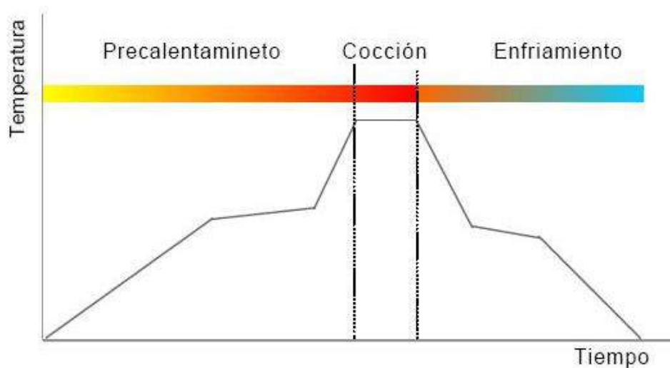
Ilustración 56 Esquema del proceso de cocción
