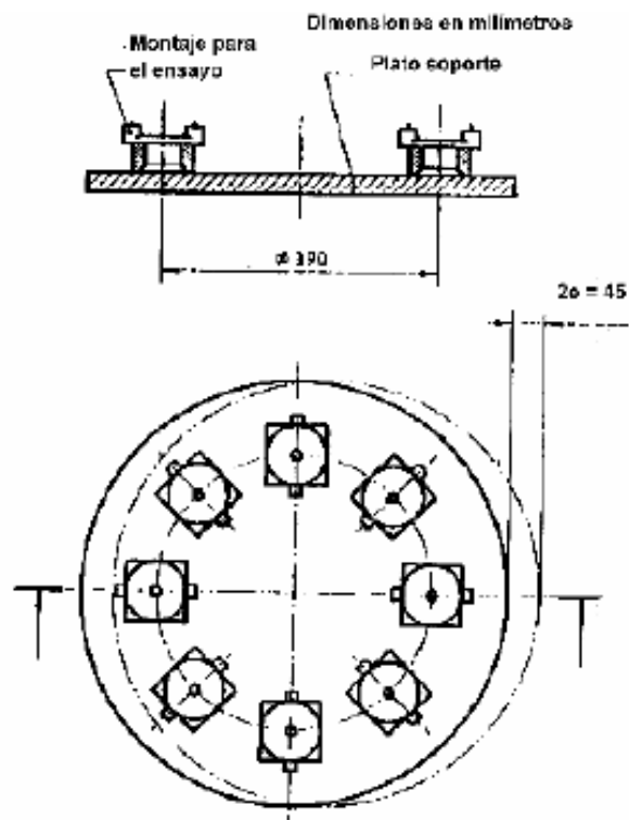
Ilustración 70 Equipo de abrasión superficial
