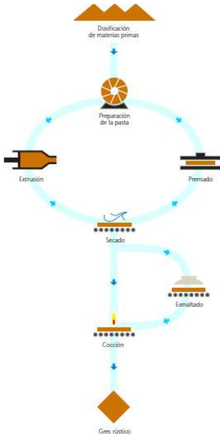
Ilustración 14 Esquema del proceso de fabricación del gres rústico
