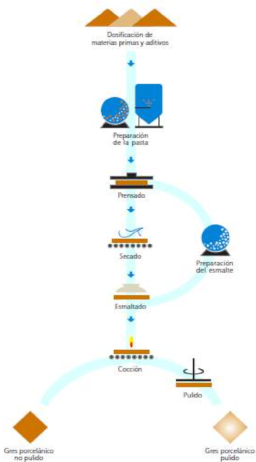
Ilustración 13 Esquema de fabricación del gres porcelánico
