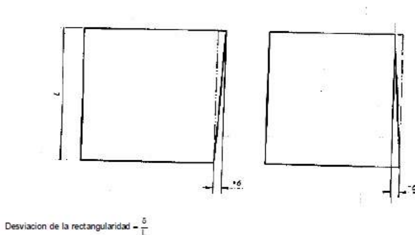
Ilustración 63 Desviación de la rectangularidad
