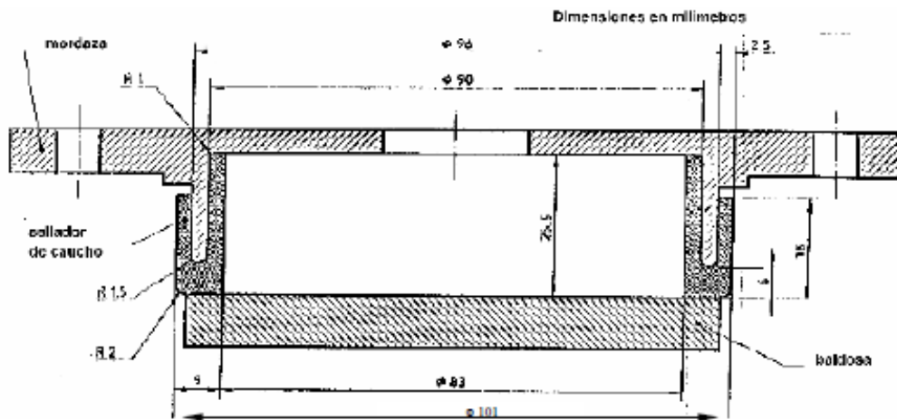
Ilustración 71 Corte equipo de abrasión superficial
