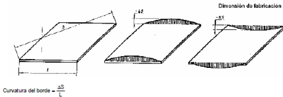
Ilustración 65 Curvatura del borde
