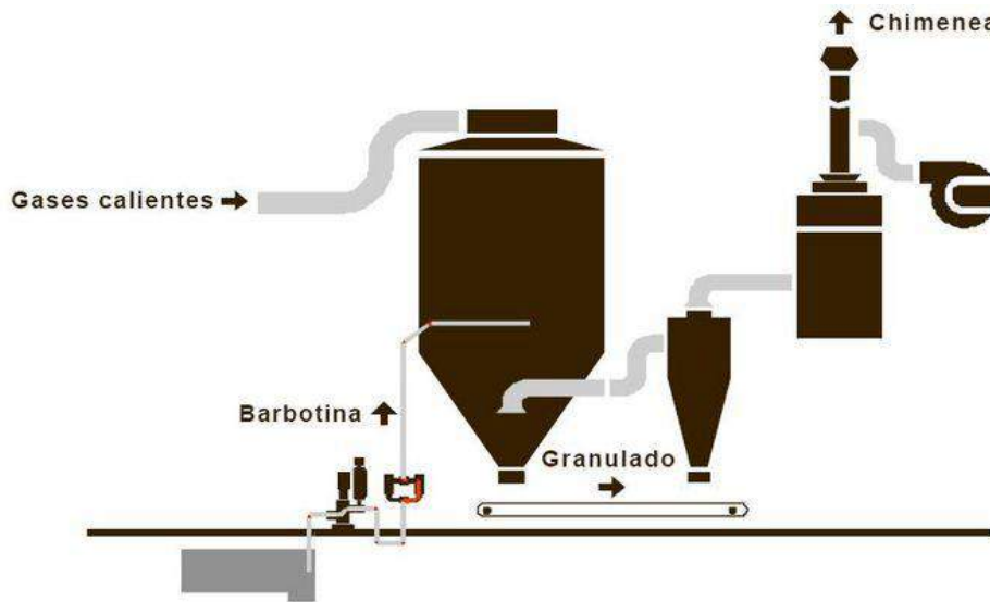
Ilustración 19 Esquema de secado por atomización
