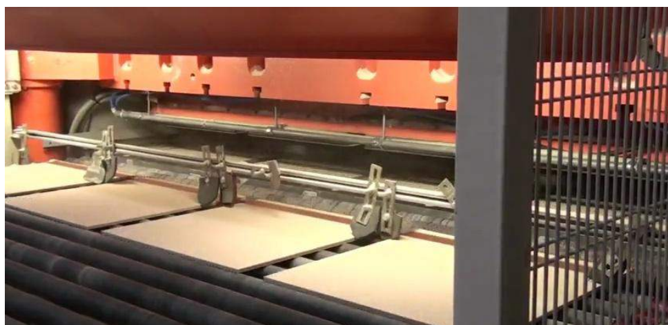
Ilustración 26 Salida de las baldosas conformadas
