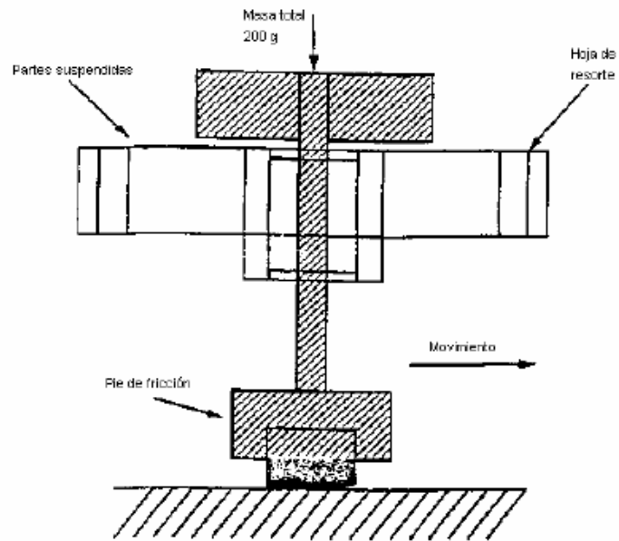
Ilustración 73 Método A2 deslizador dinámico
