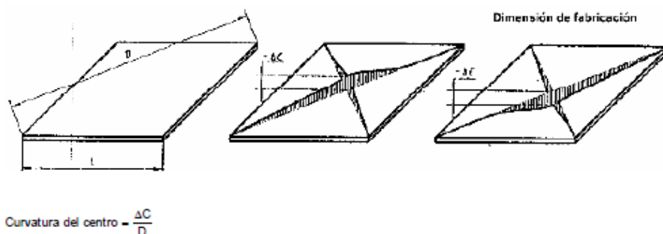
Ilustración 64 Curvatura del centro
